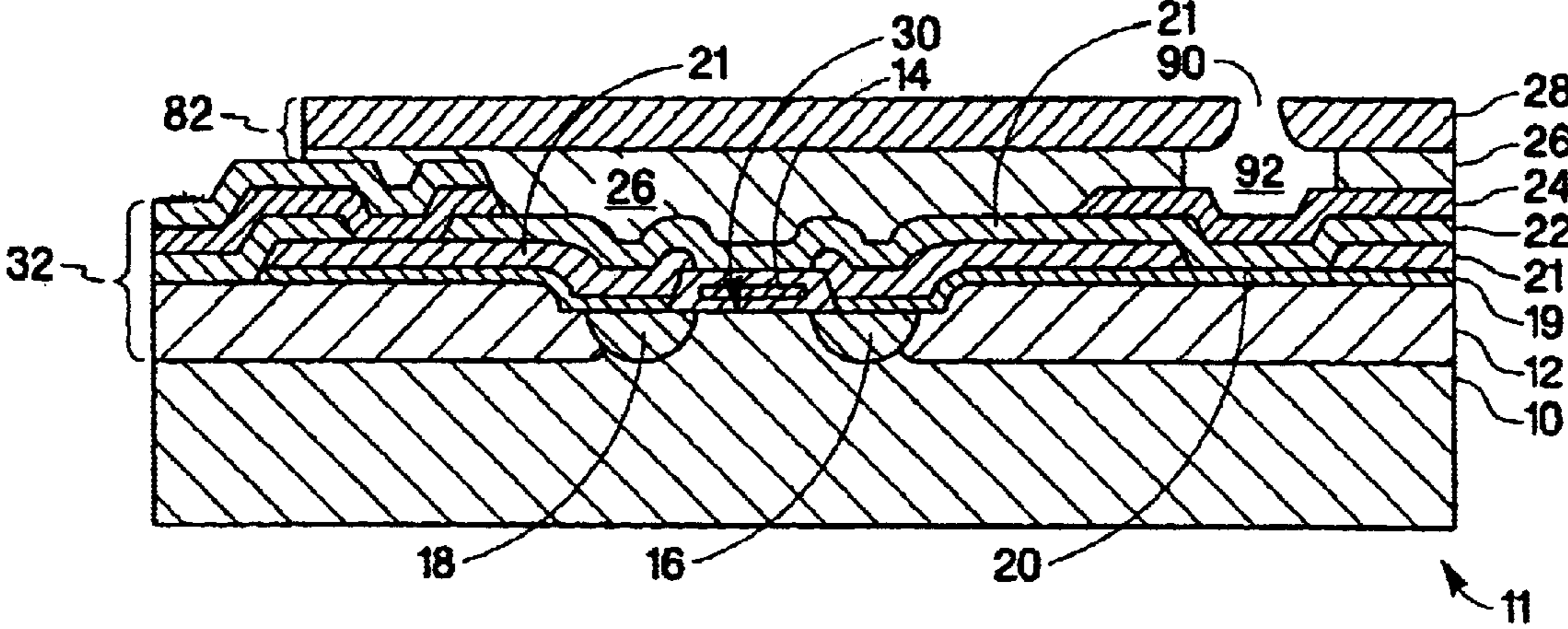
Fig. 1 -- PRIOR ART --
