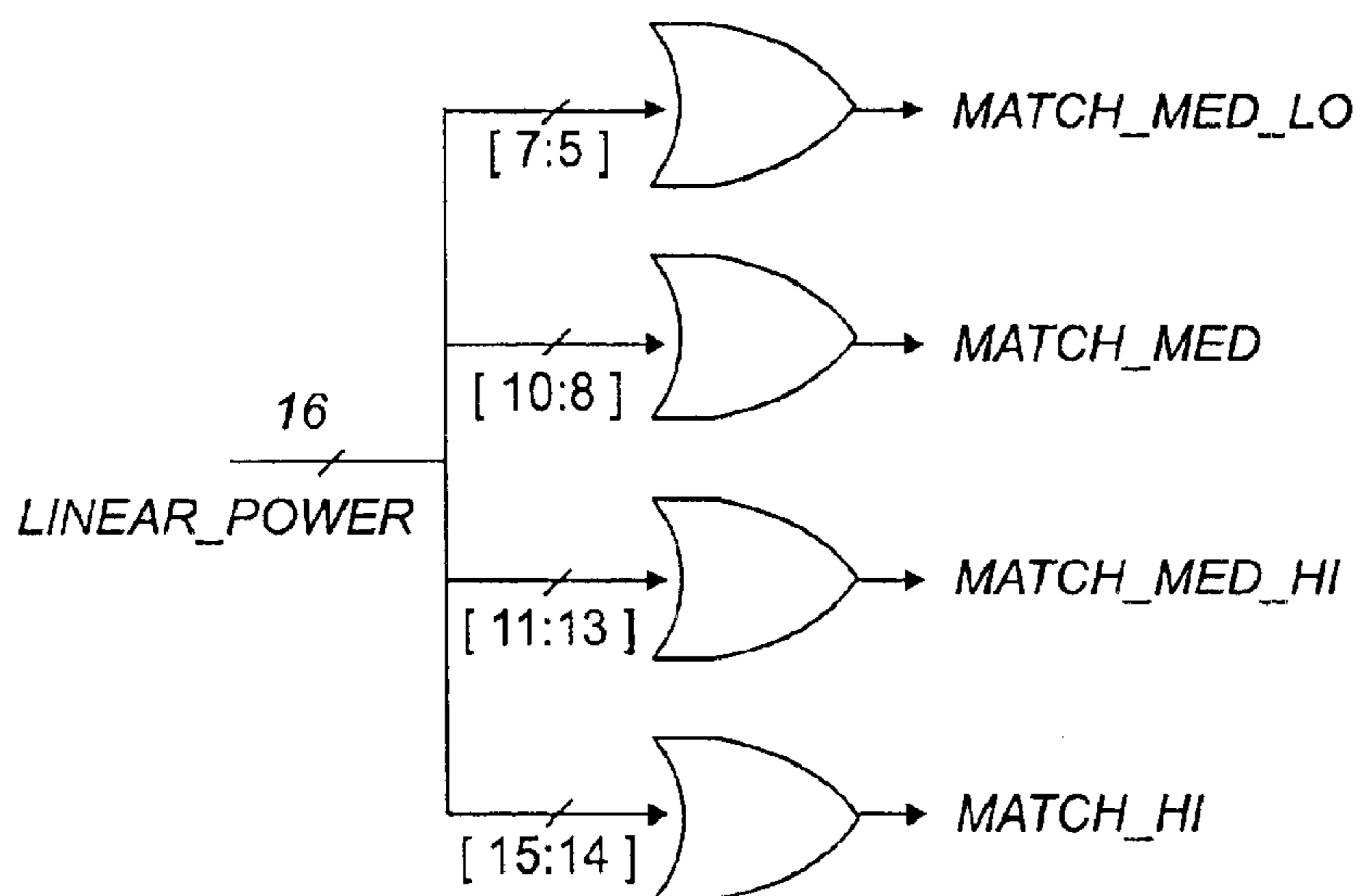
FIG. 5A
