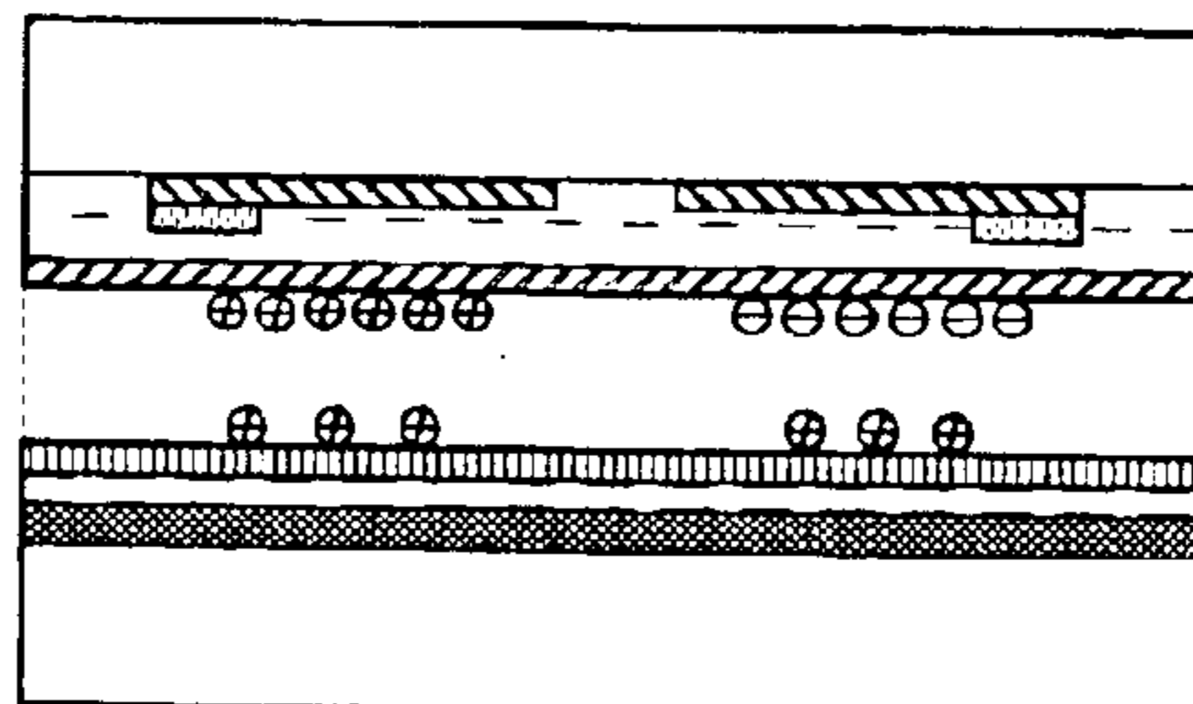
FIG. 20E (PRIOR ART)
