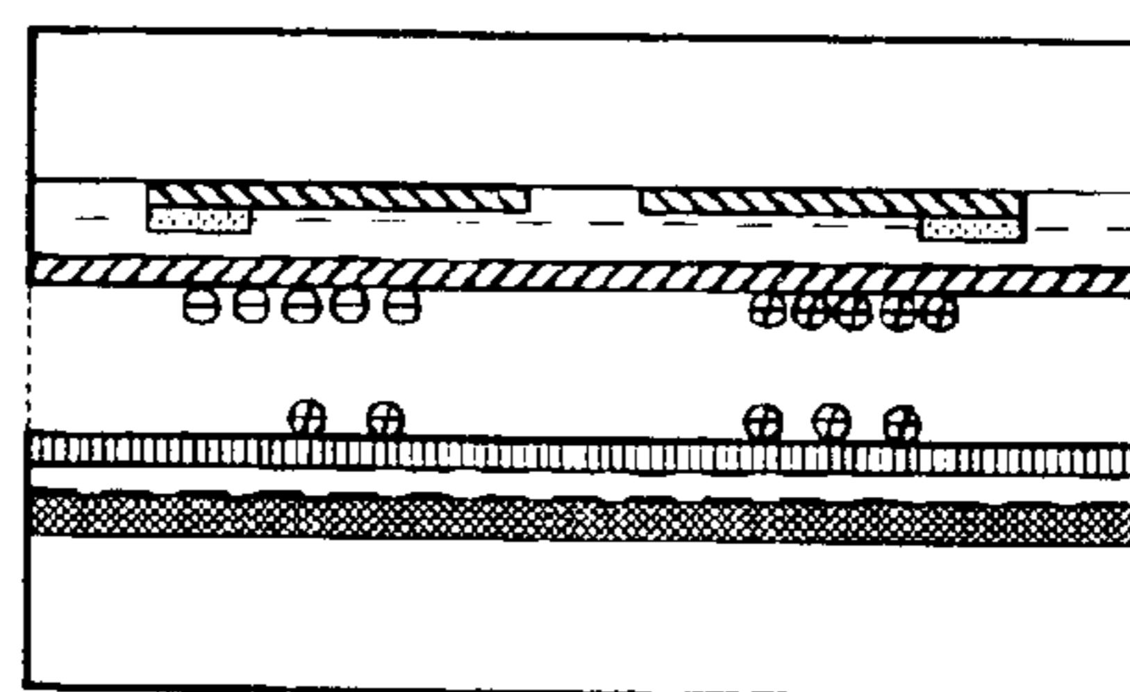
FIG. 19E (PRIOR ART)
