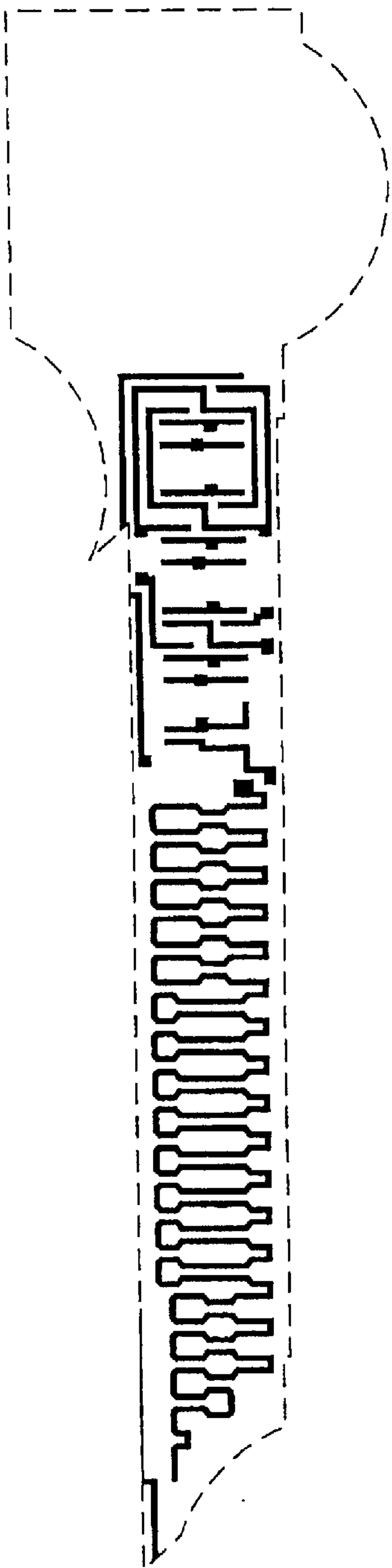
Poly mask
