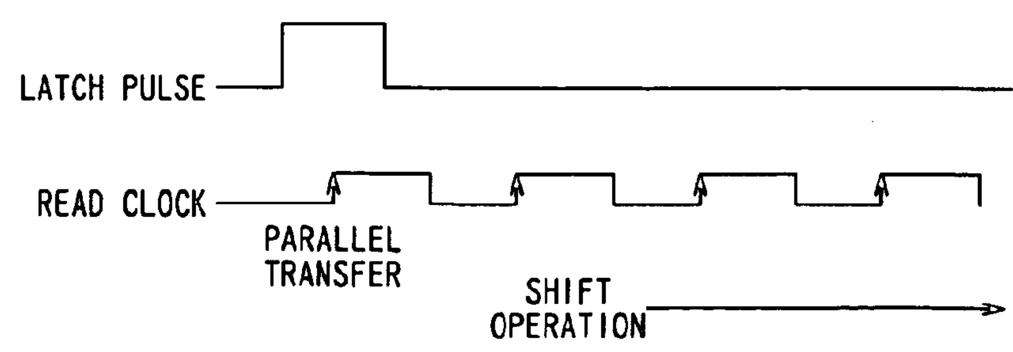
Fig. 6 D
