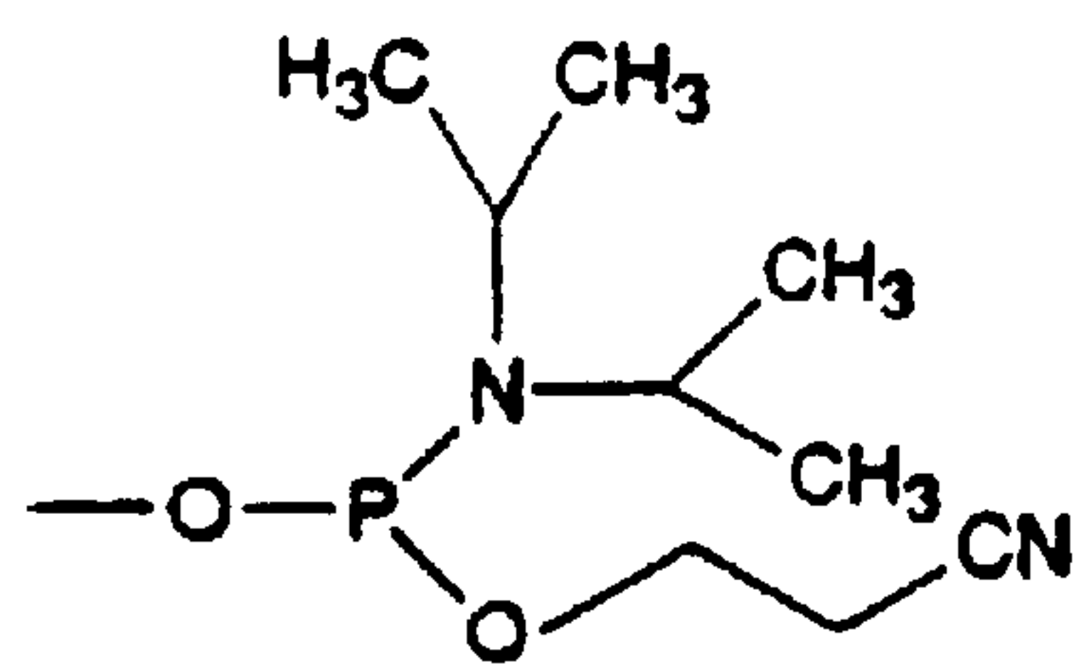
N,N-diisopropylamino-β-cyanoethoxyphosphine
