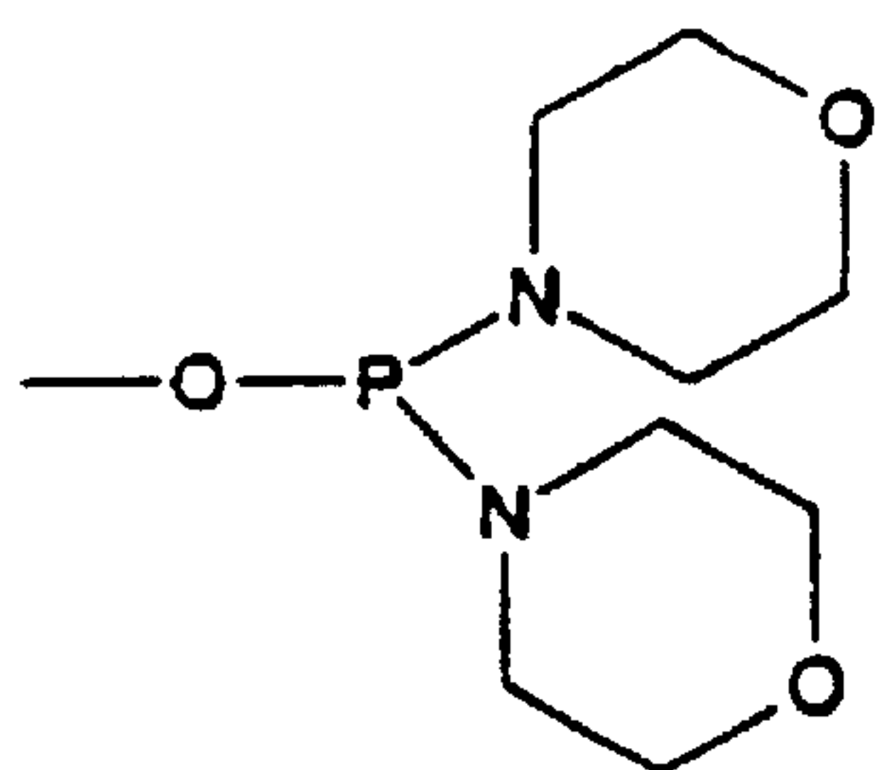
Bis morpholino-phosphine
