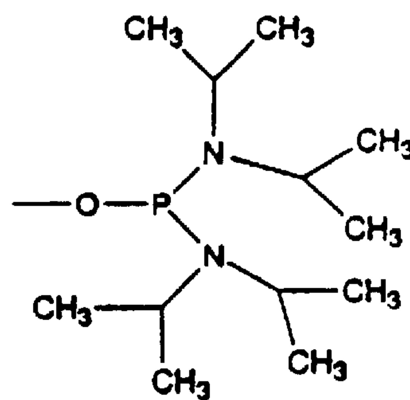
Bis(N,N-diisopropylamino)- phosphine
