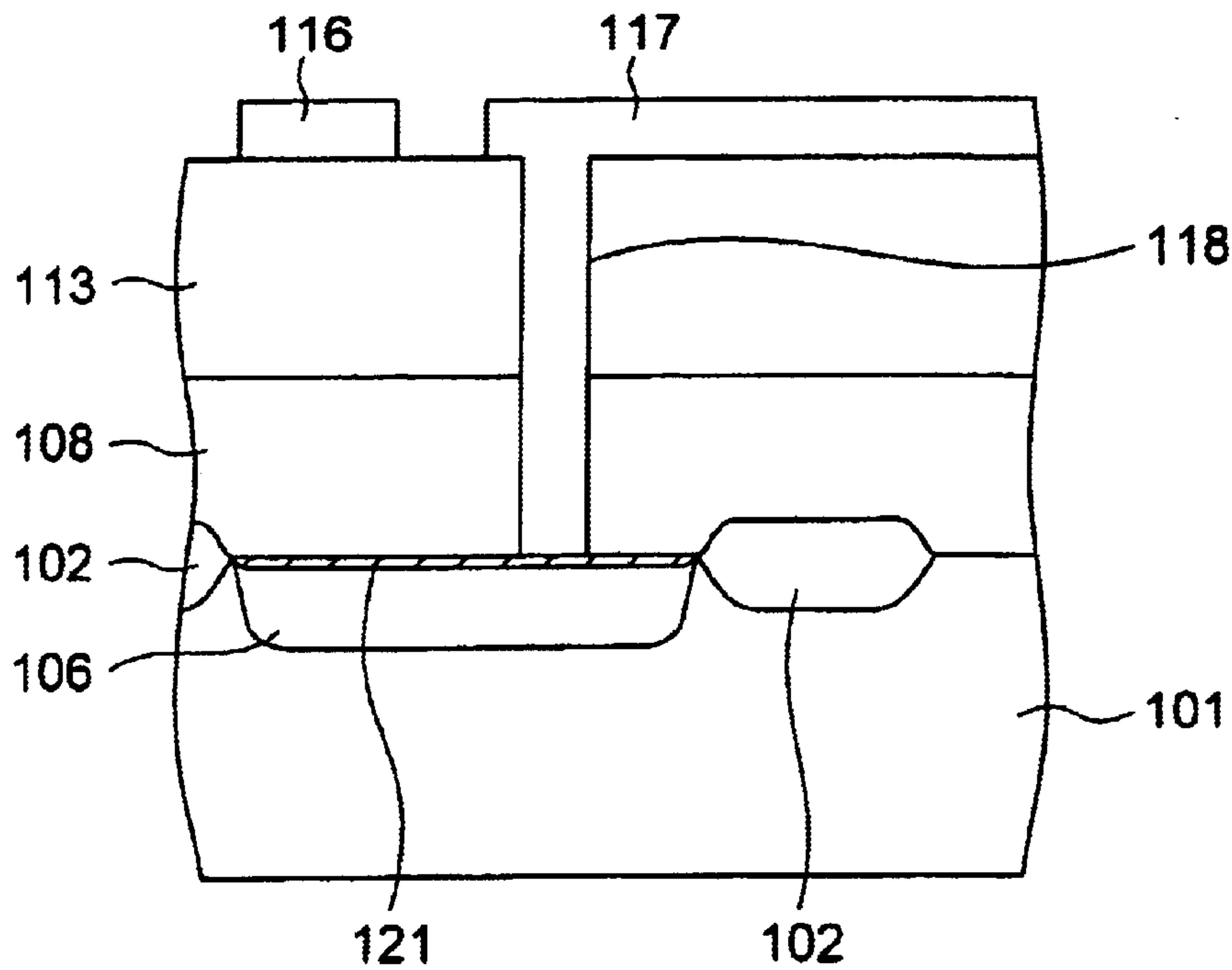
FIG. 2B b-b' SECTION
