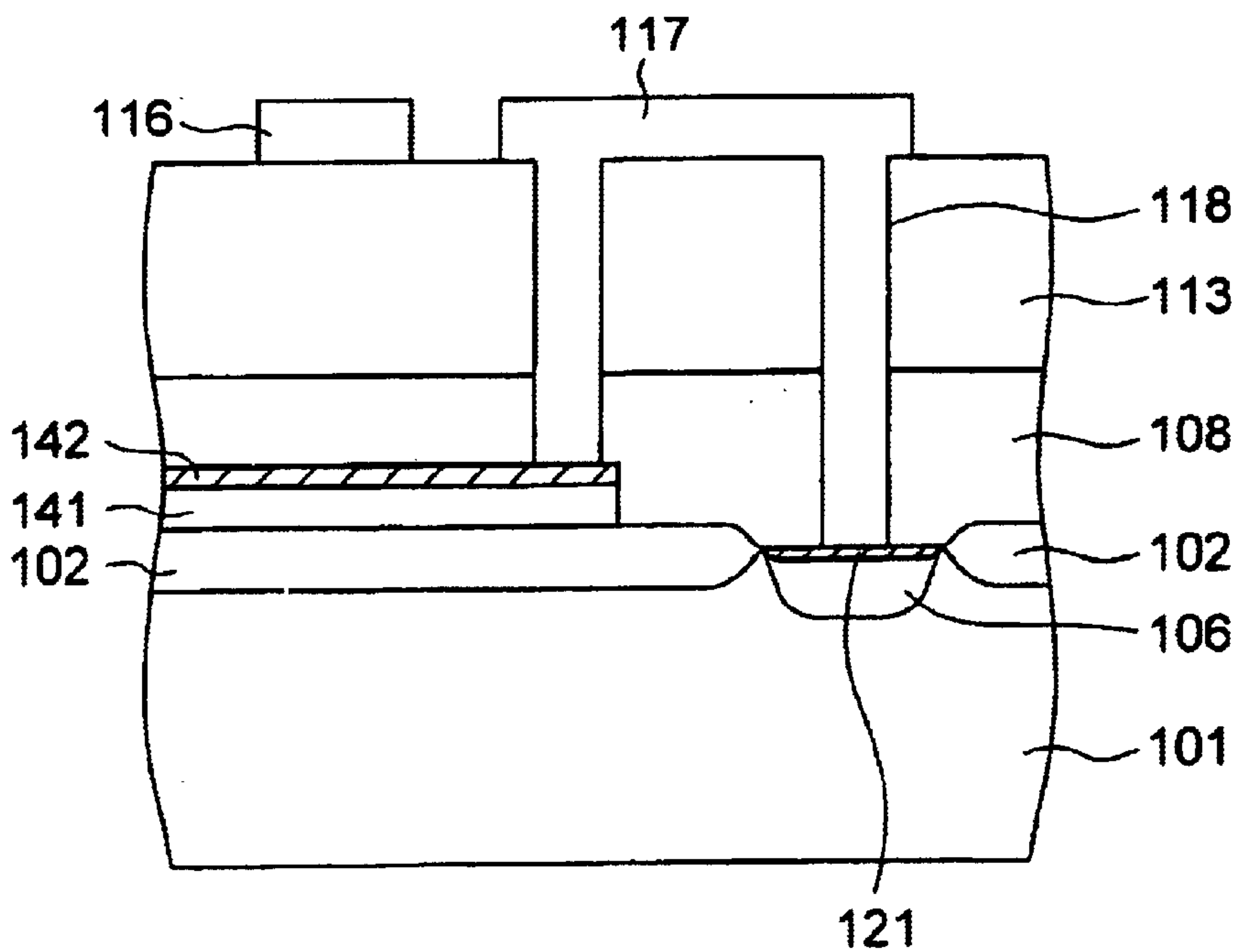
FIG. 6B d-d' SECTION
