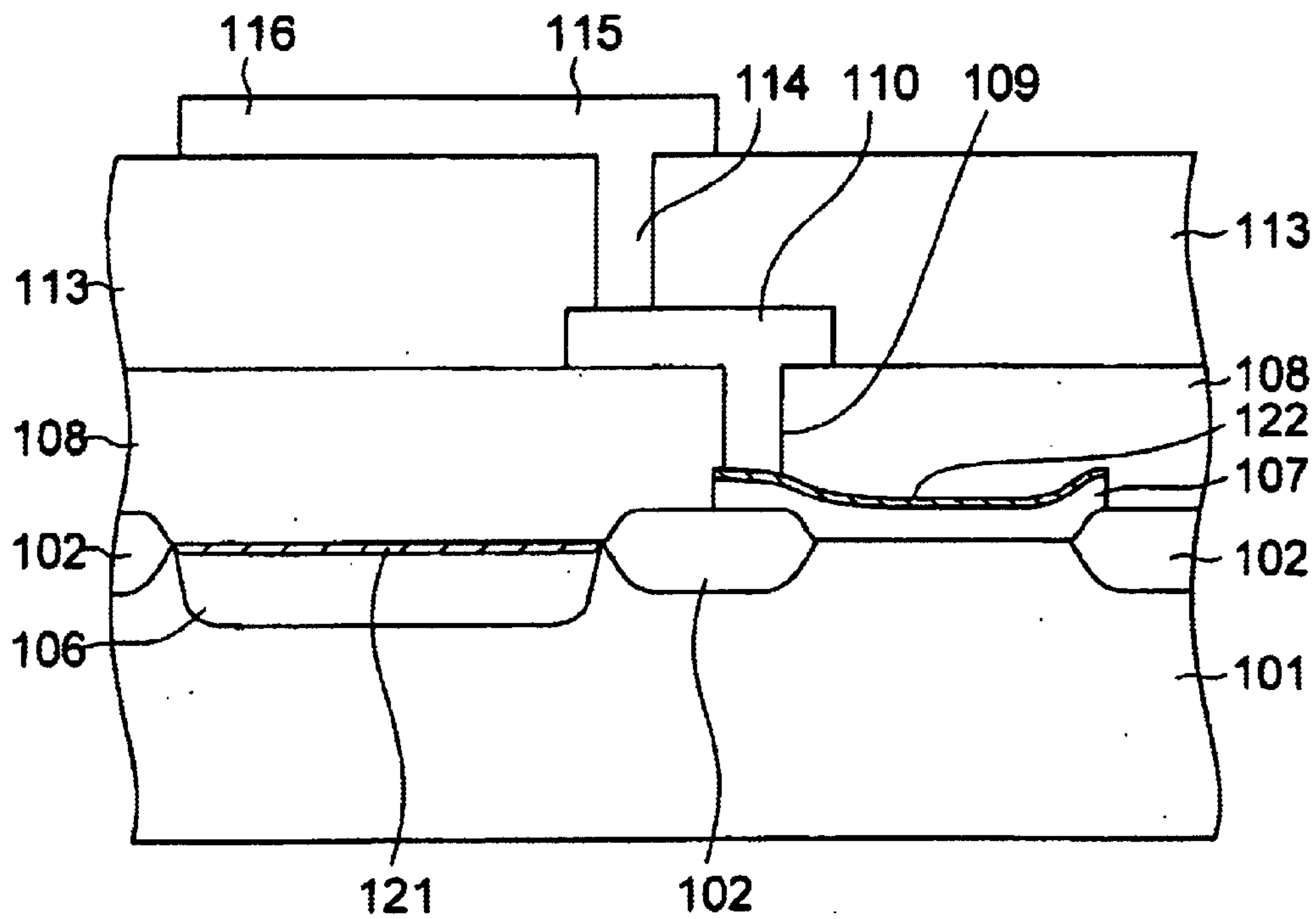
FIG. 2A a-a' SECTION
