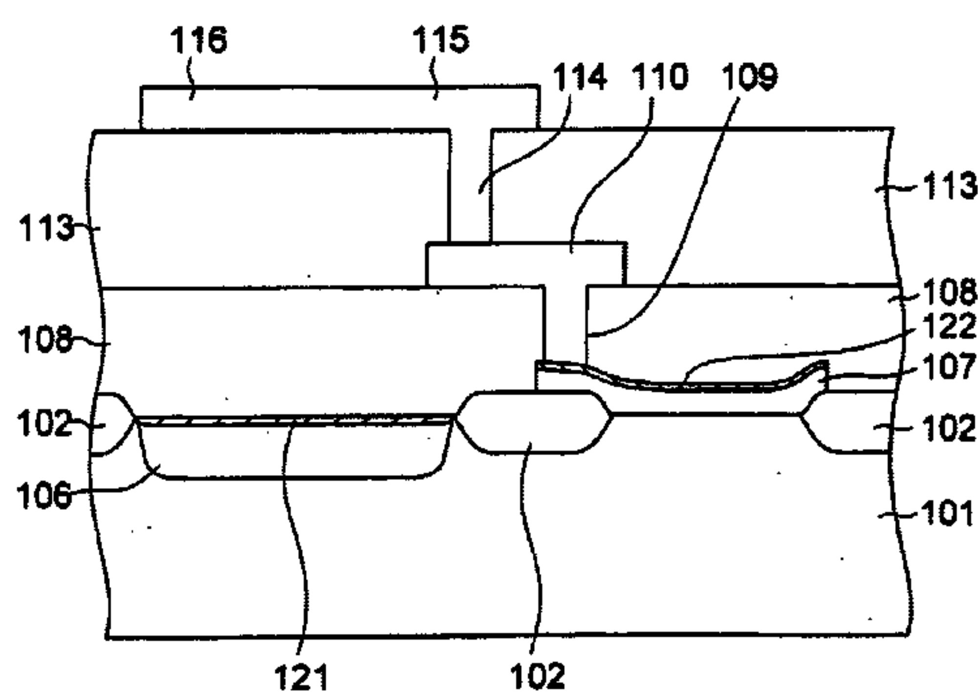
a-a' SECTION
