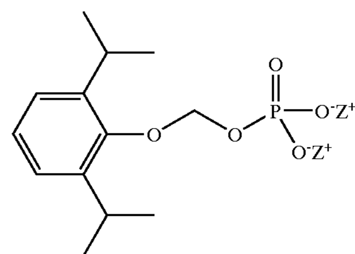
Propofol Prodrug
