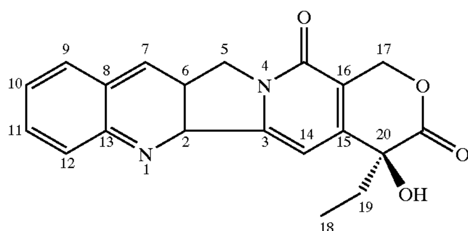
Camptothecin
