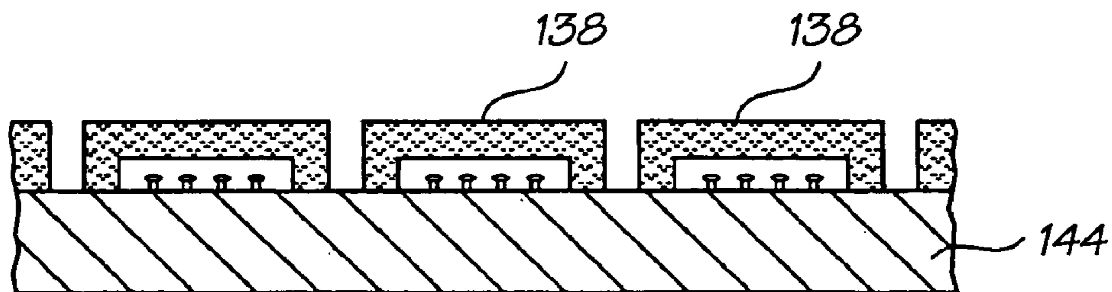
FIG. 20
