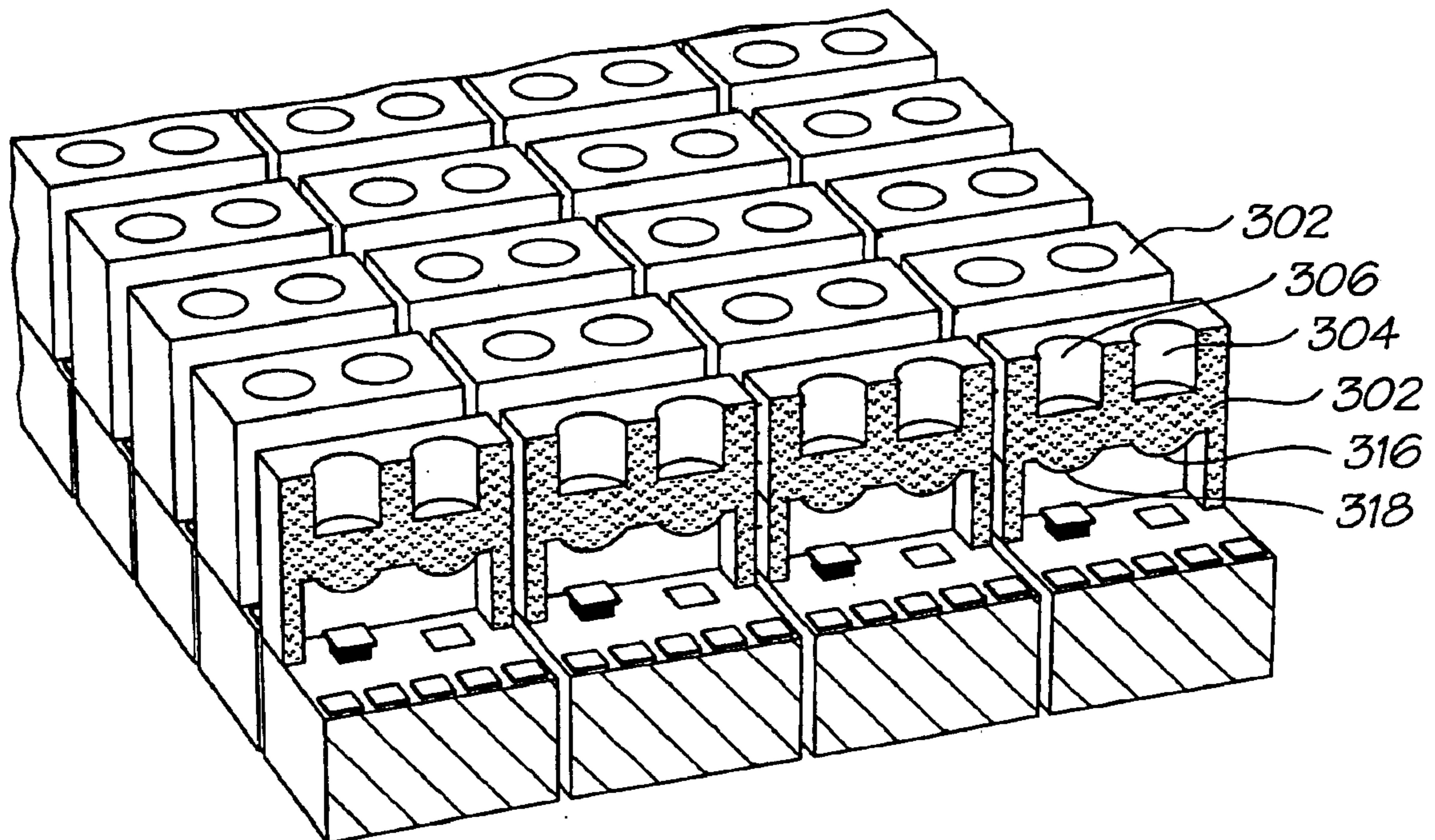
FIG. 34
