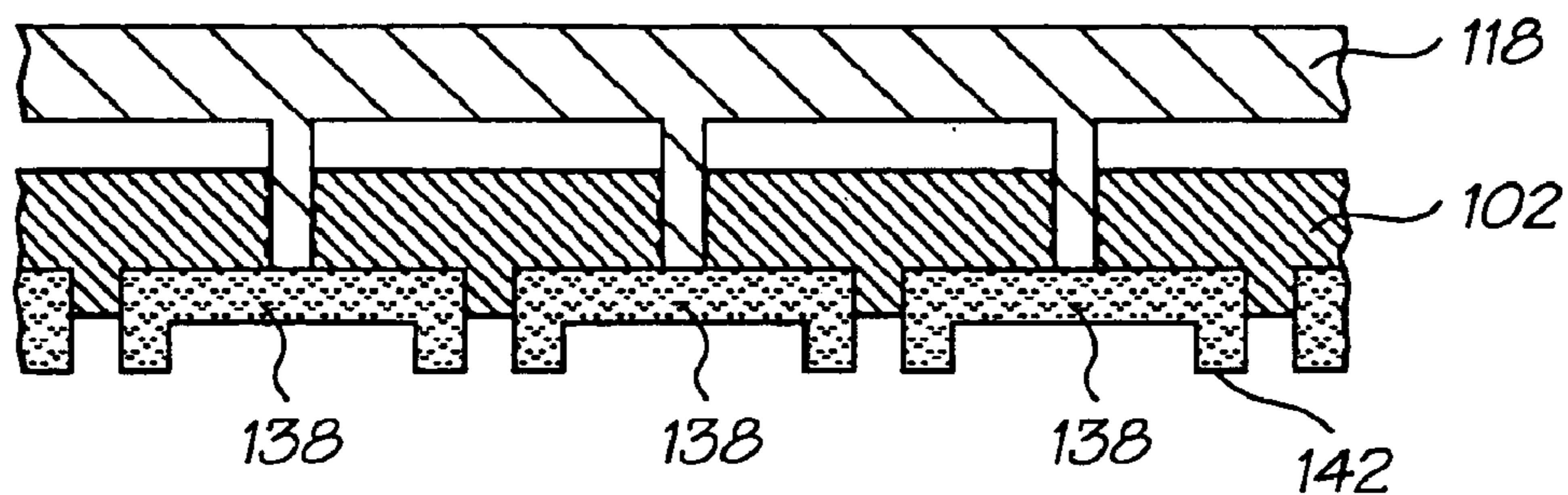
FIG. 18
