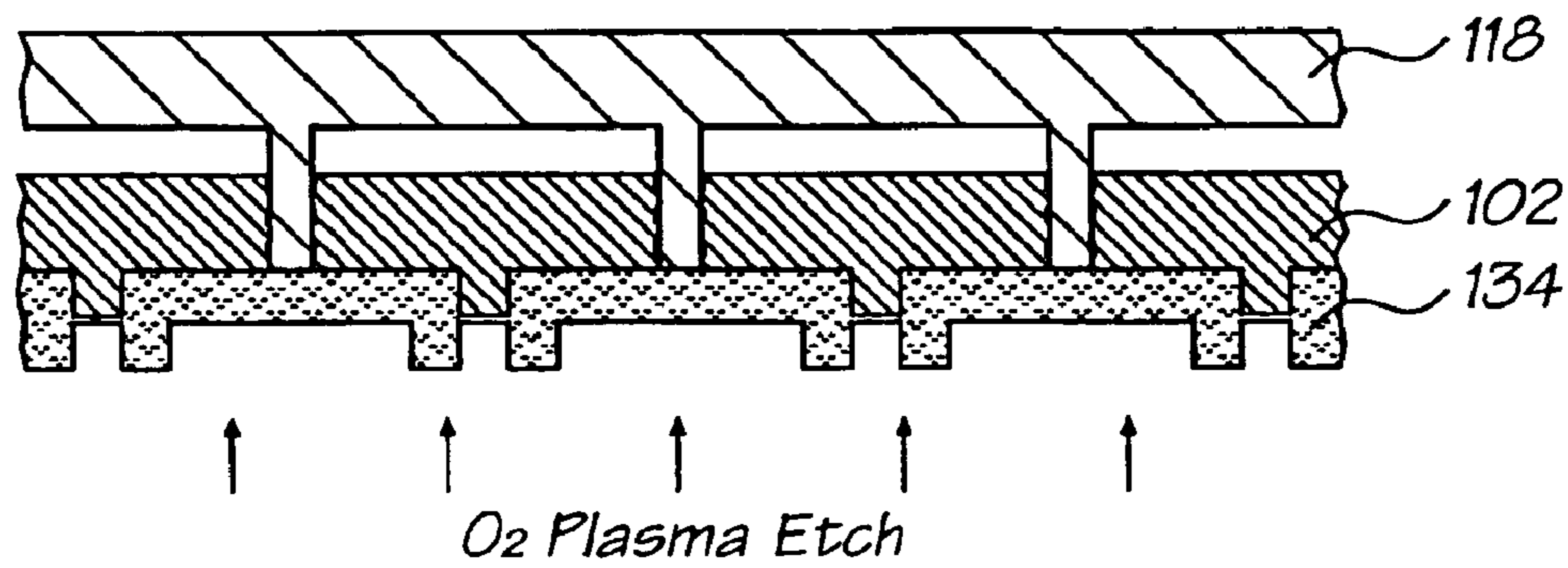
FIG. 17
