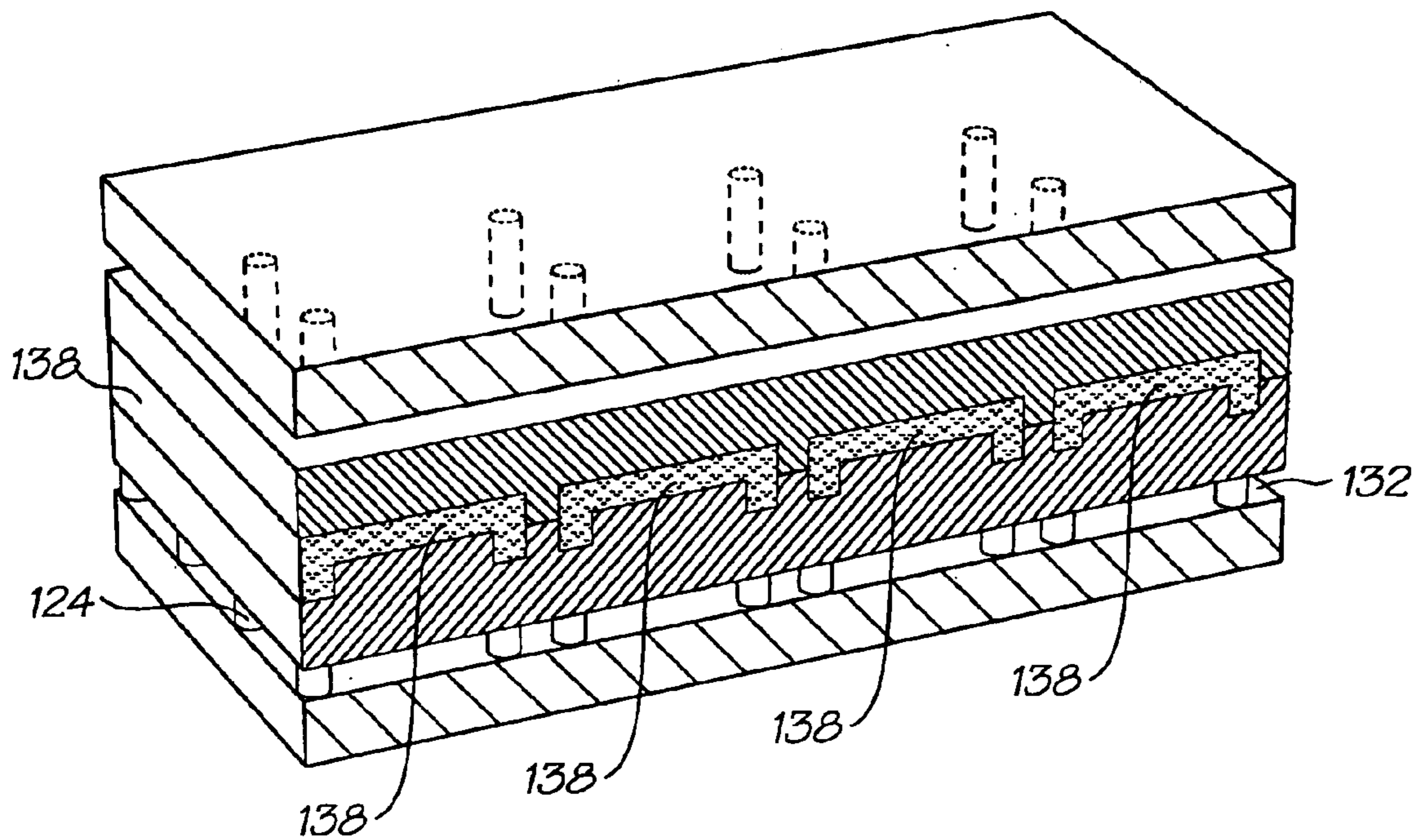
FIG. 14
