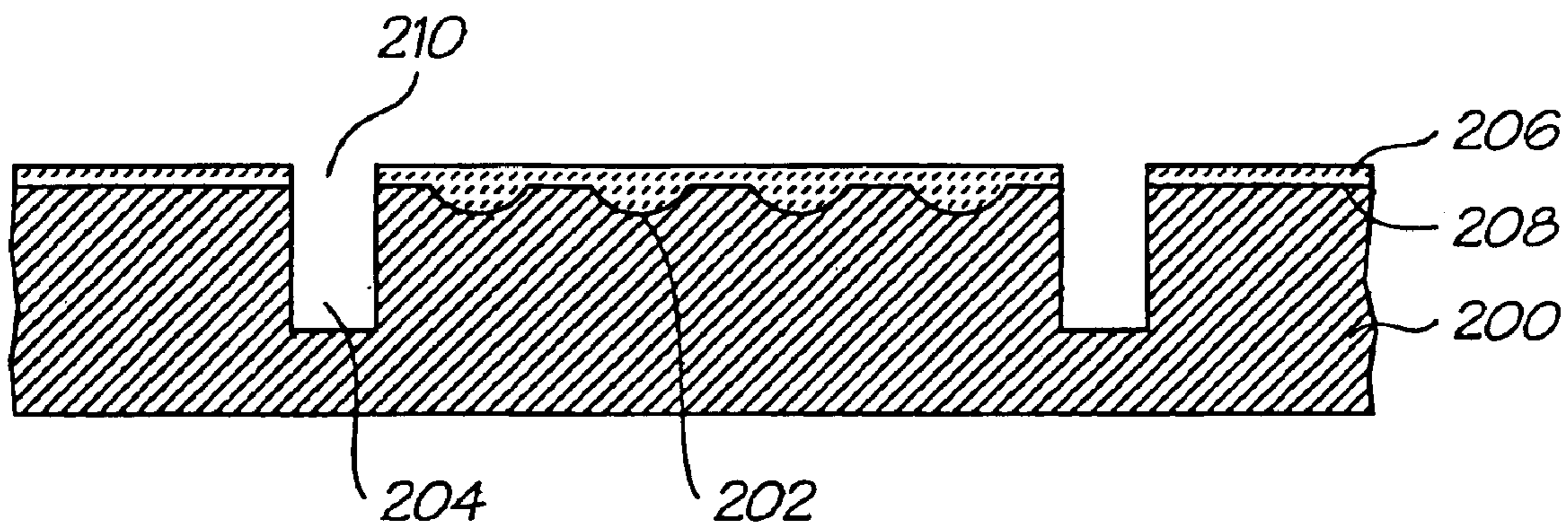
FIG. 23c
