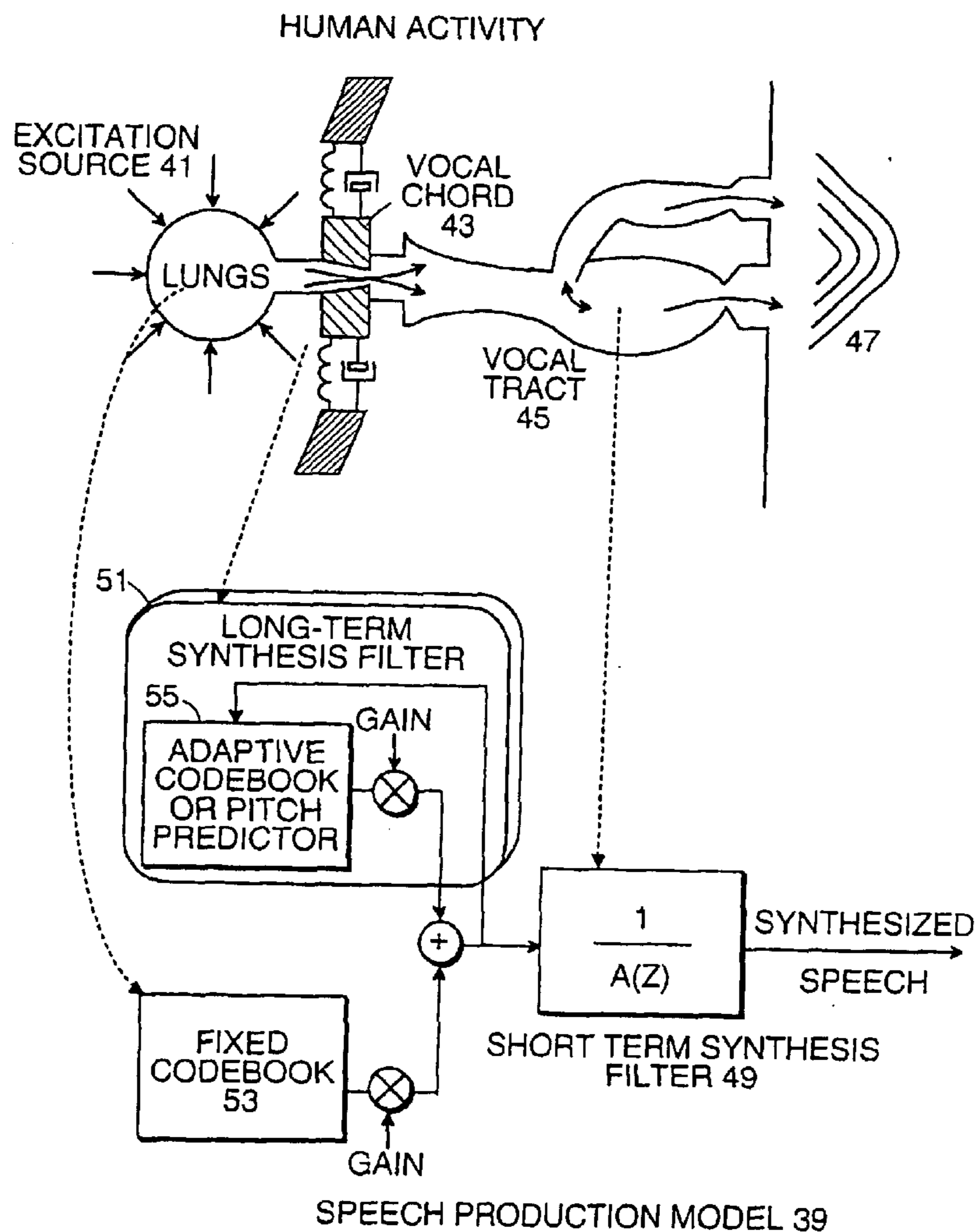
FIG. 1
