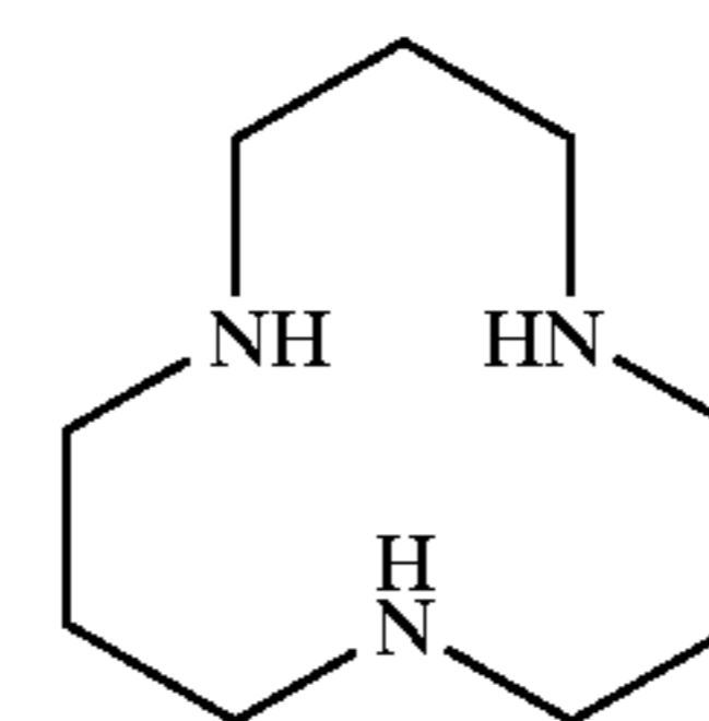
1,5,9-triazacyclododecane
