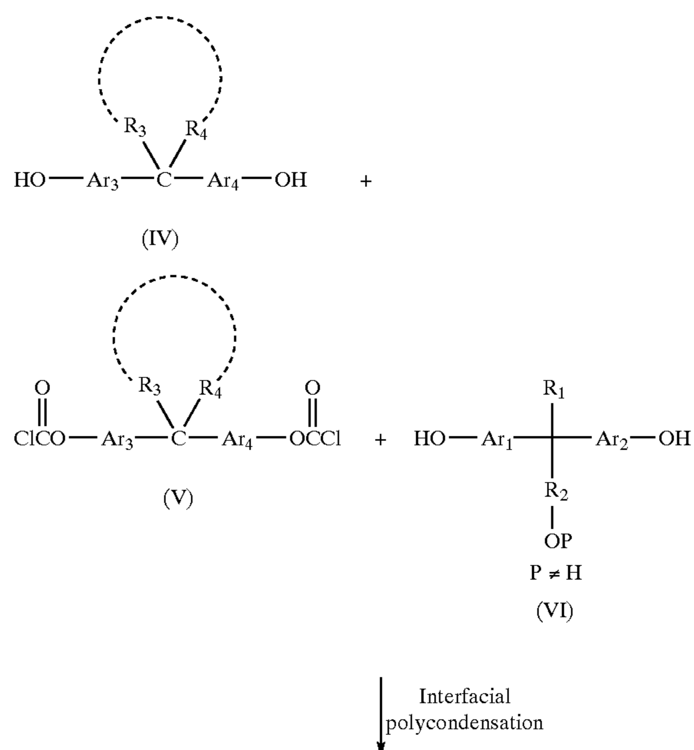
Scheme(II)
