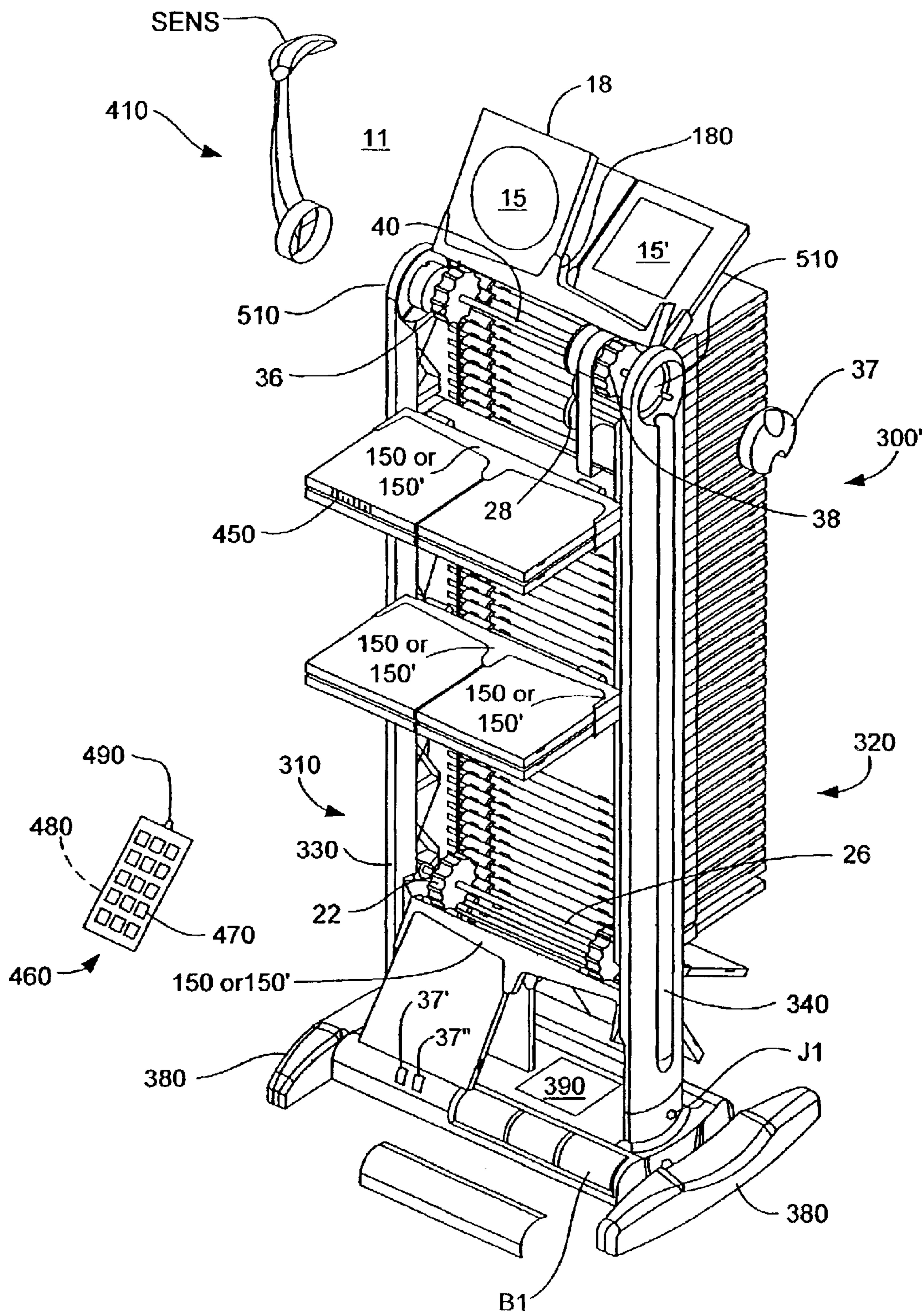
FIG.- 15C
