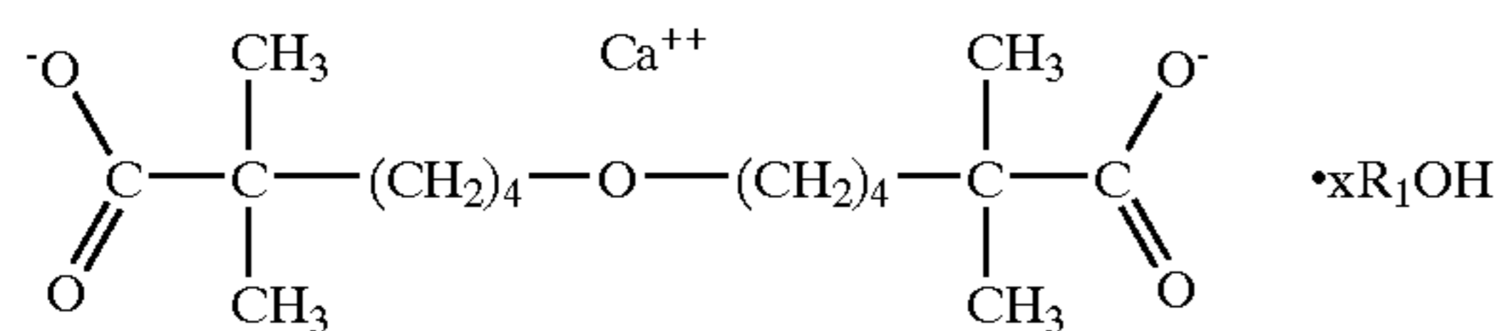
CI-1027
