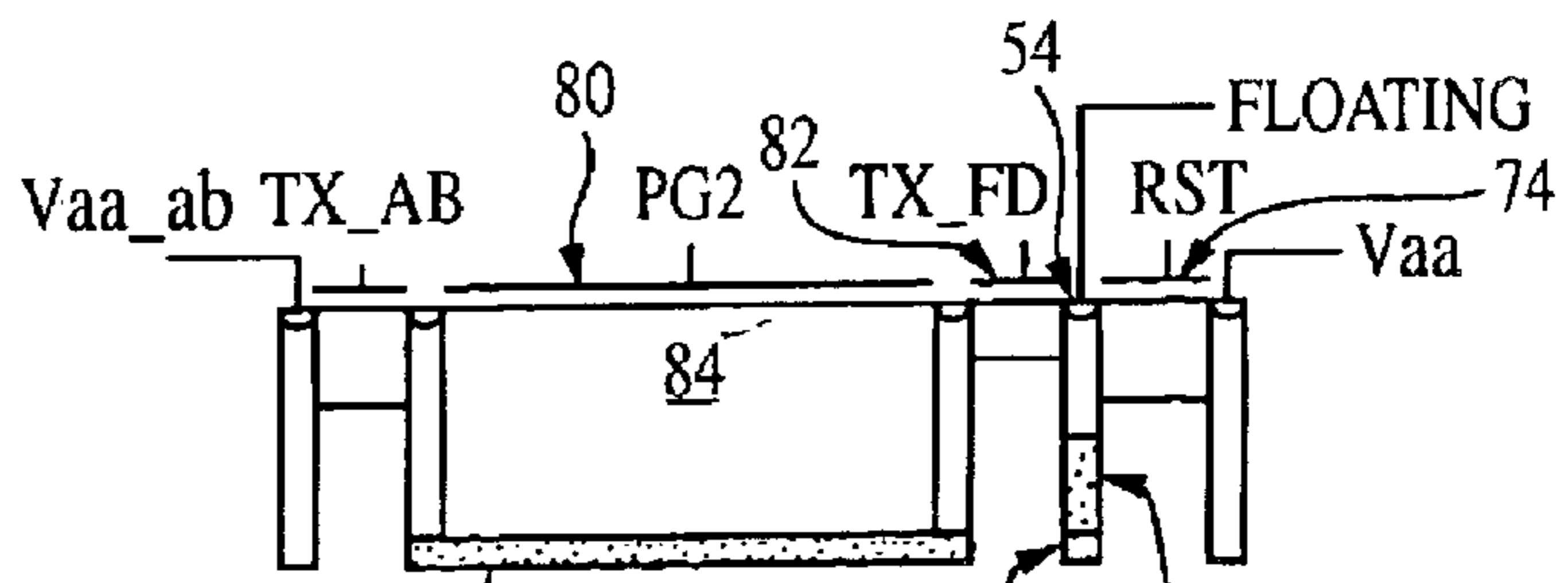
Qerr(TX_FD) Qsig FIG. 6F
