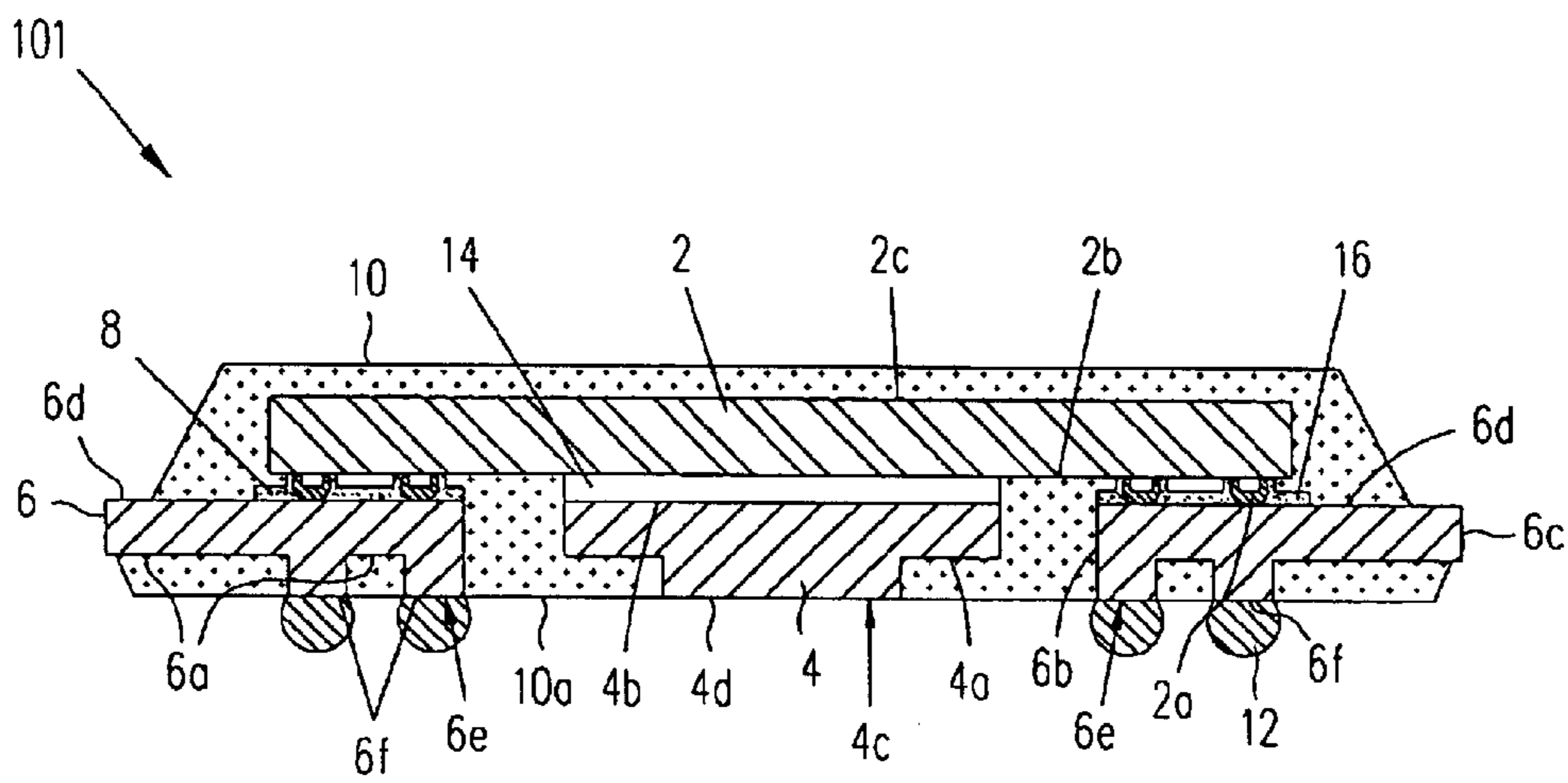
FIG. 2b
