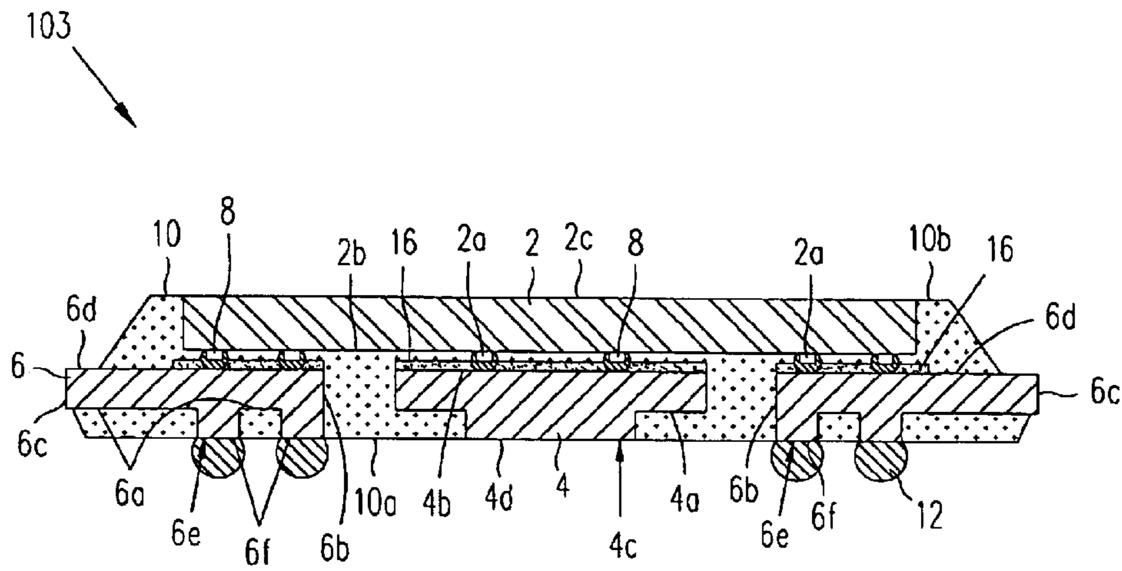
FIG. 4b
