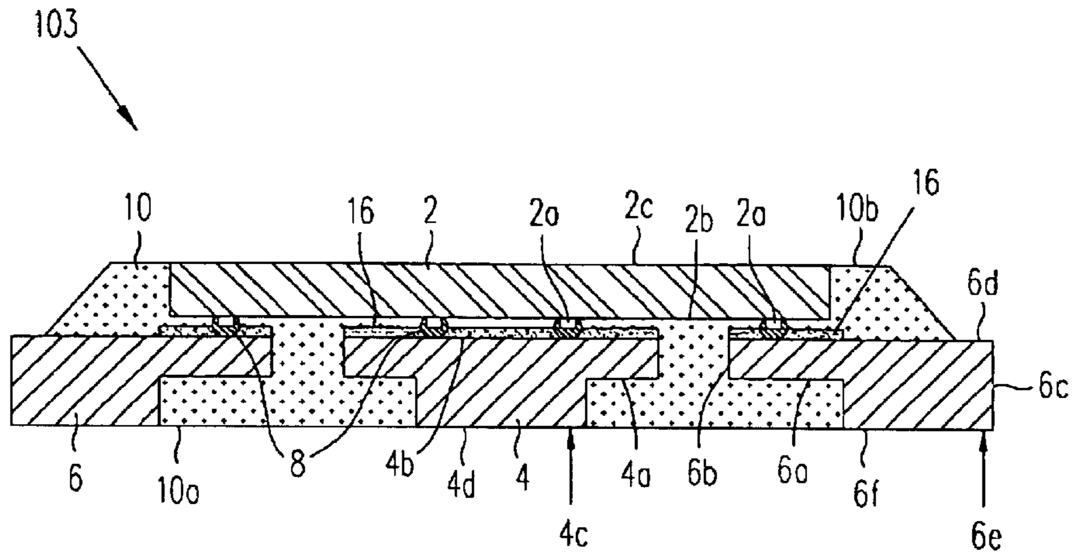
FIG. 4a
