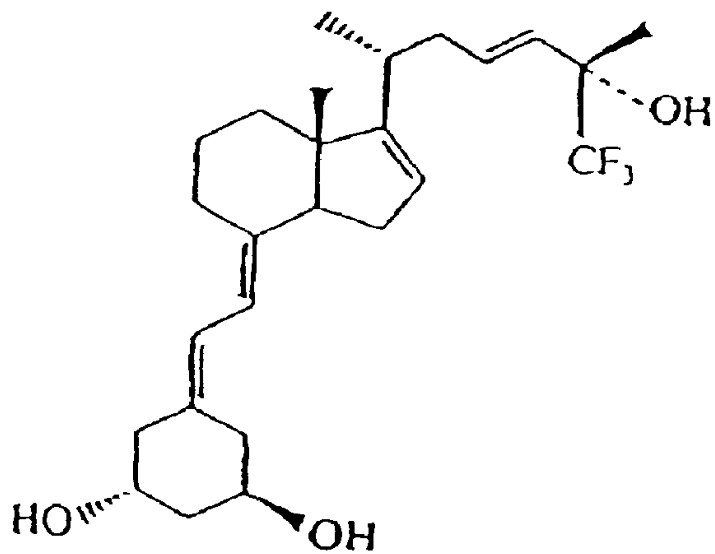
1,25S-(OH) 2 -16,23-diene-26-F 3 -19-nor D 3
