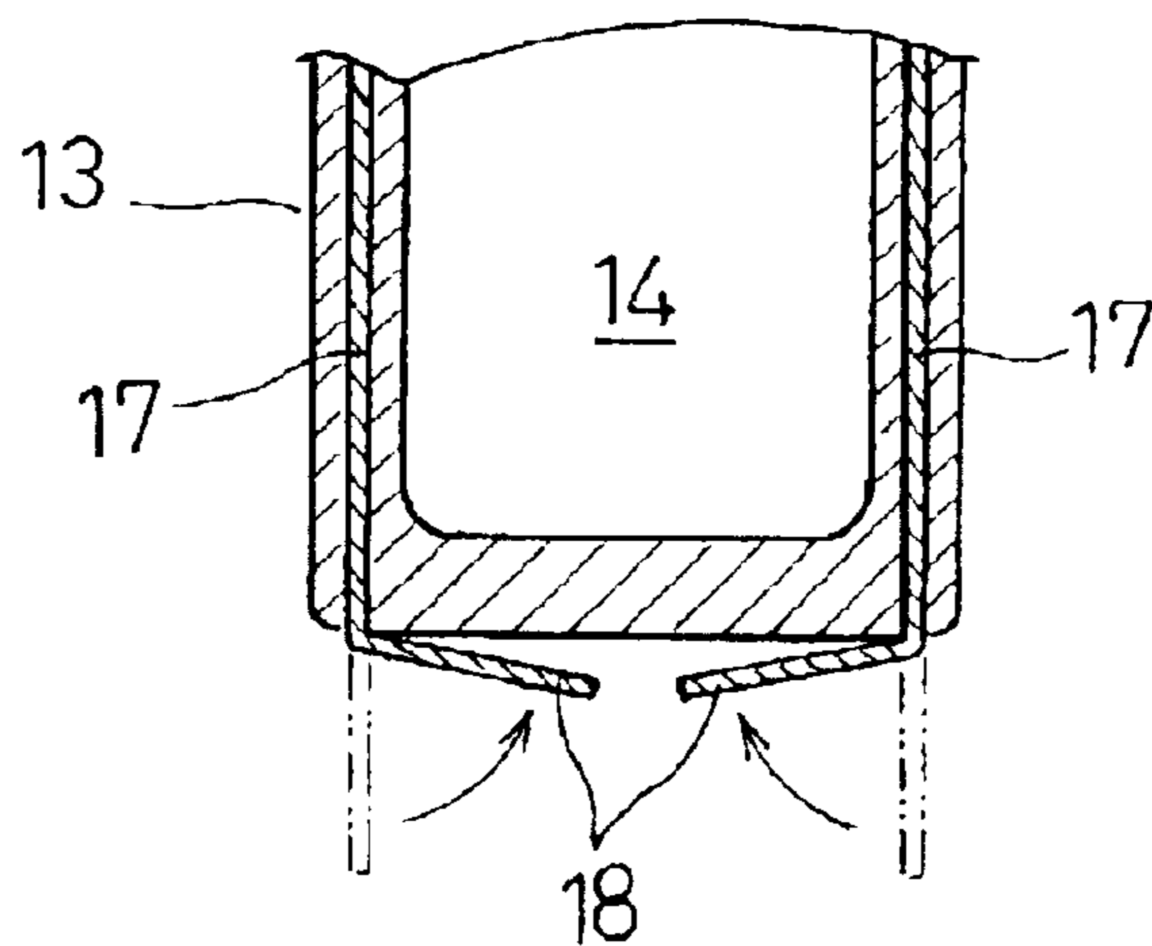
Fig. 3C
