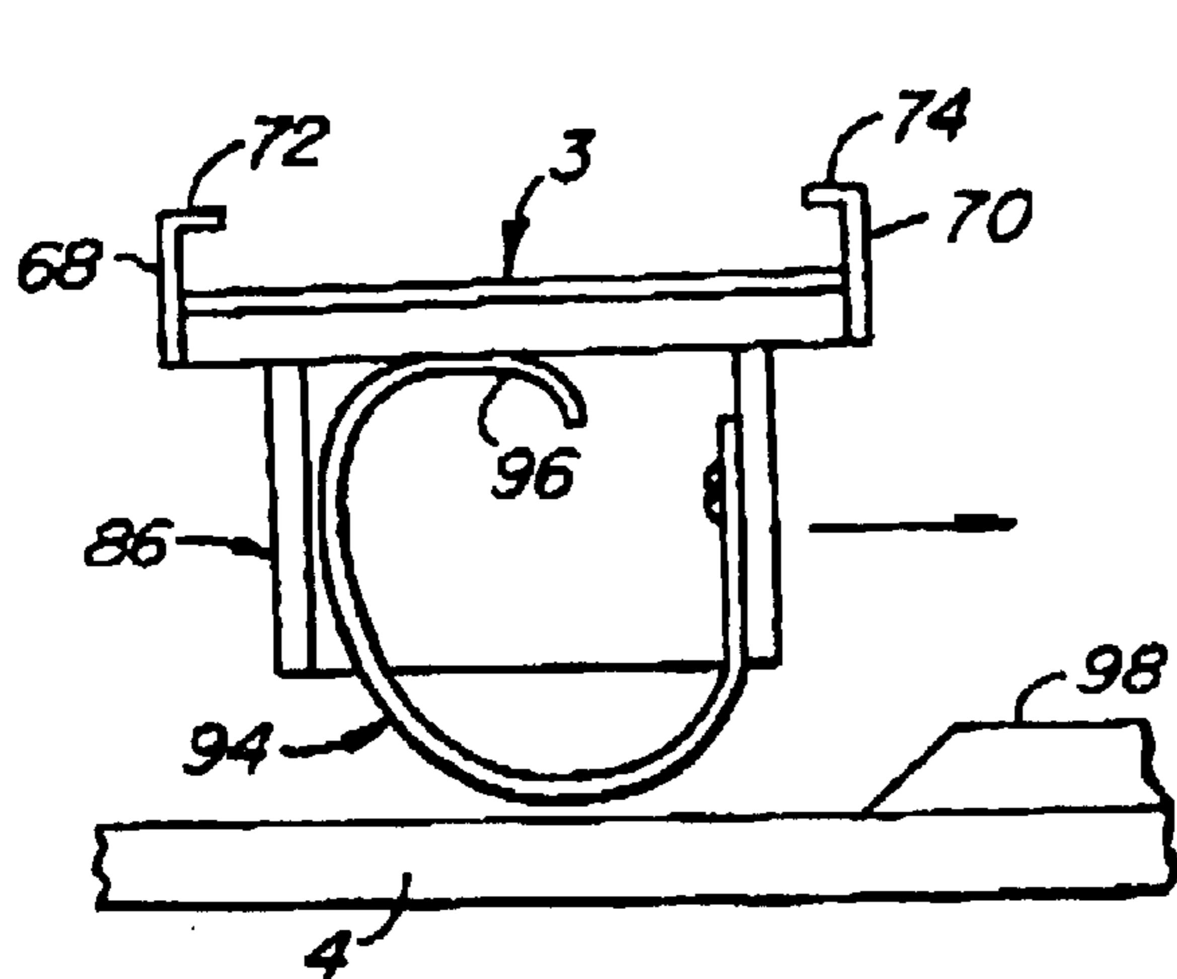
FIG. 9A.
