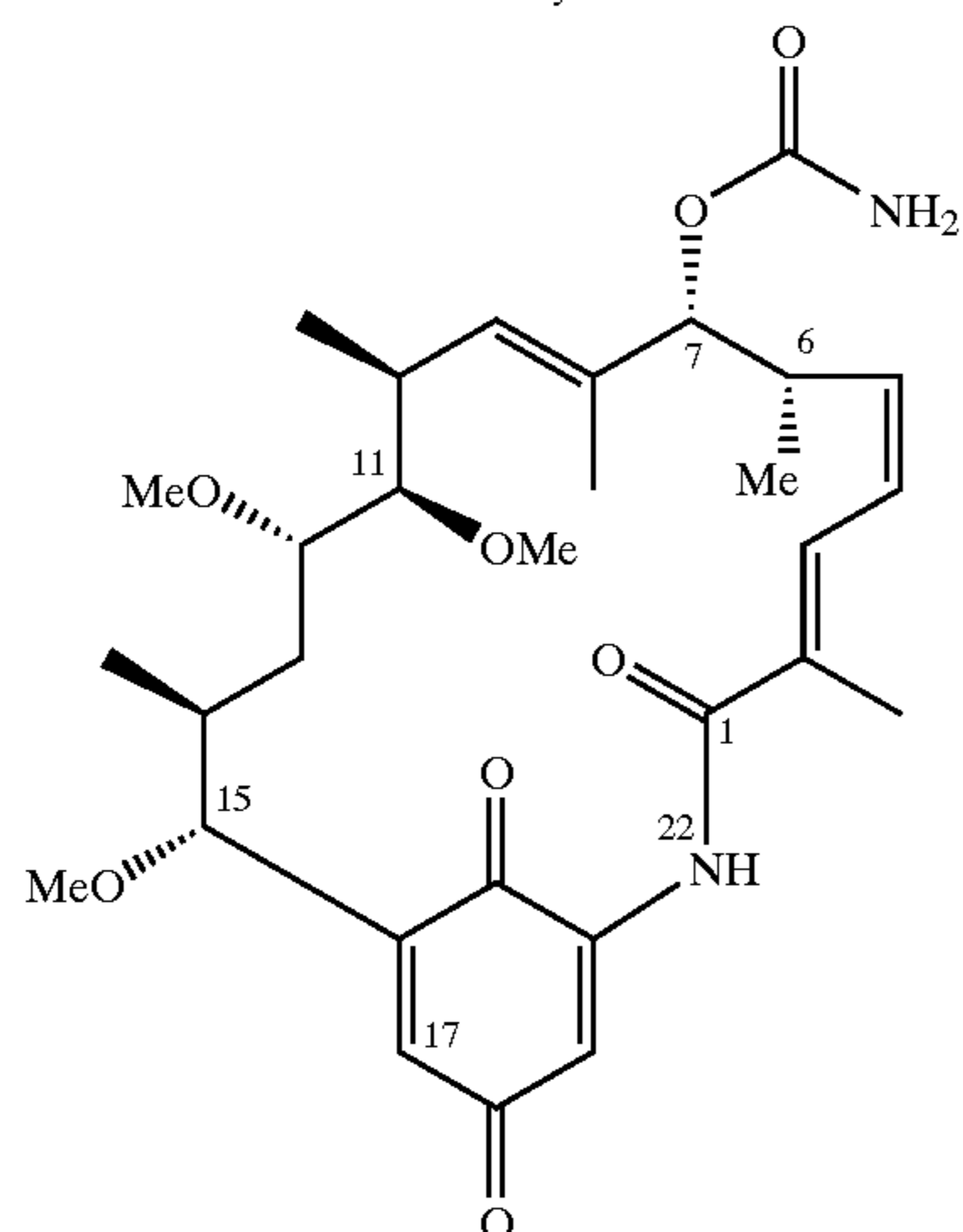
Macbecin I
