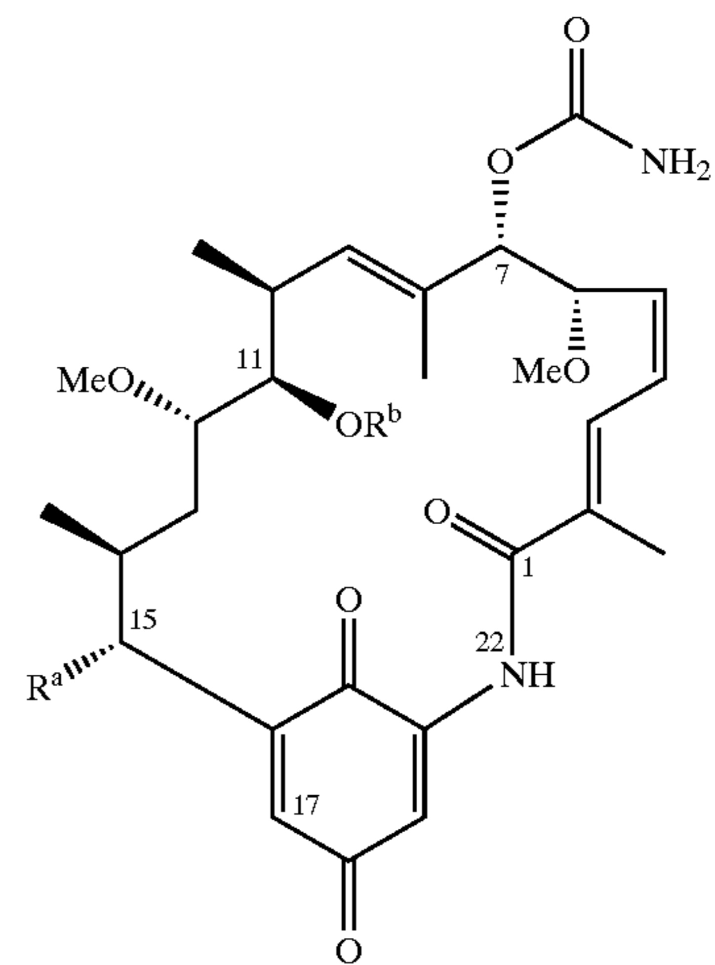
Herbimycins
