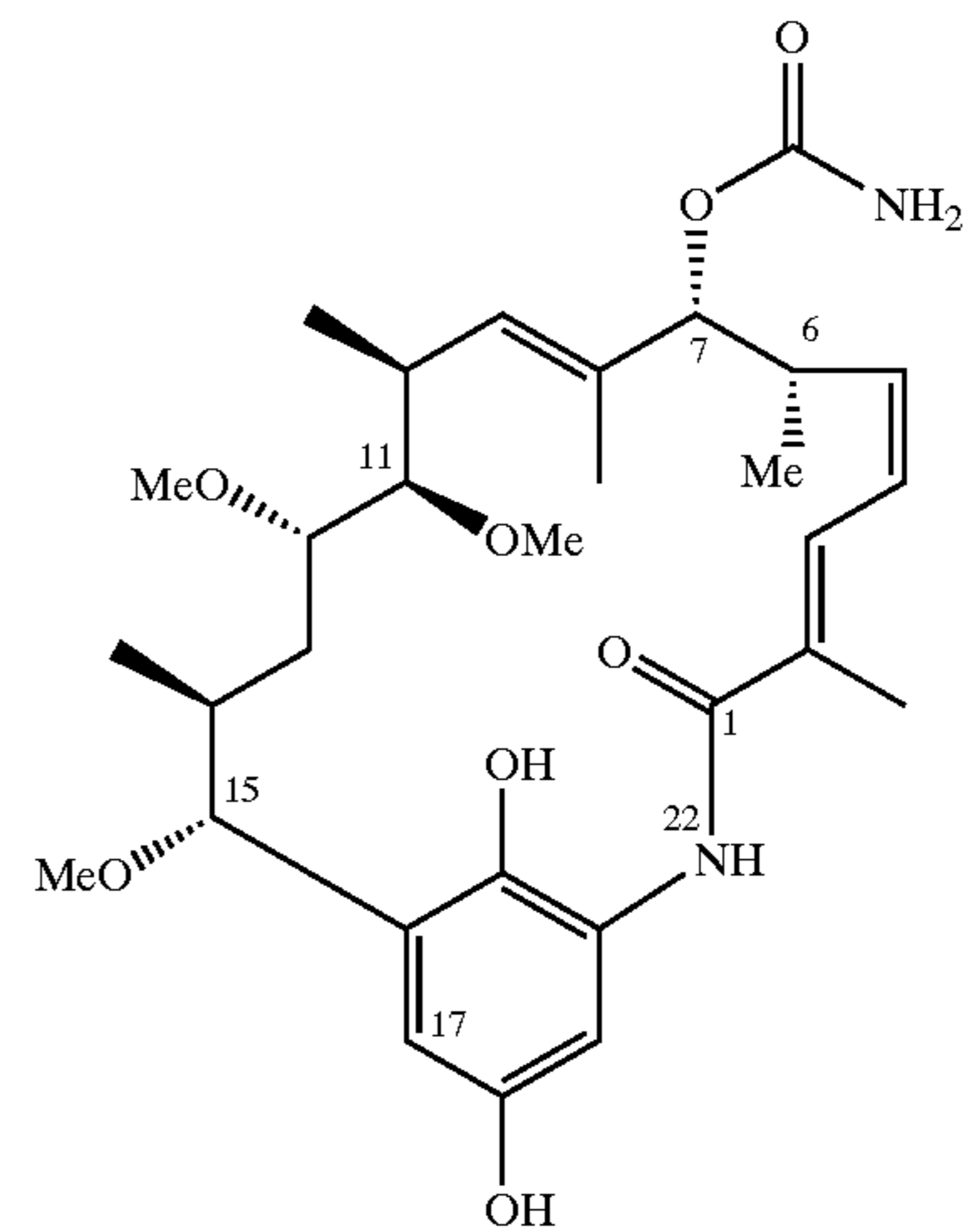
Macbecin II
