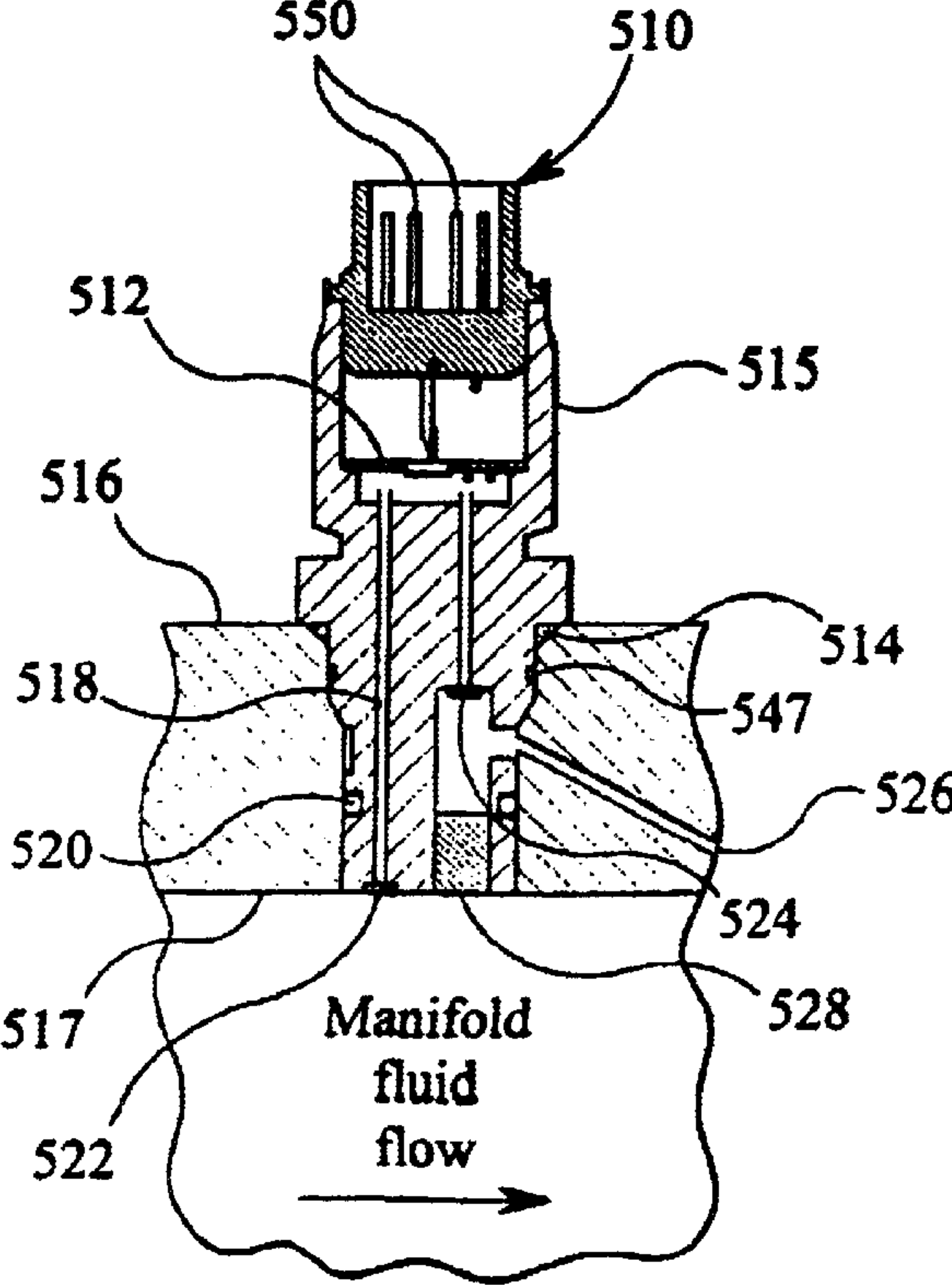
FIG 4 section A-A
