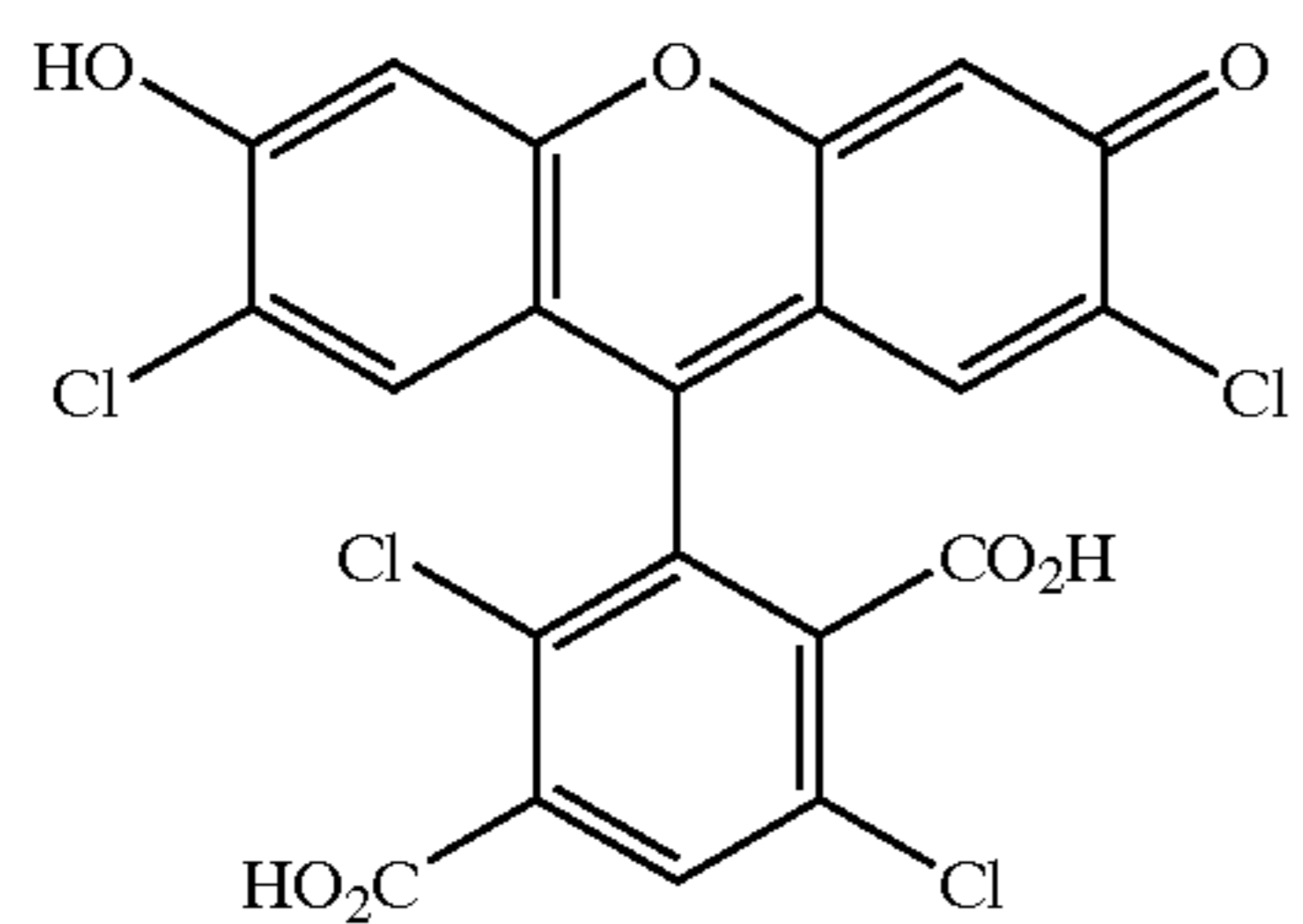
TET
