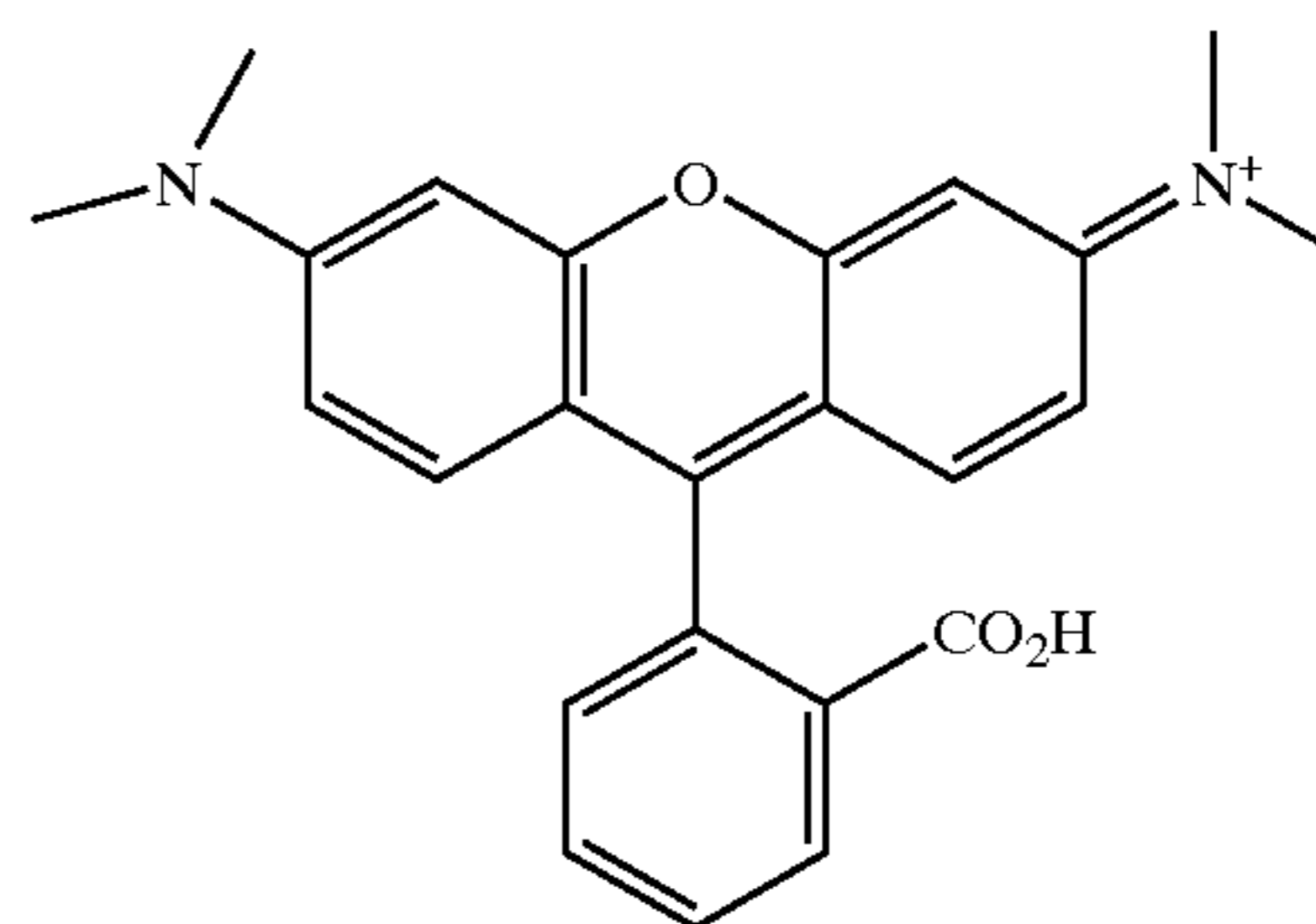
Rhodamine
