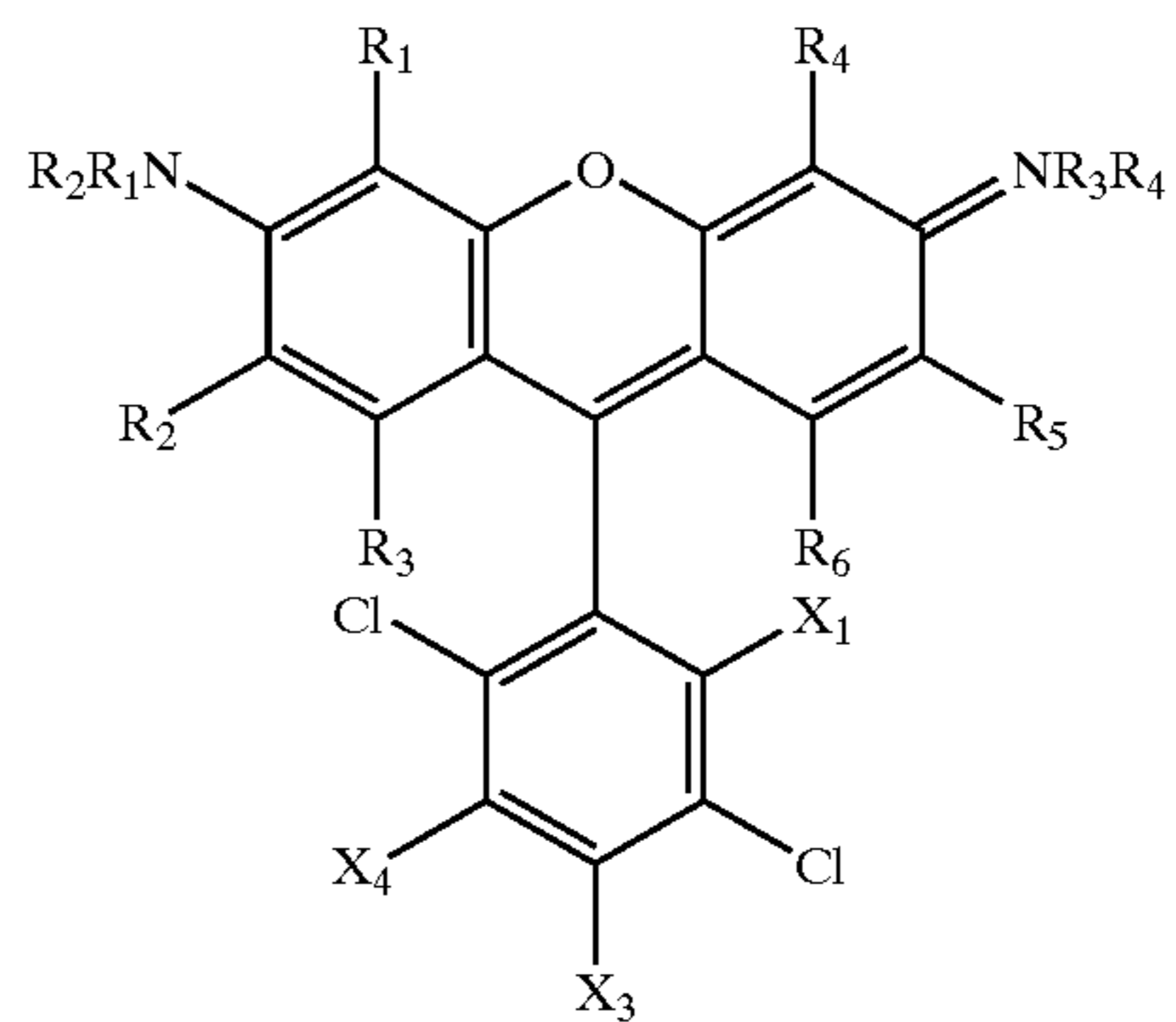
4,7 Dichlororhodamine
