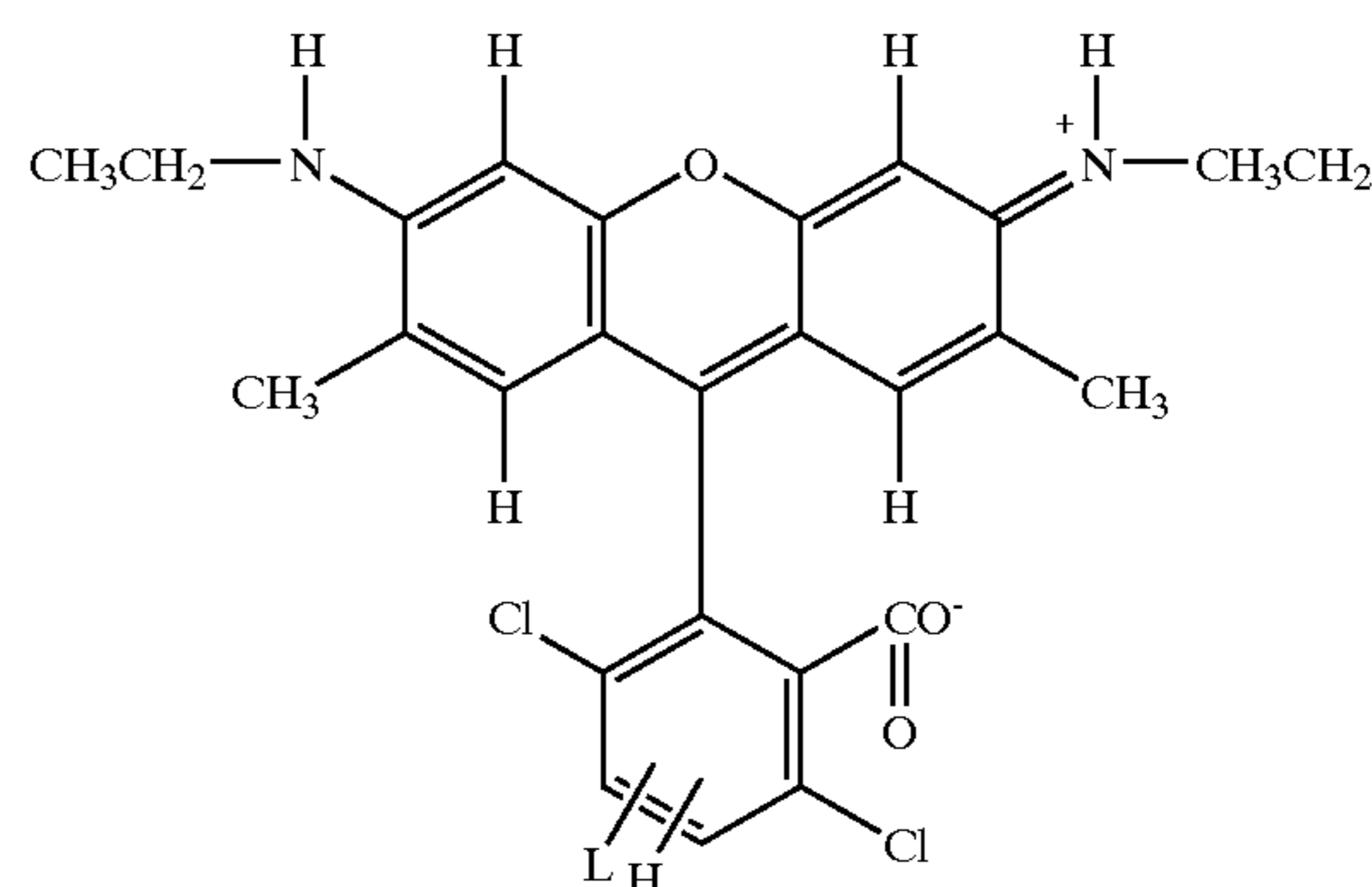
DR6G-2
