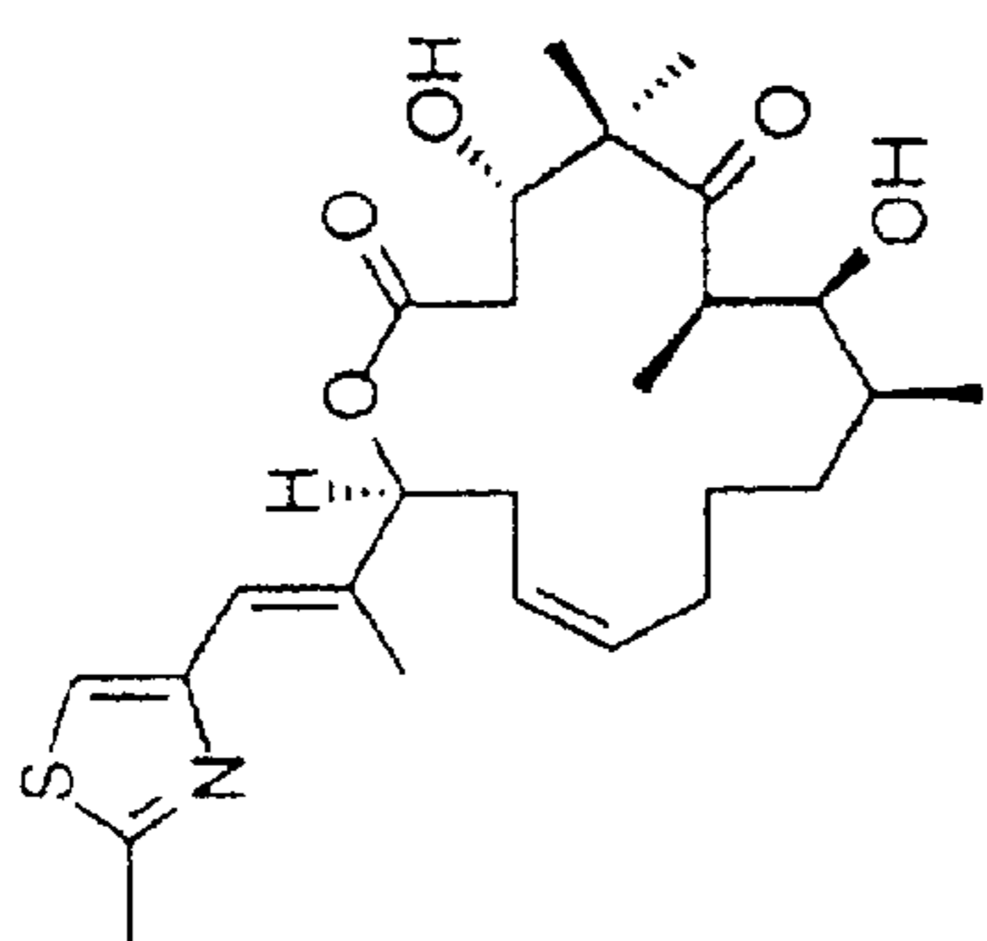
desoxyepothilone A
