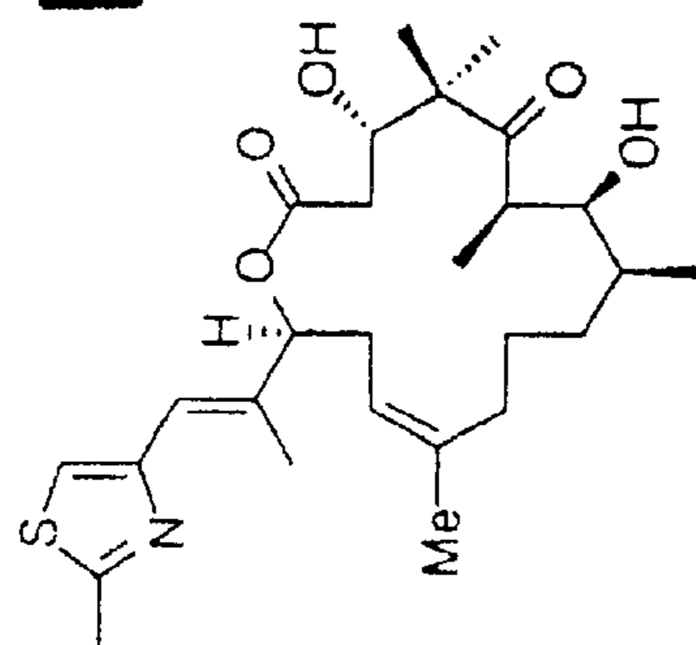
desoxyepothilone B
