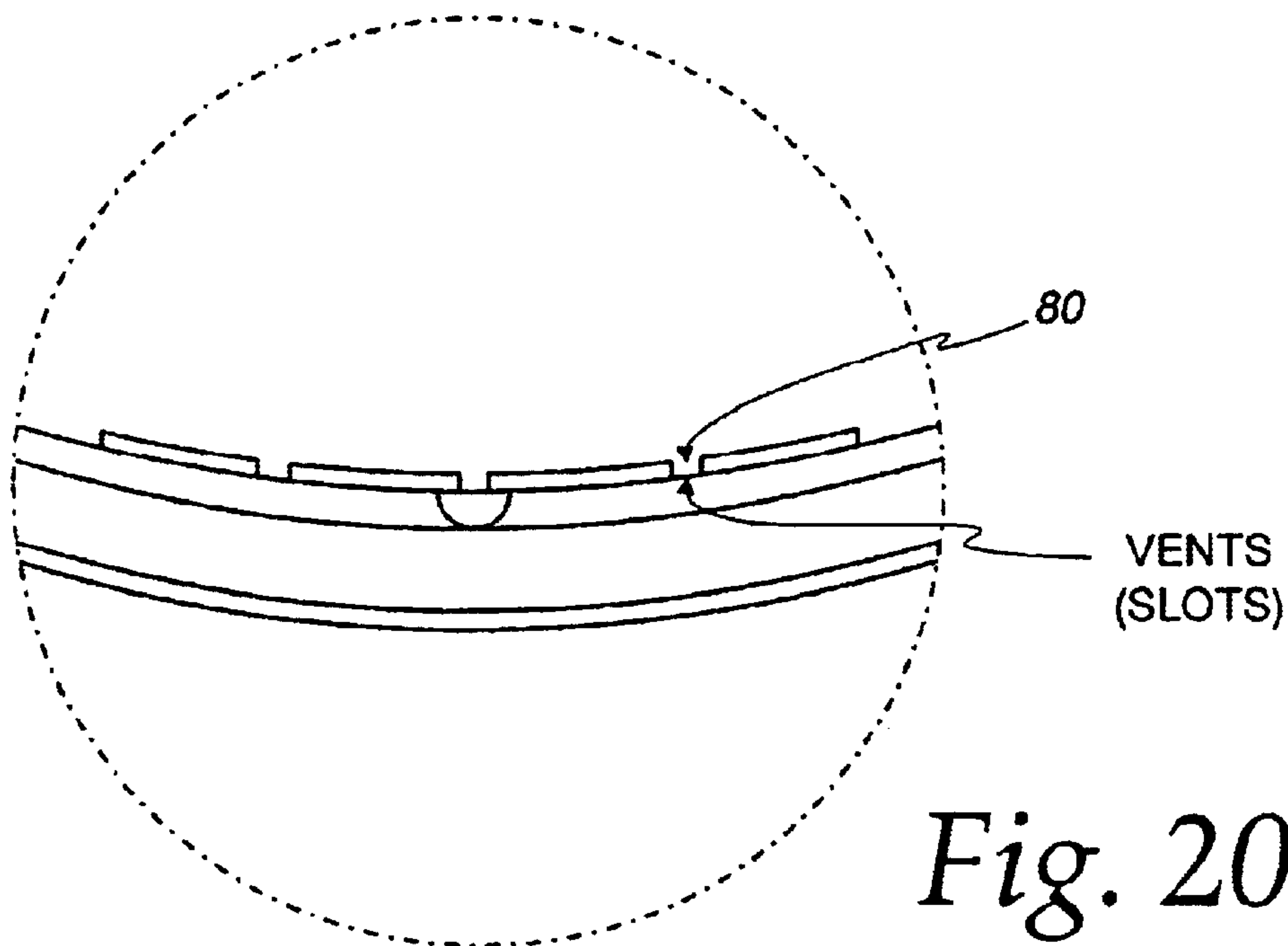
DETAIL Fig. 20
