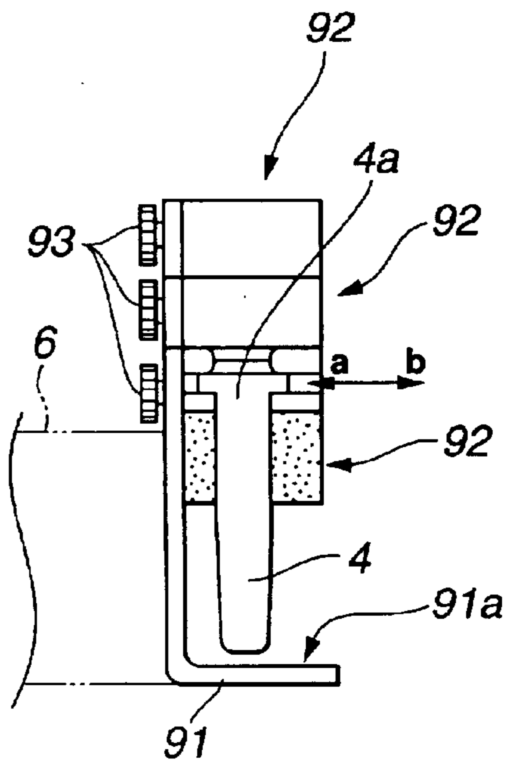
FIG.12B
