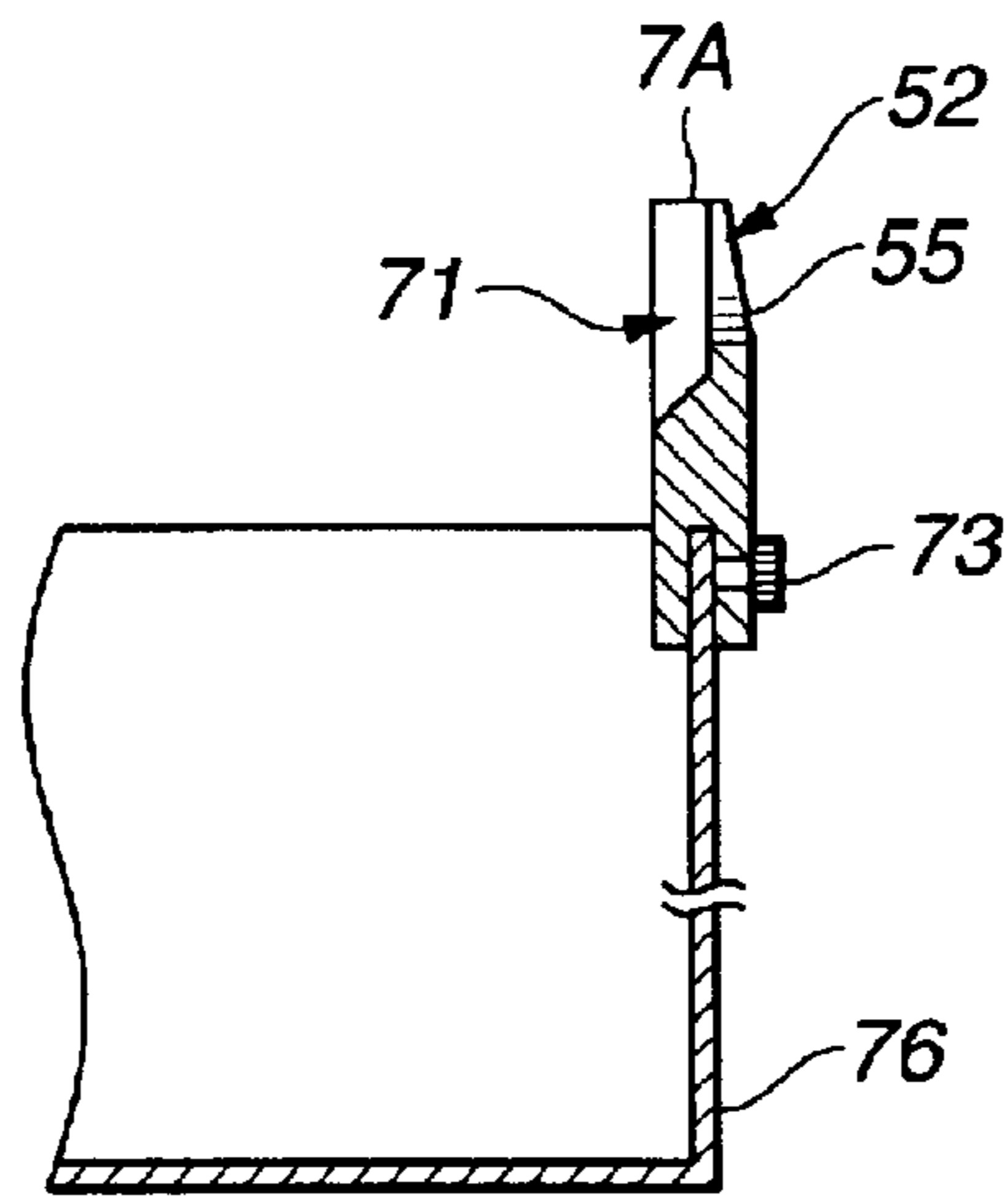
FIG.7B
