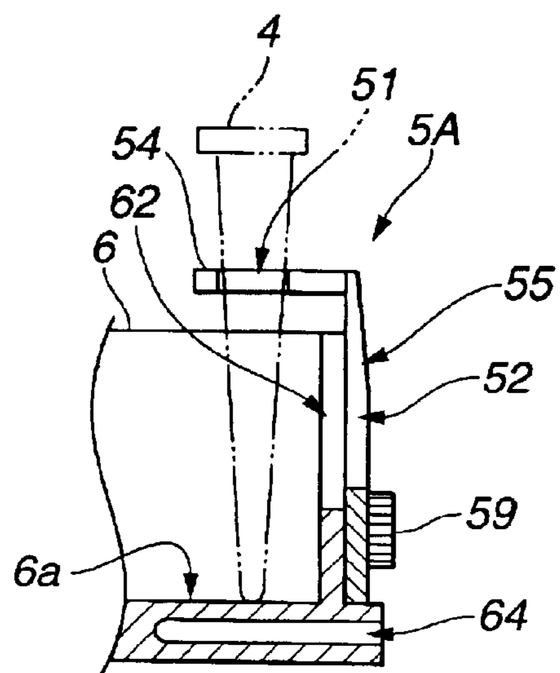
FIG.4C
