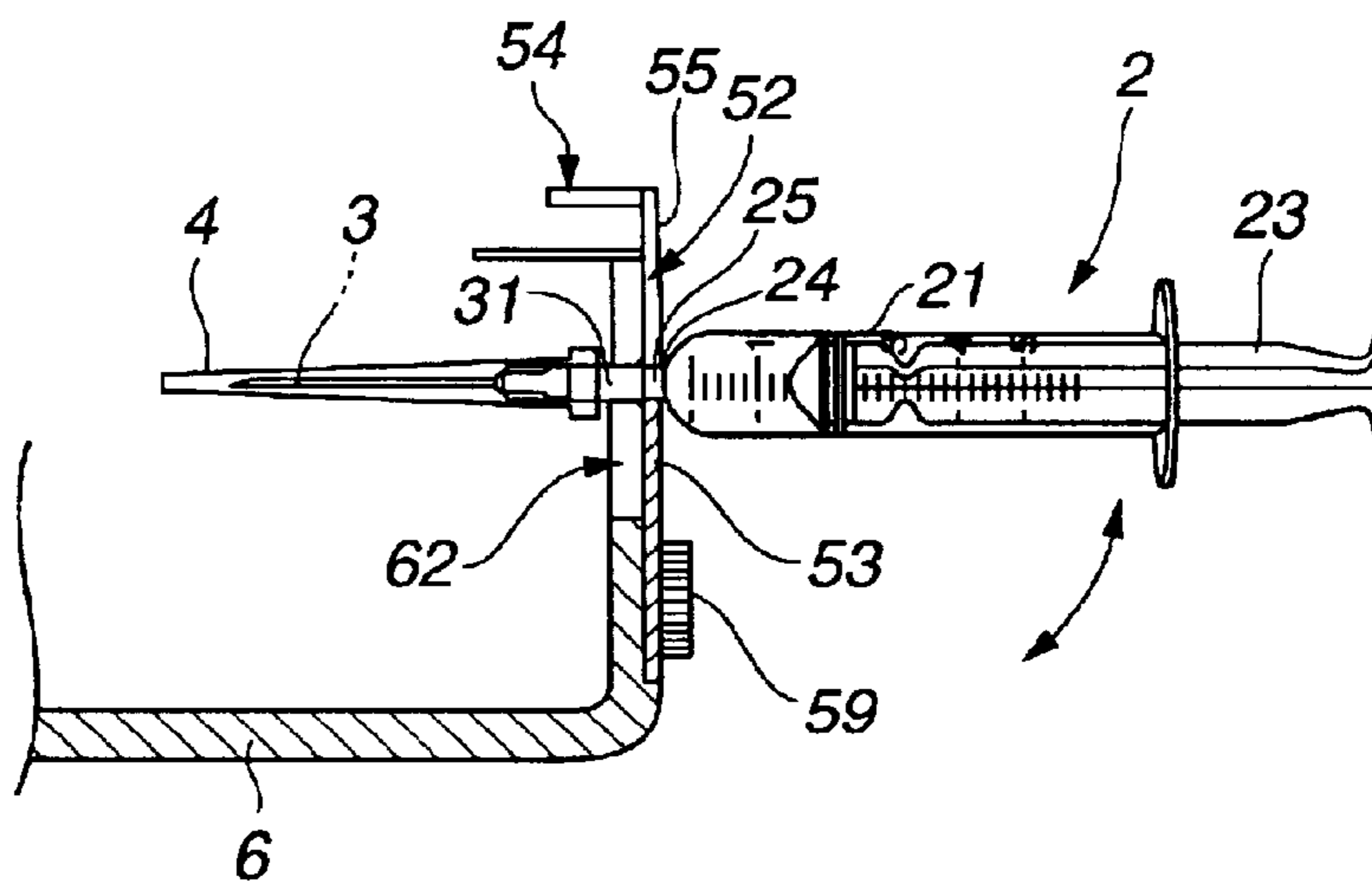
FIG.6B
