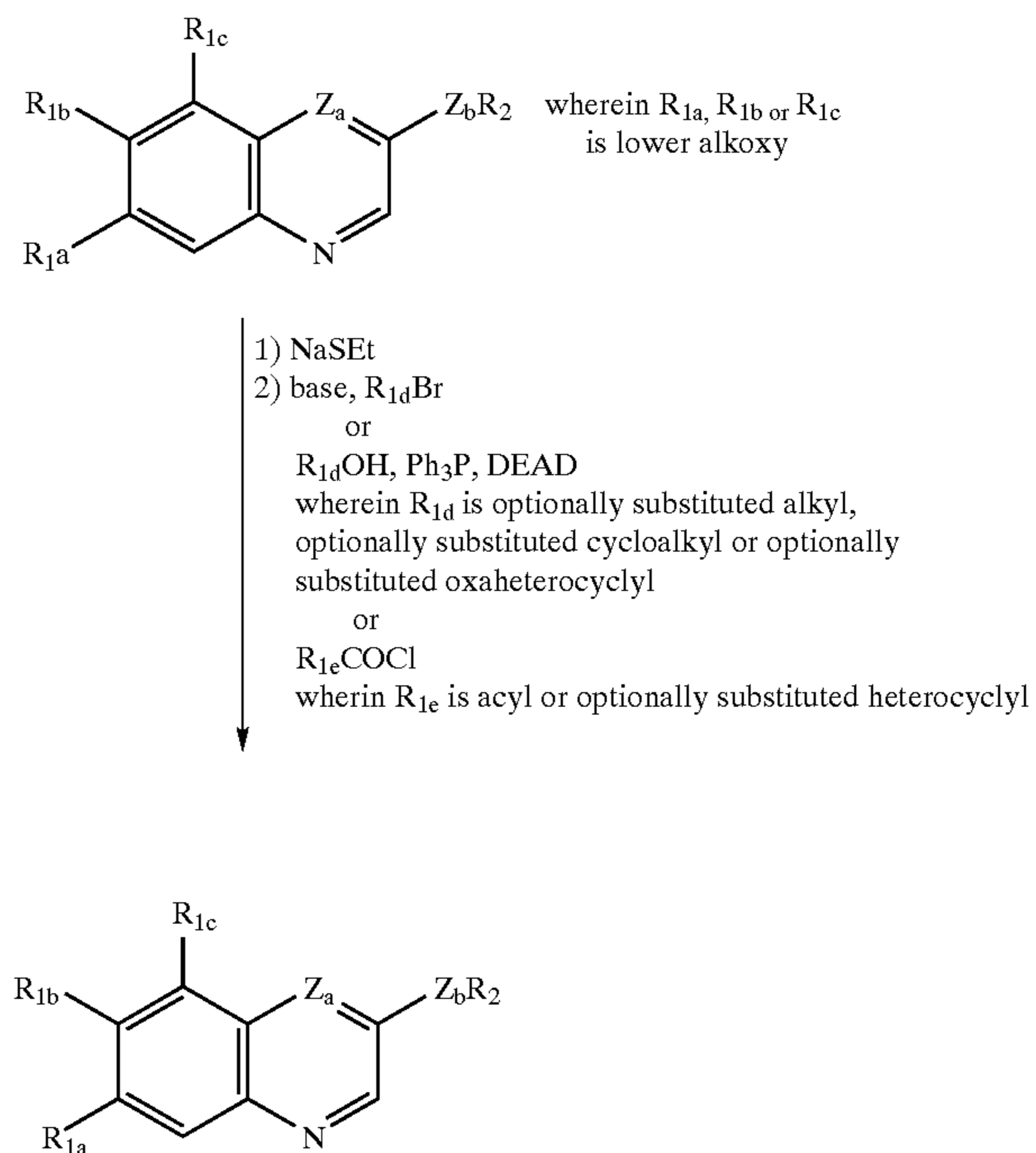
Scheme VI
