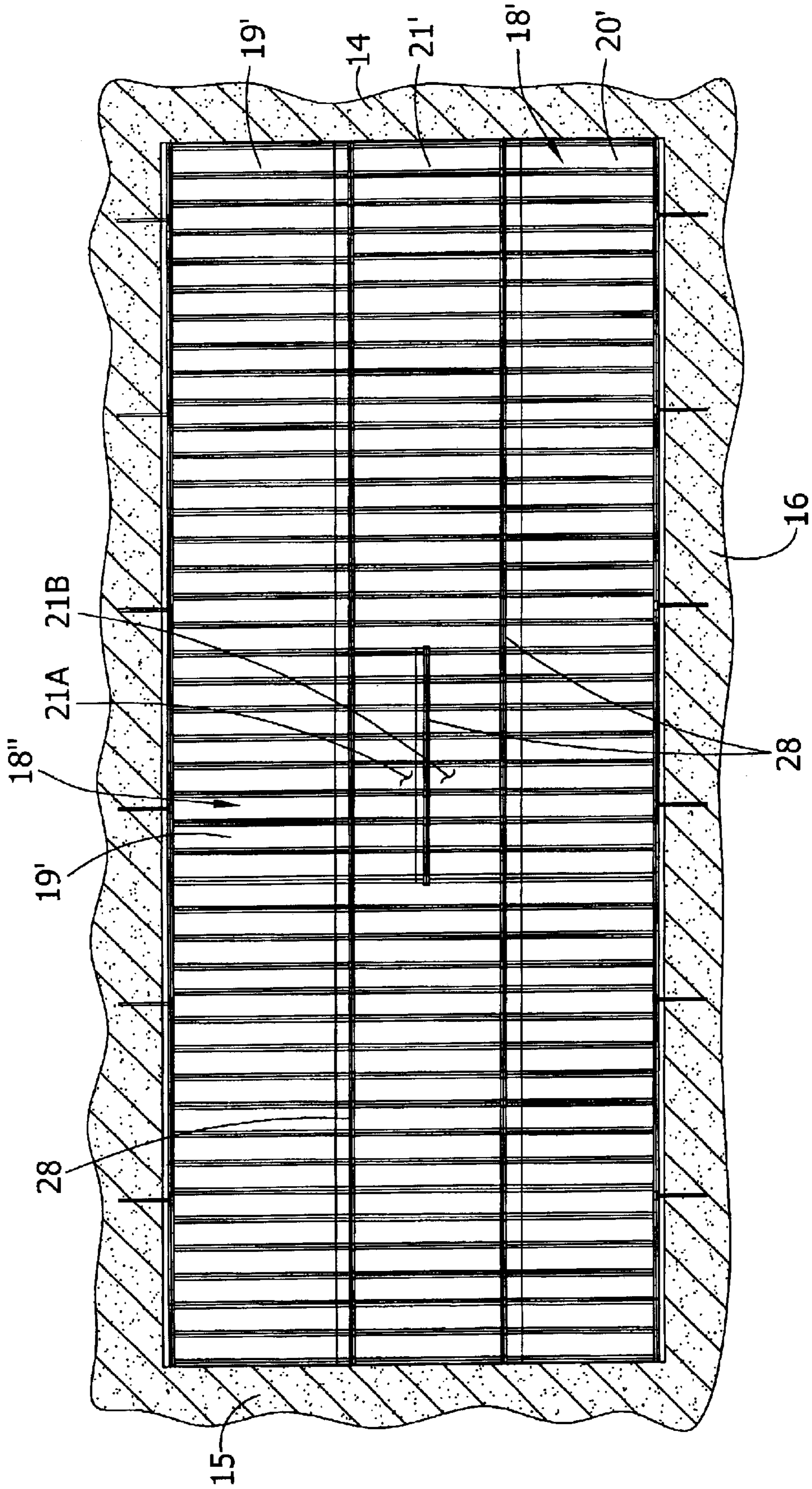
FIG. 11A
