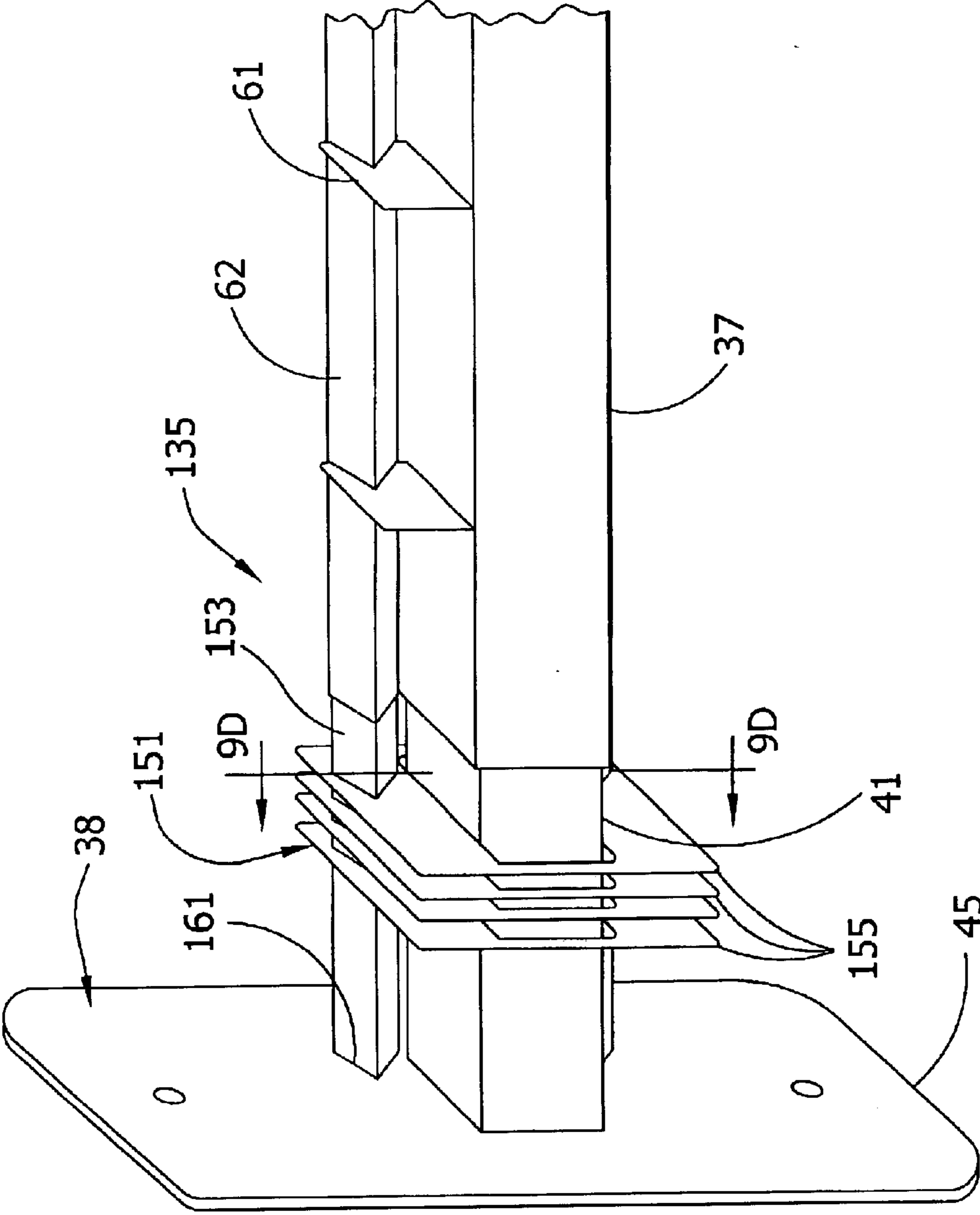
FIG. 9A
