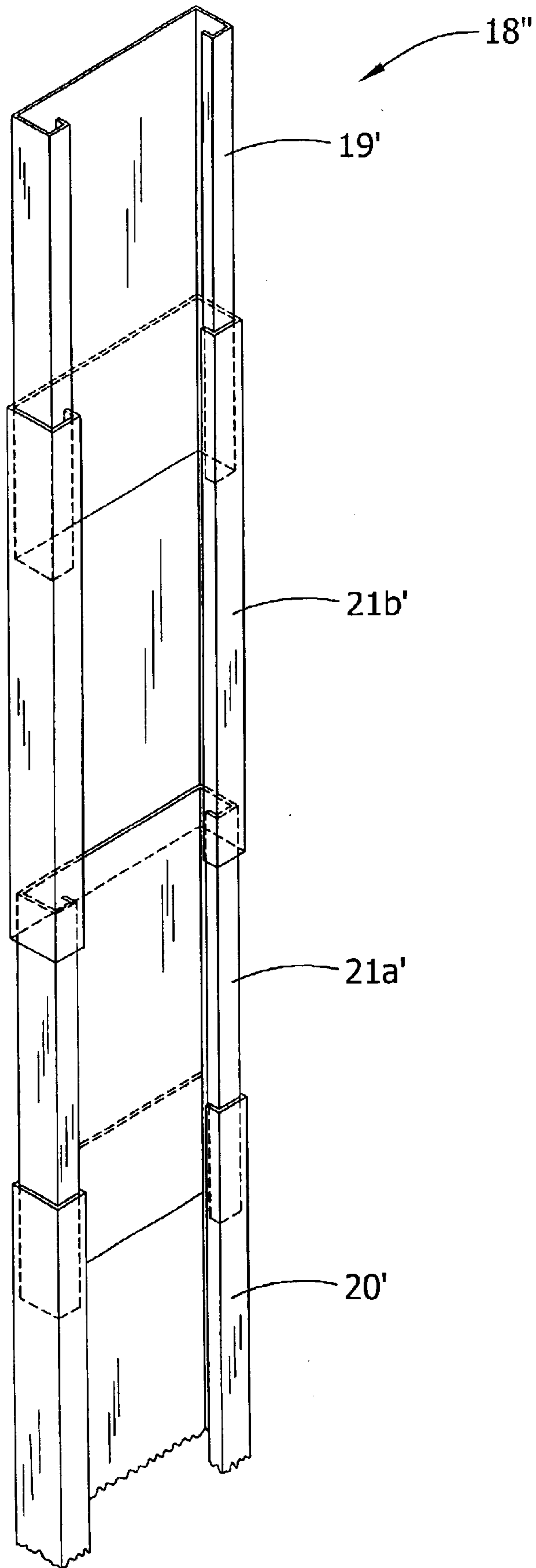
FIG. 12
