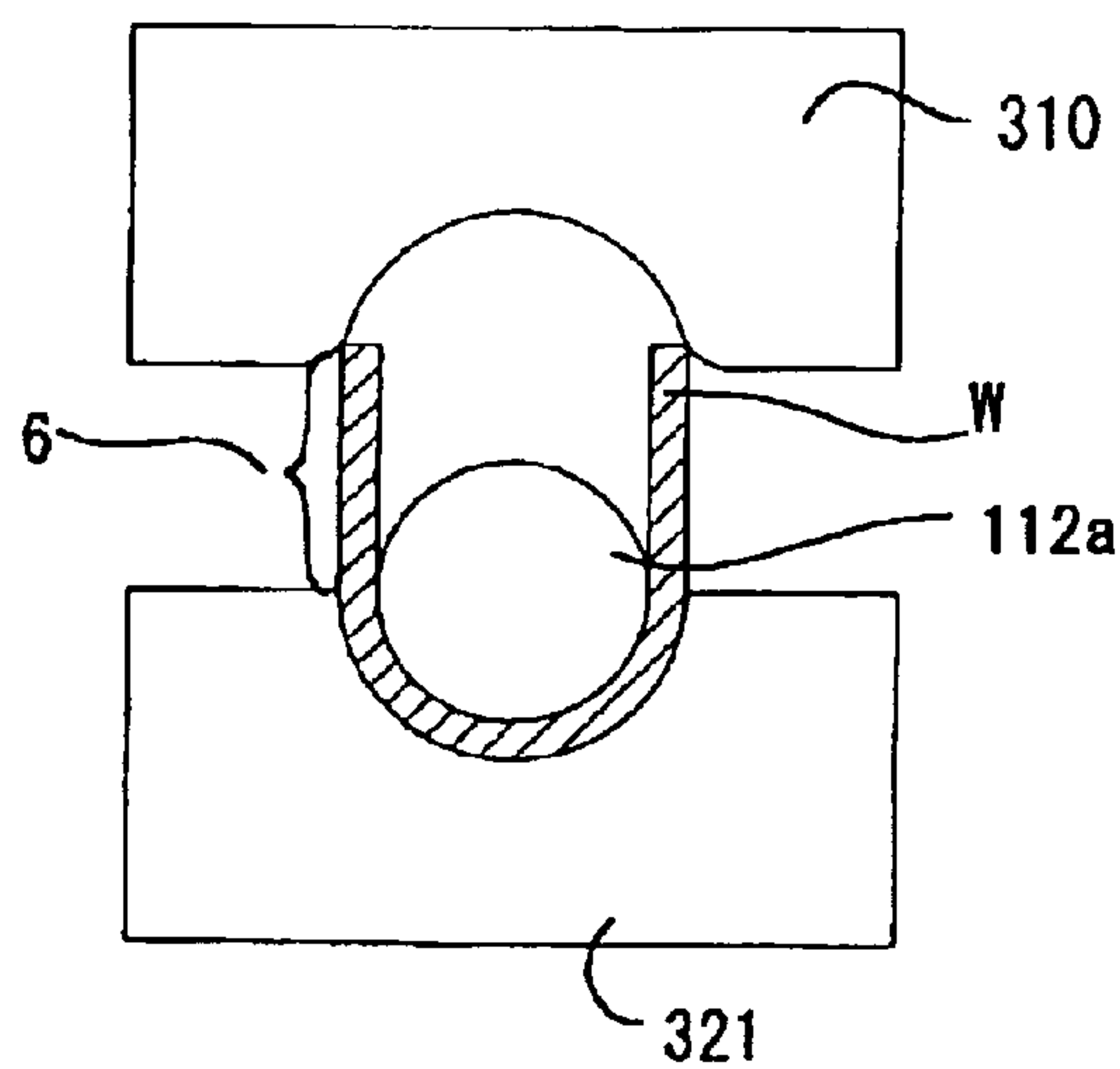
Fig.20c
