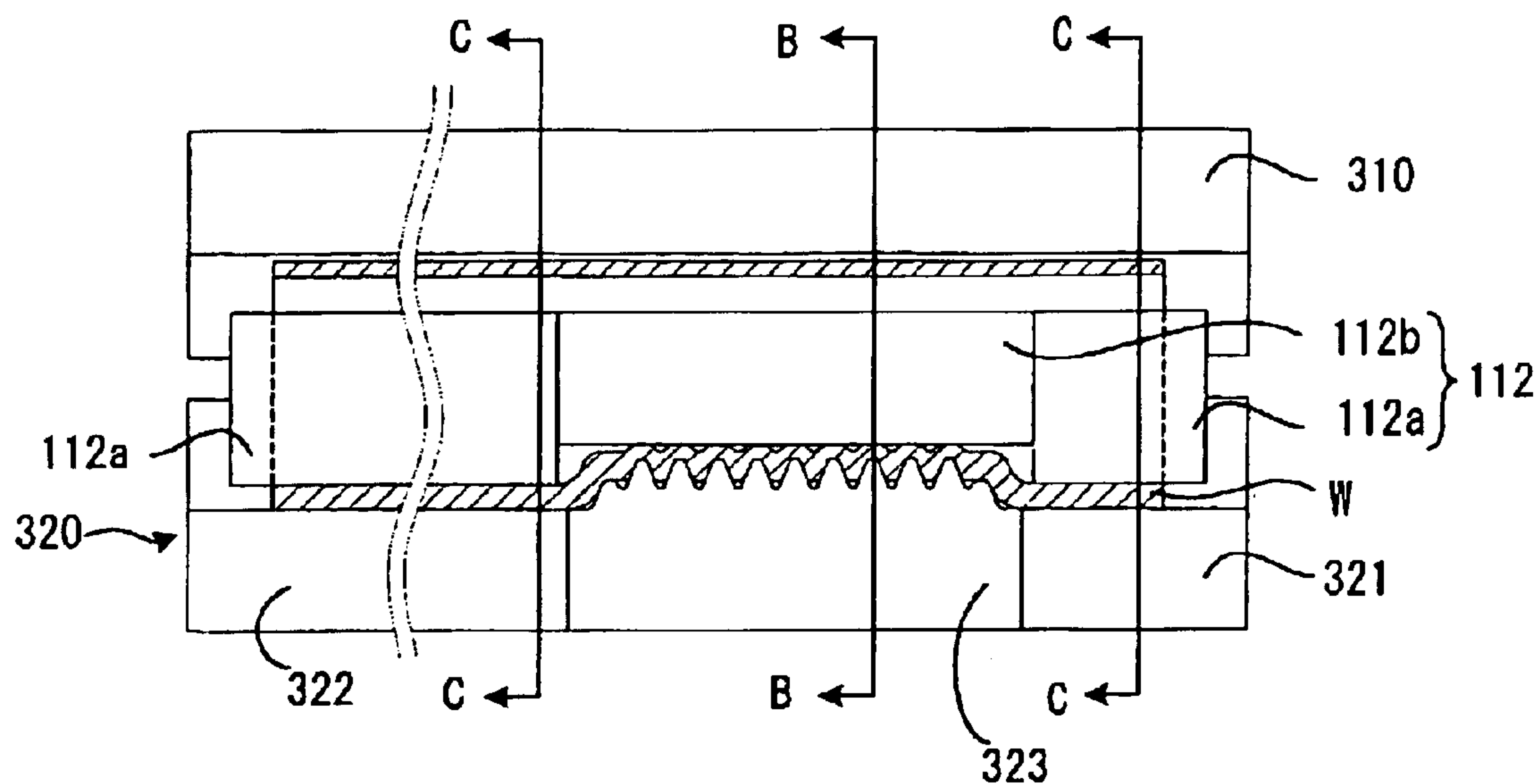
Fig.21a
