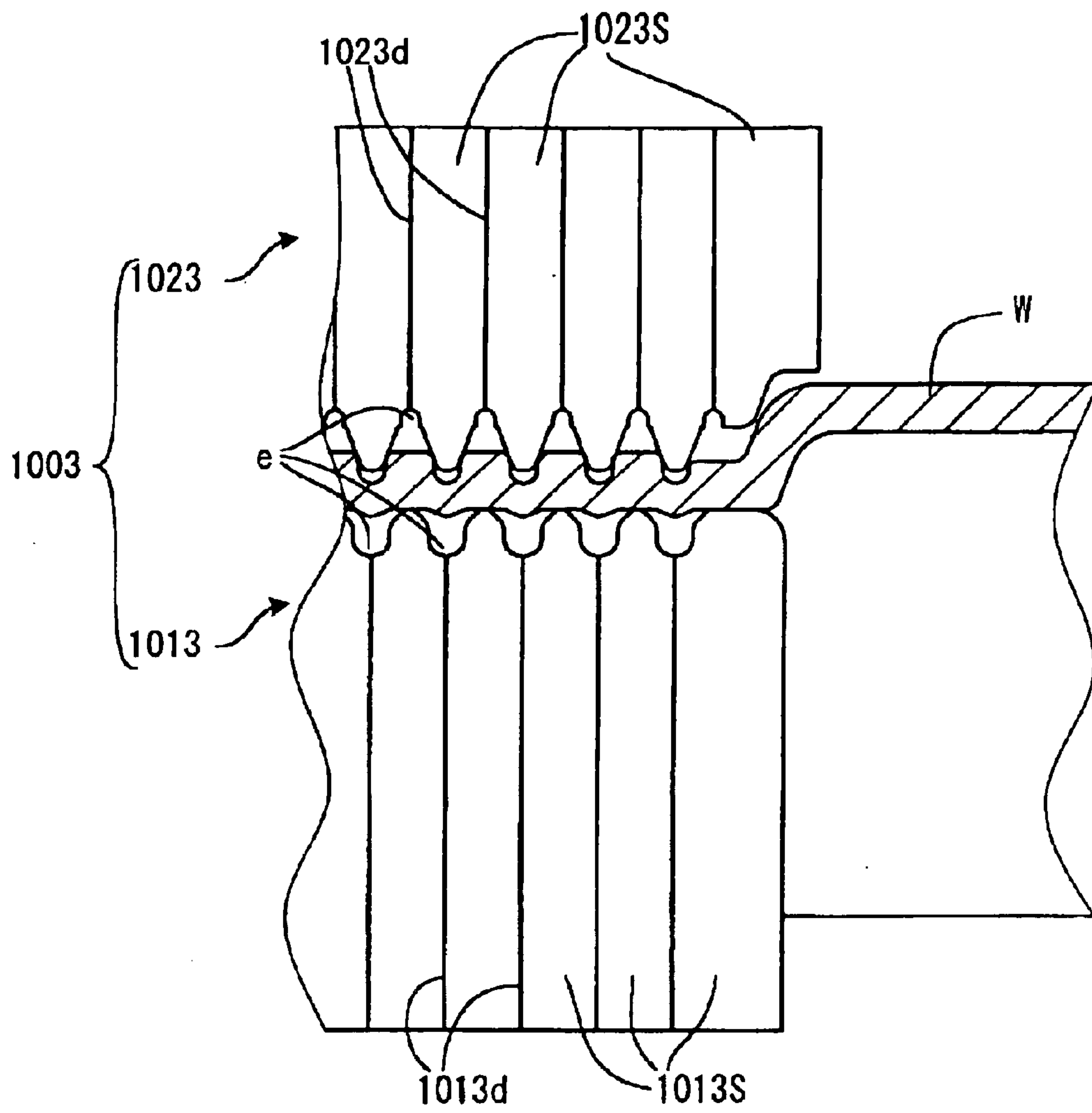
Fig. 19
