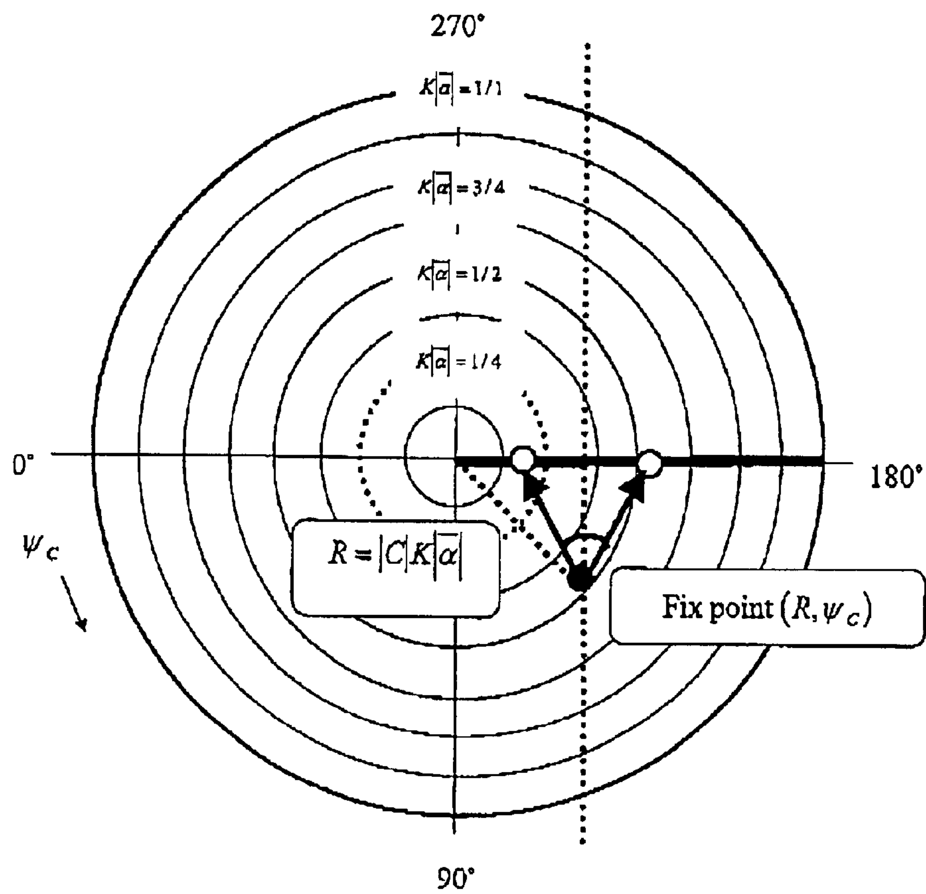
Fig. 9
