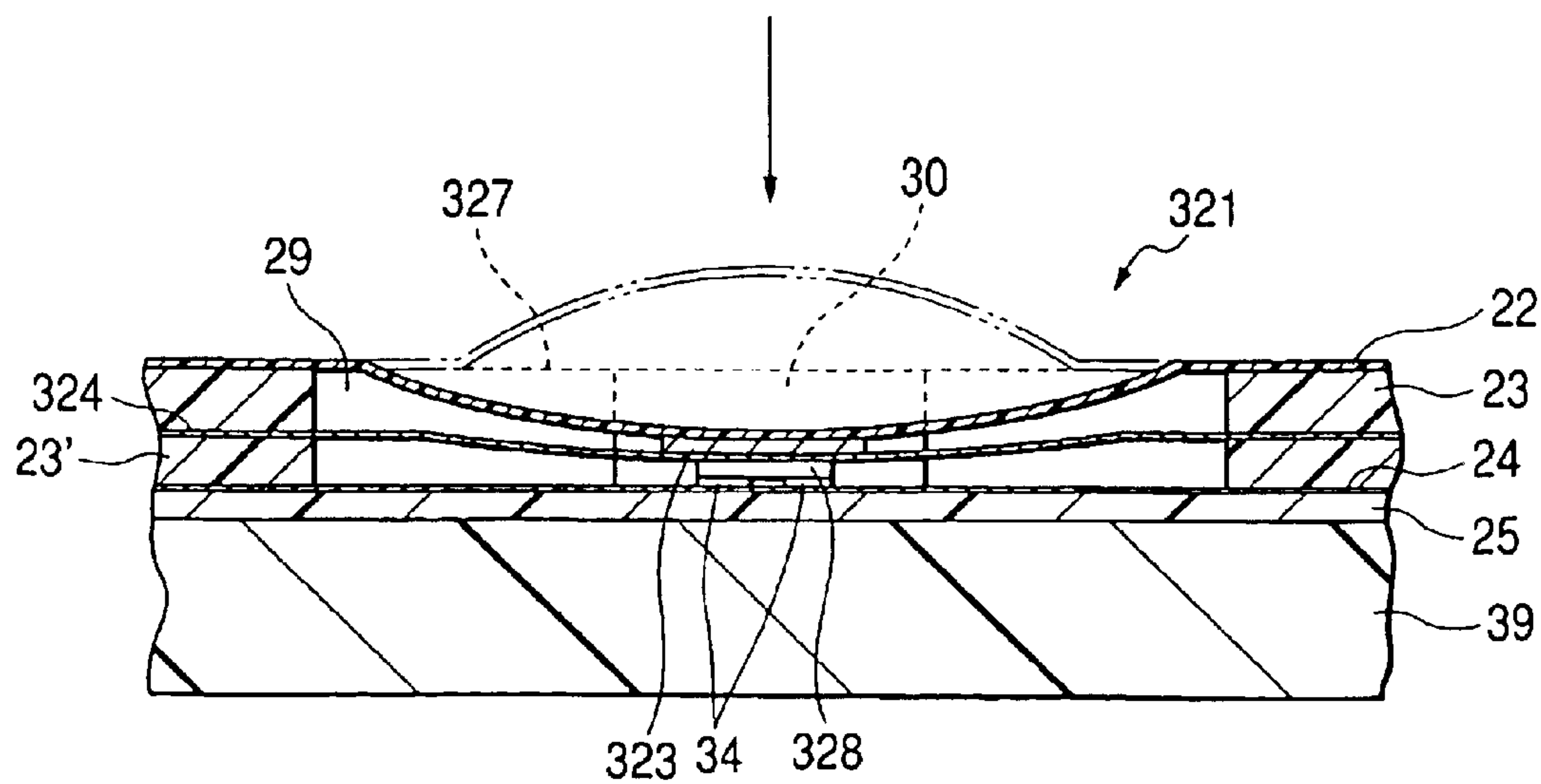
FIG. 34
