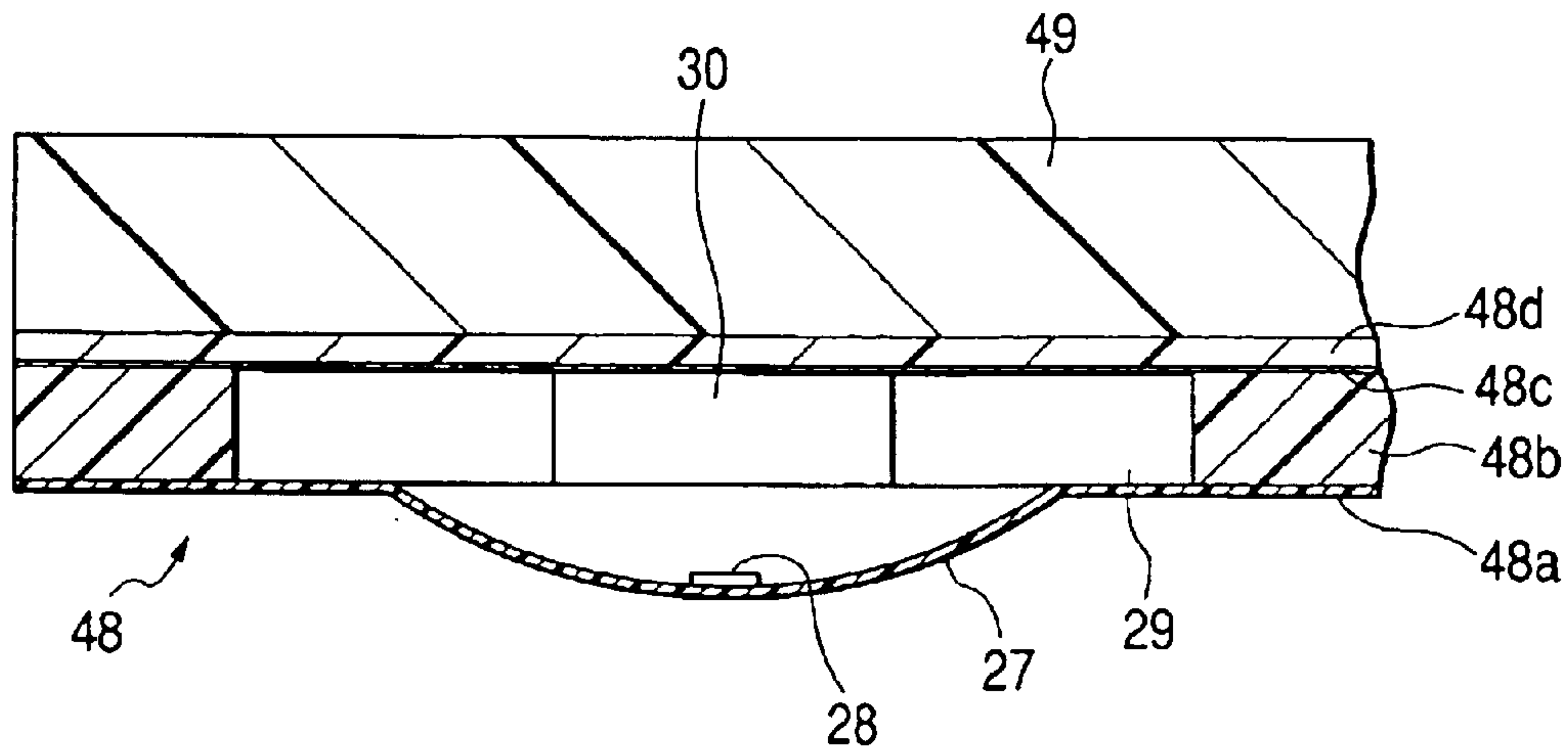
FIG. 21A
