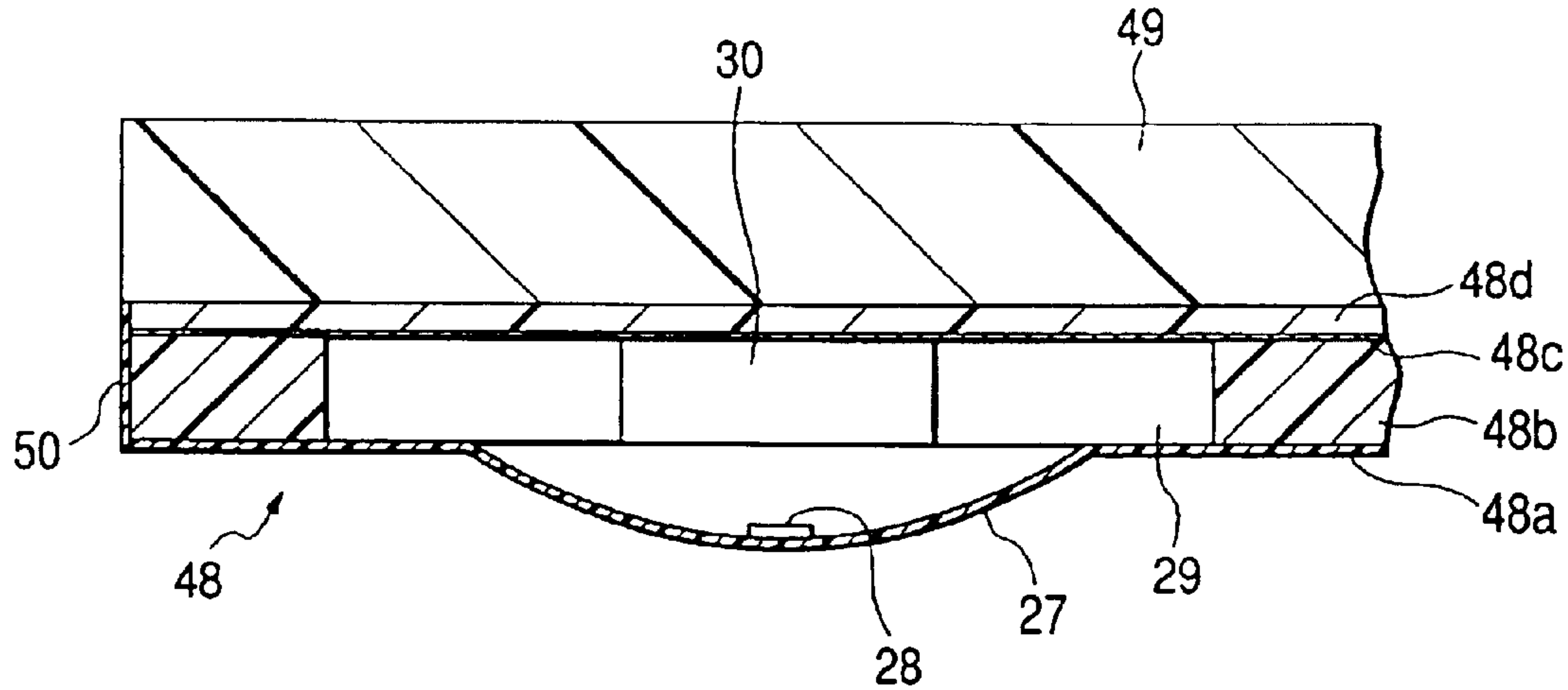
FIG. 21B
