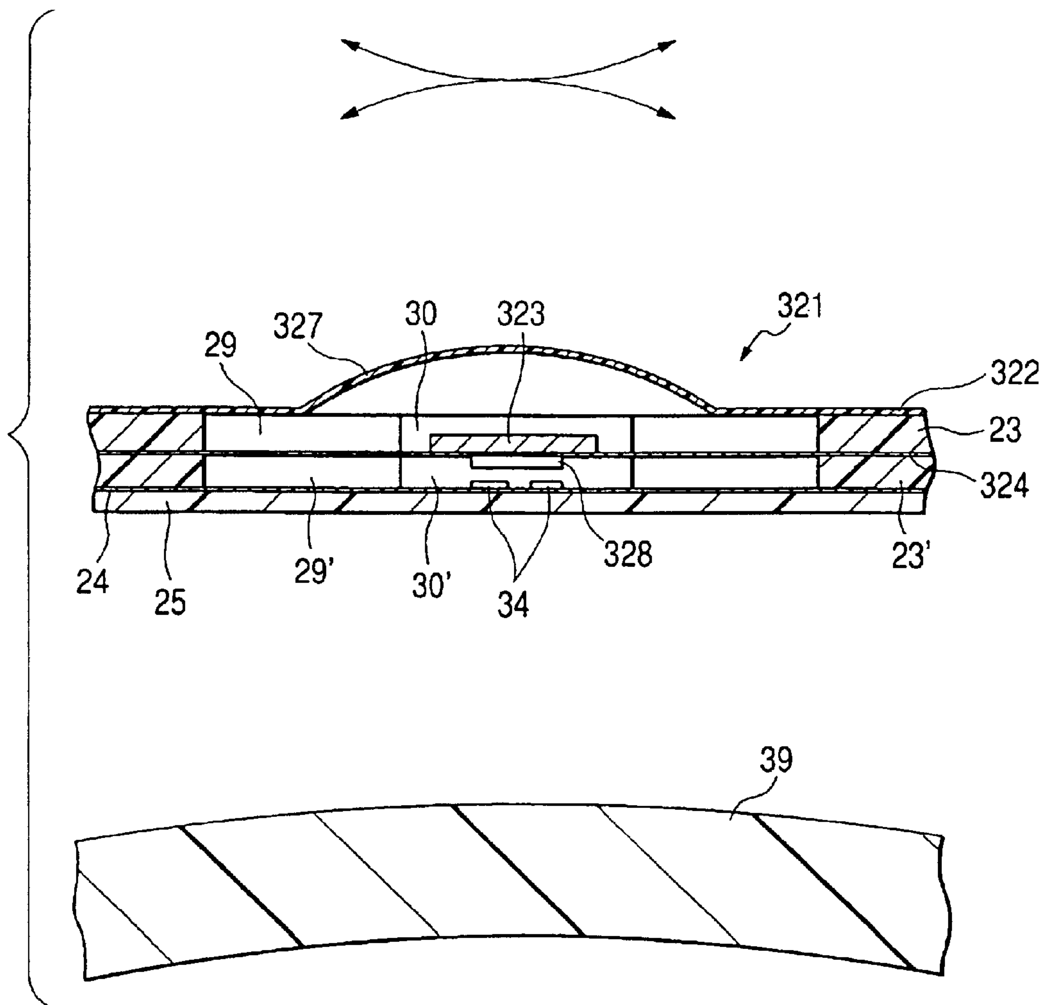
FIG. 34
