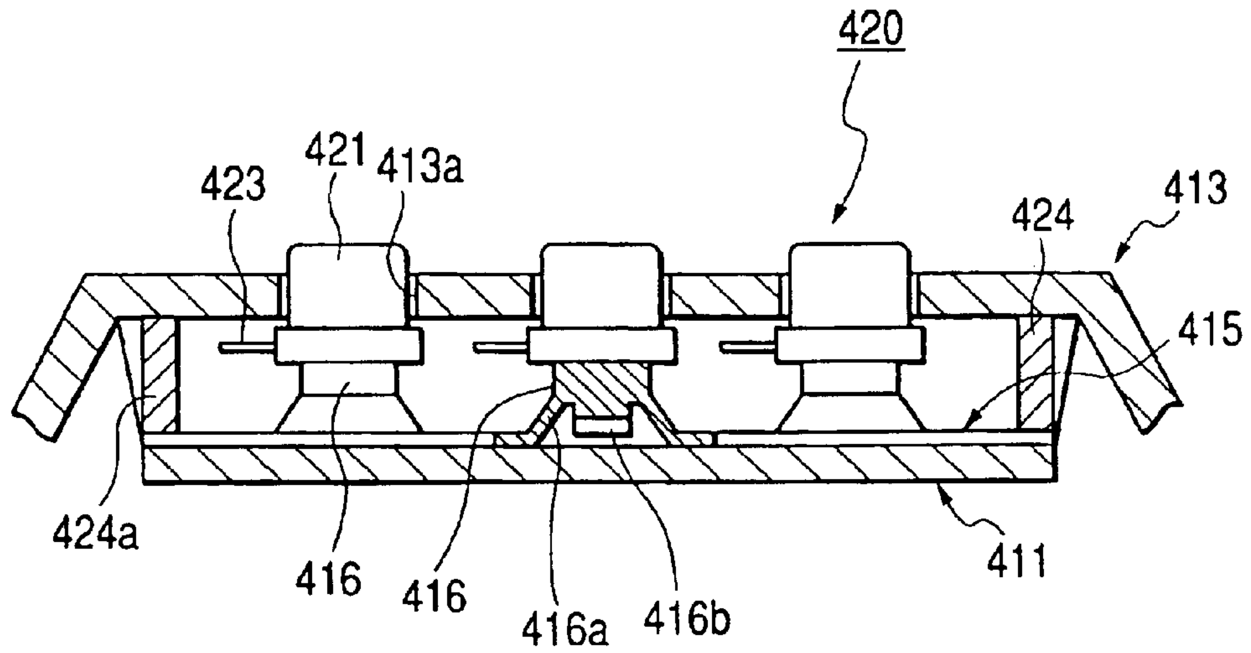
FIG. 36
