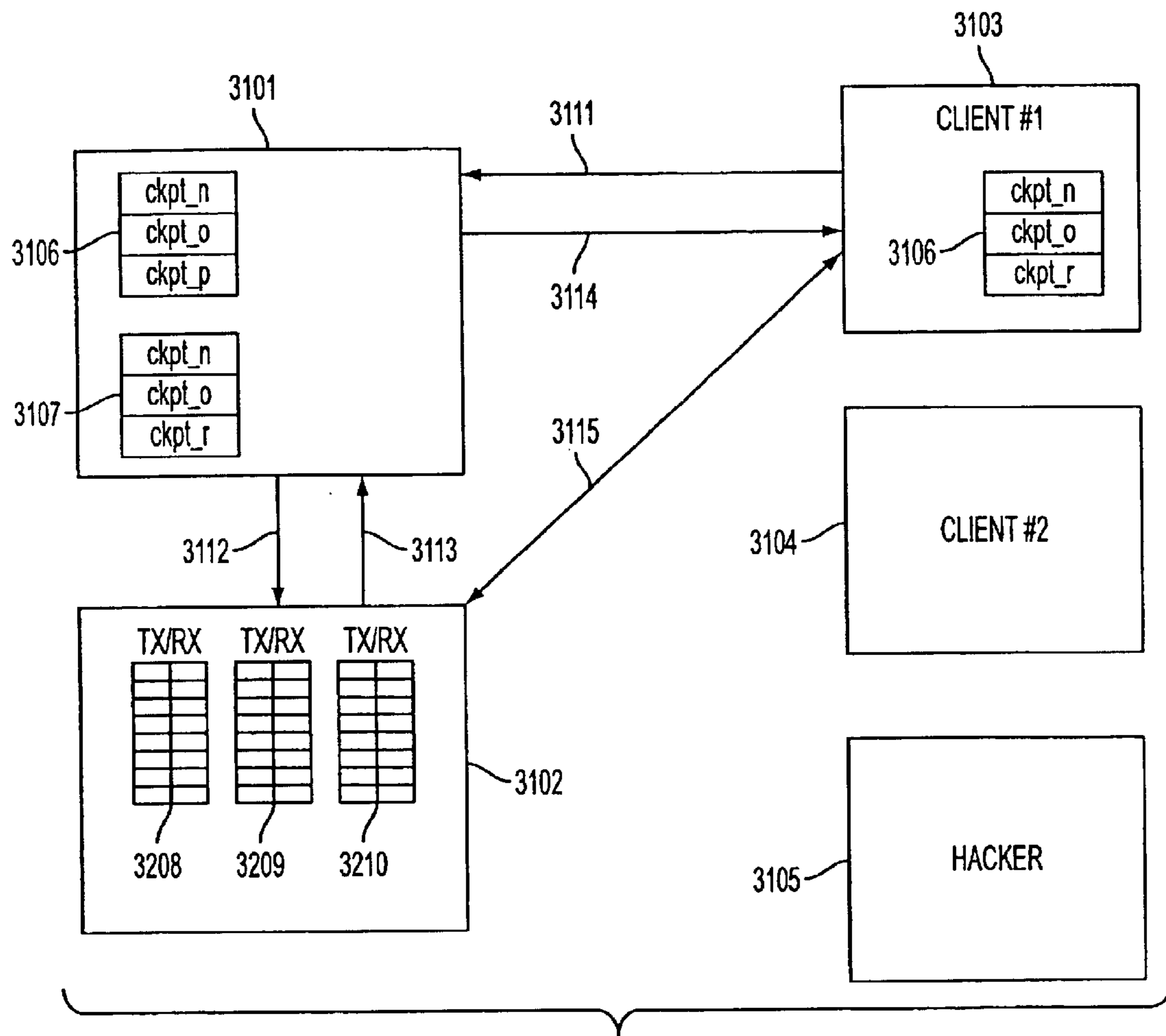
FIG. 31
