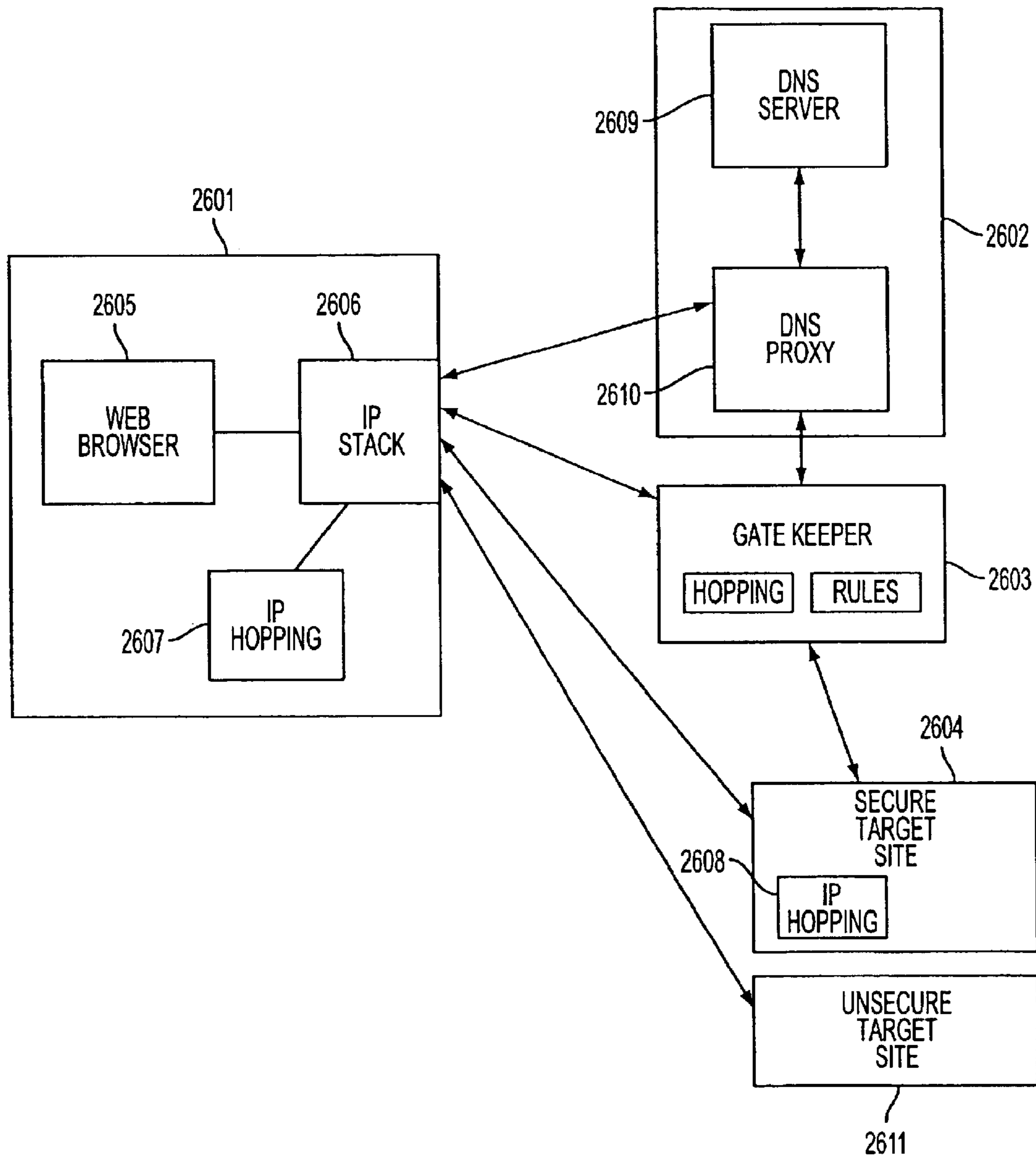
FIG. 26
