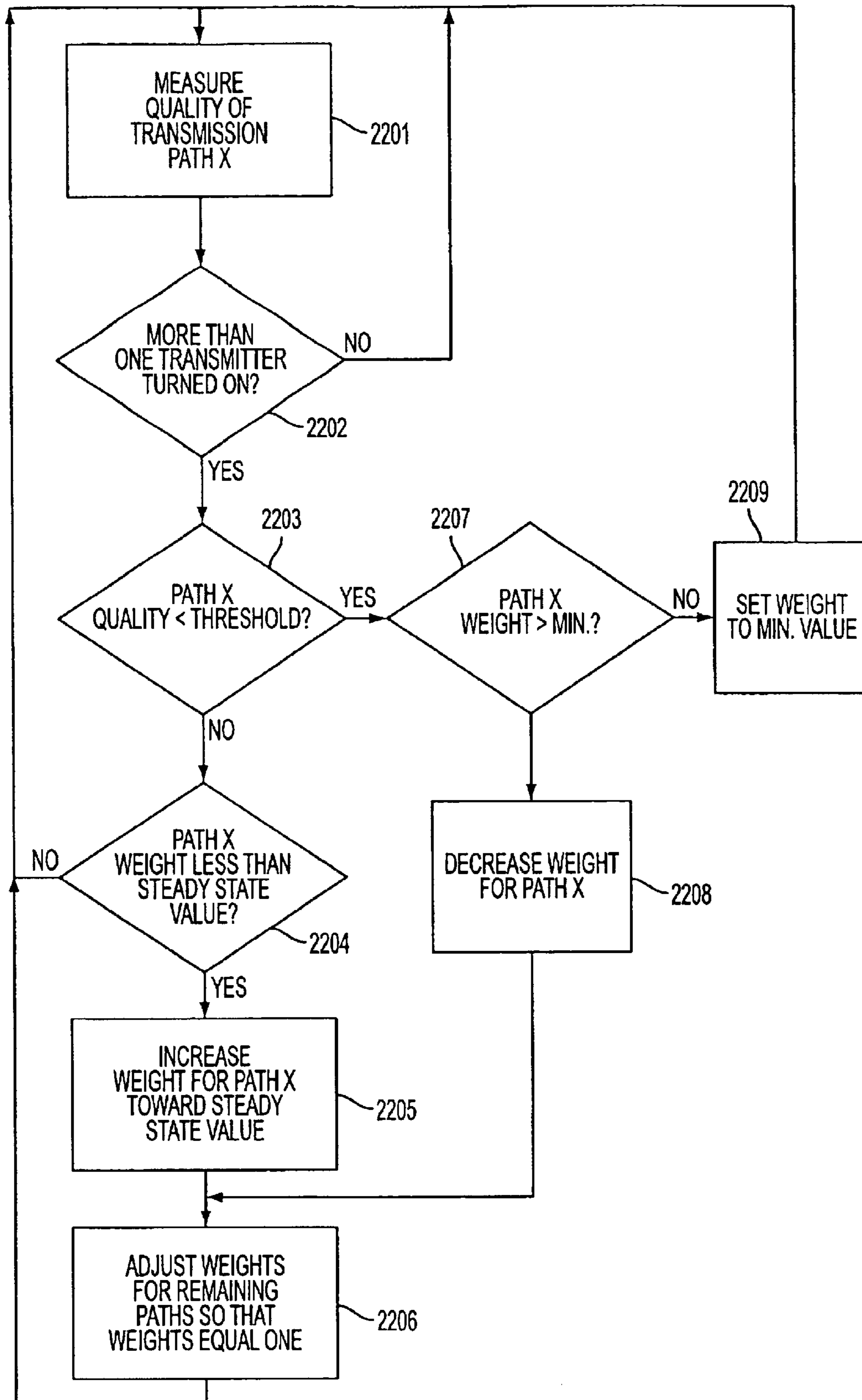
FIG. 22A
