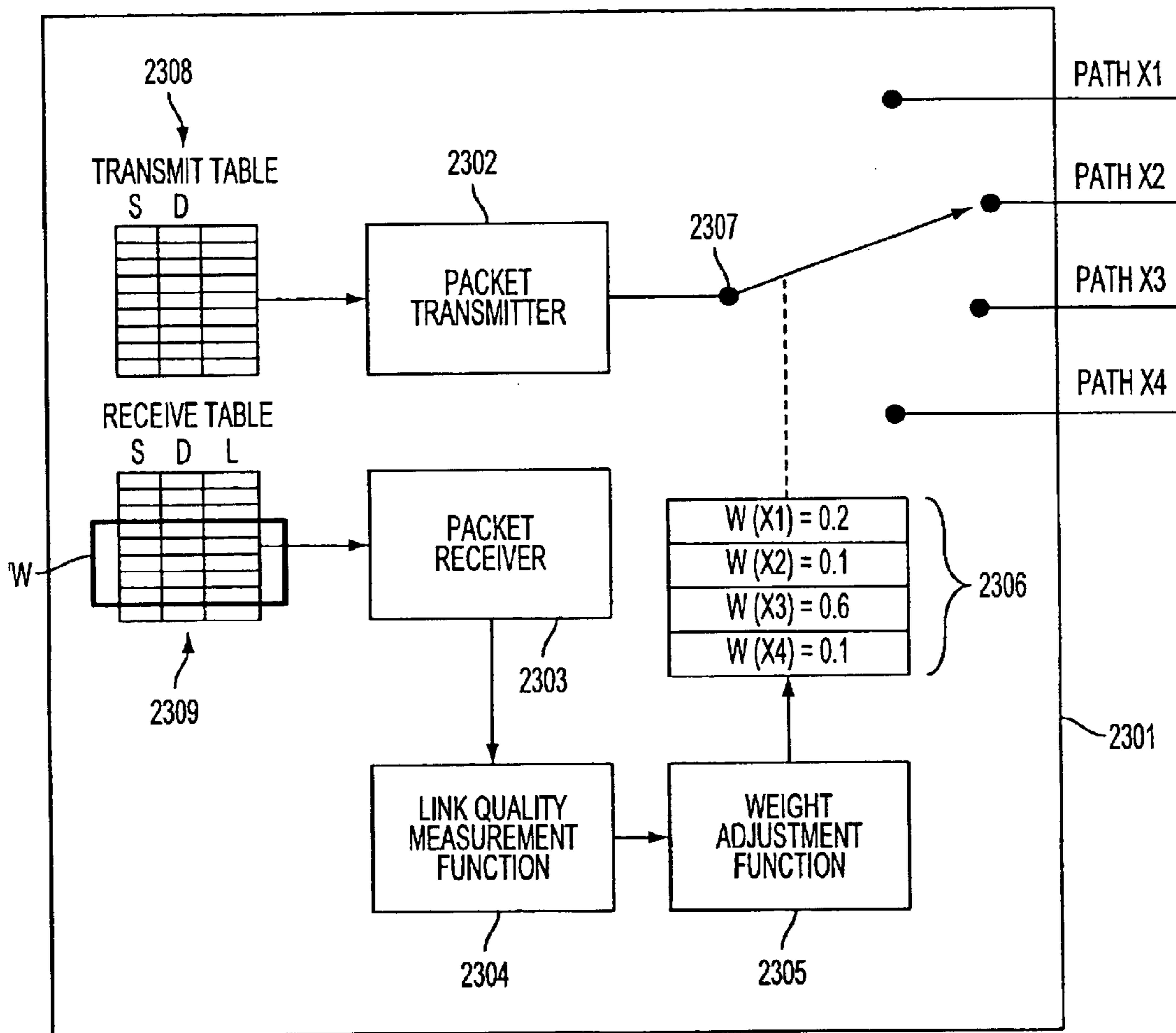
FIG. 23
