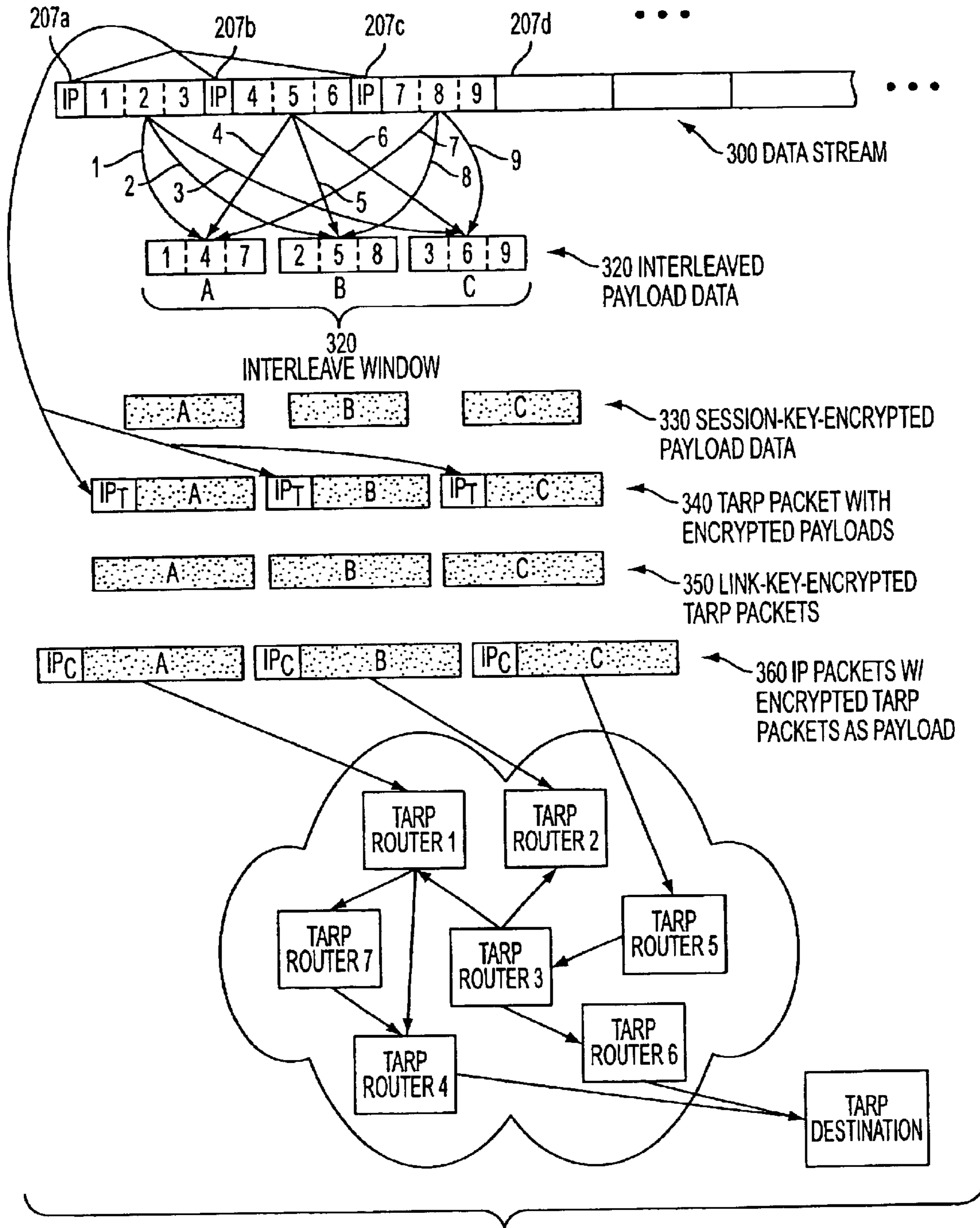
FIG. 3A
