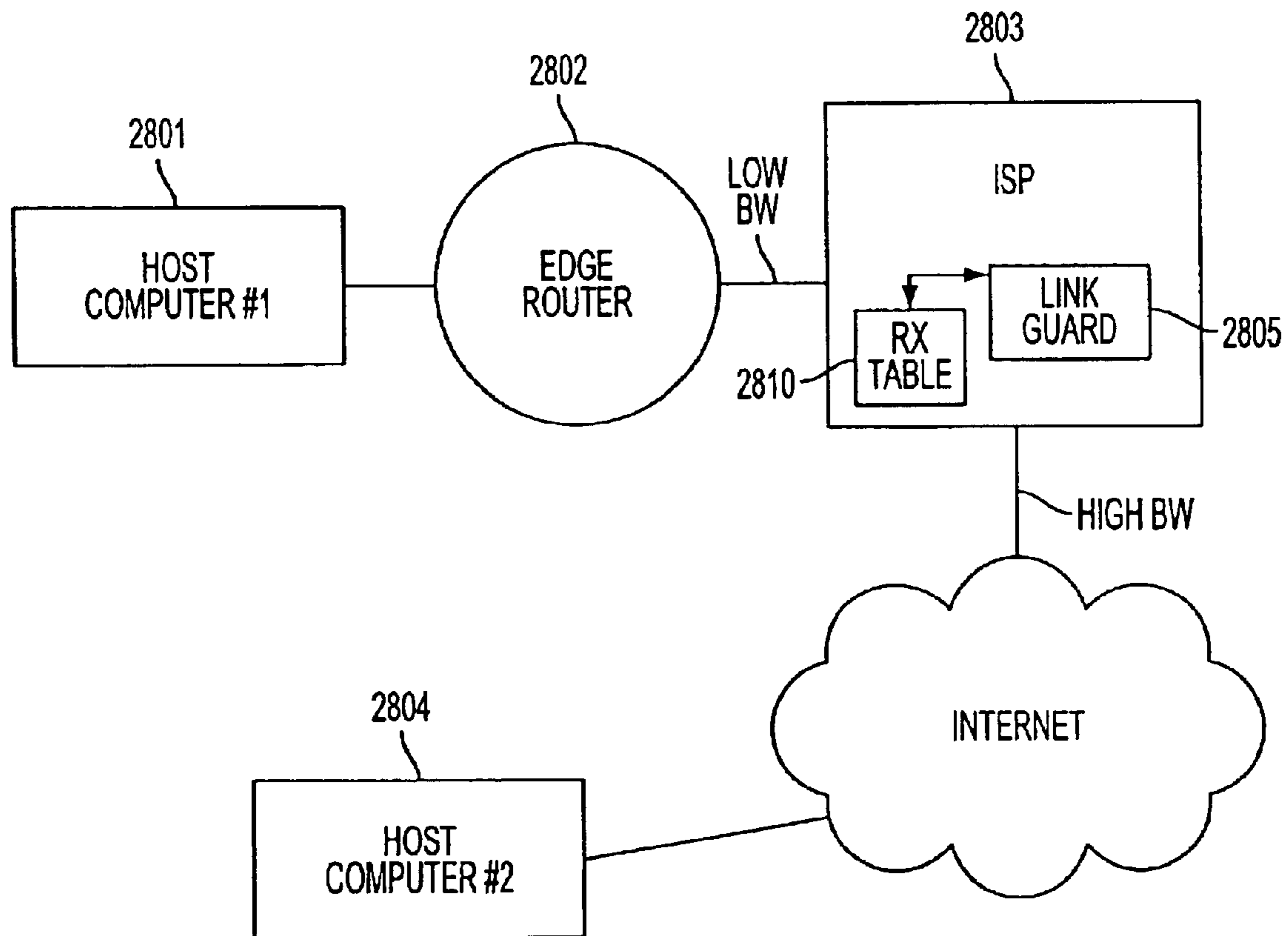
FIG. 28
