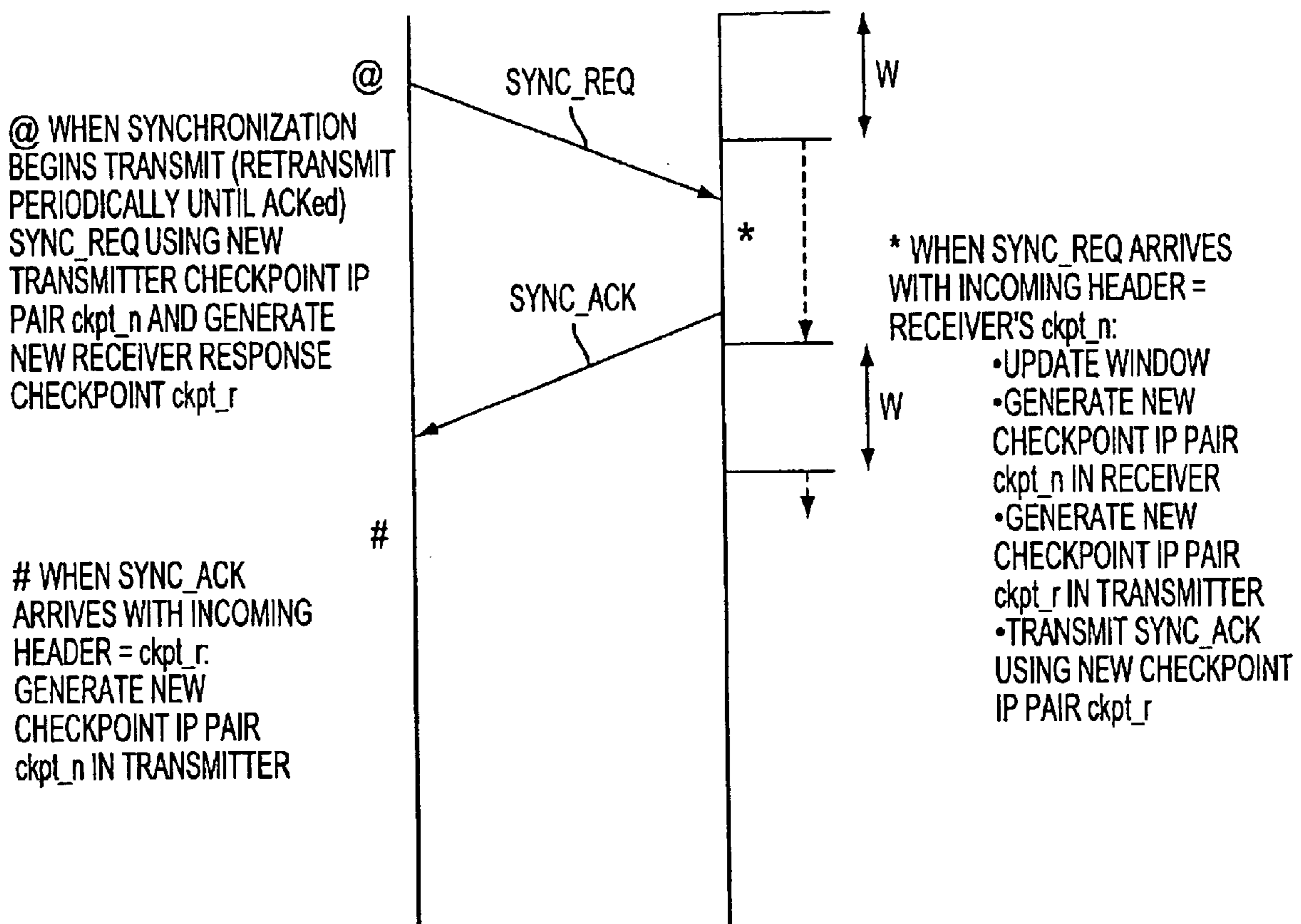
FIG. 15
