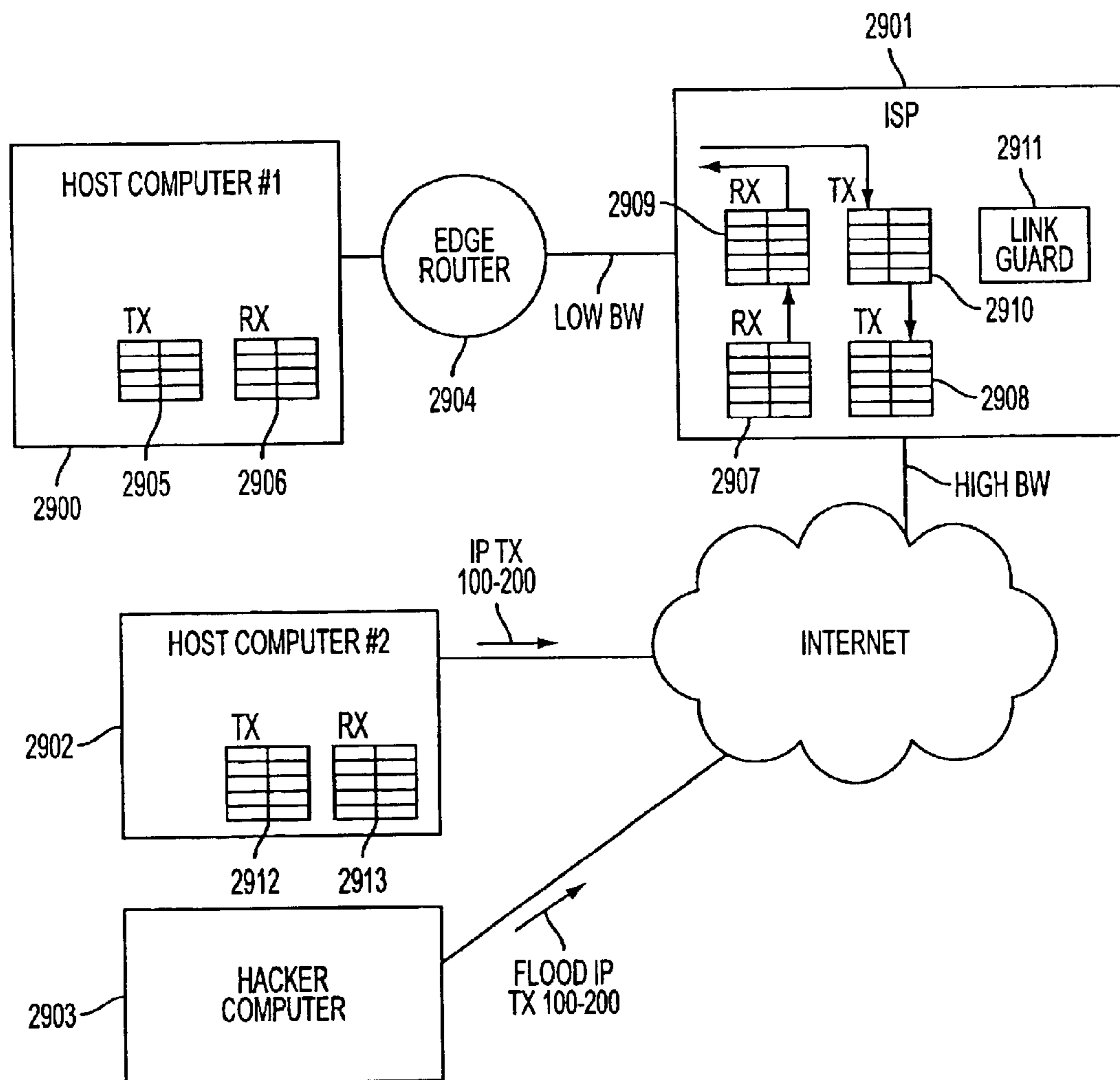
FIG. 29
