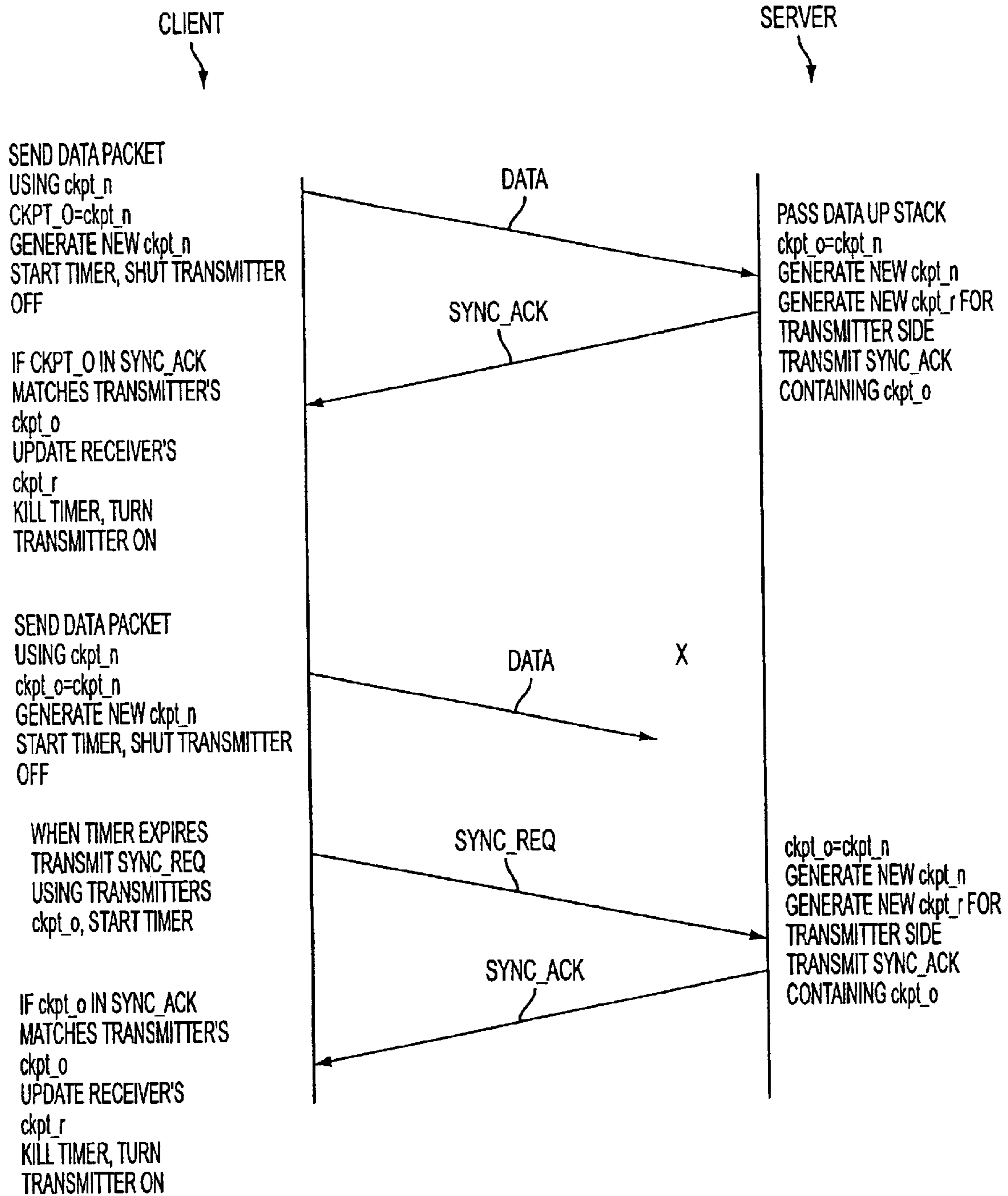
FIG. 32
