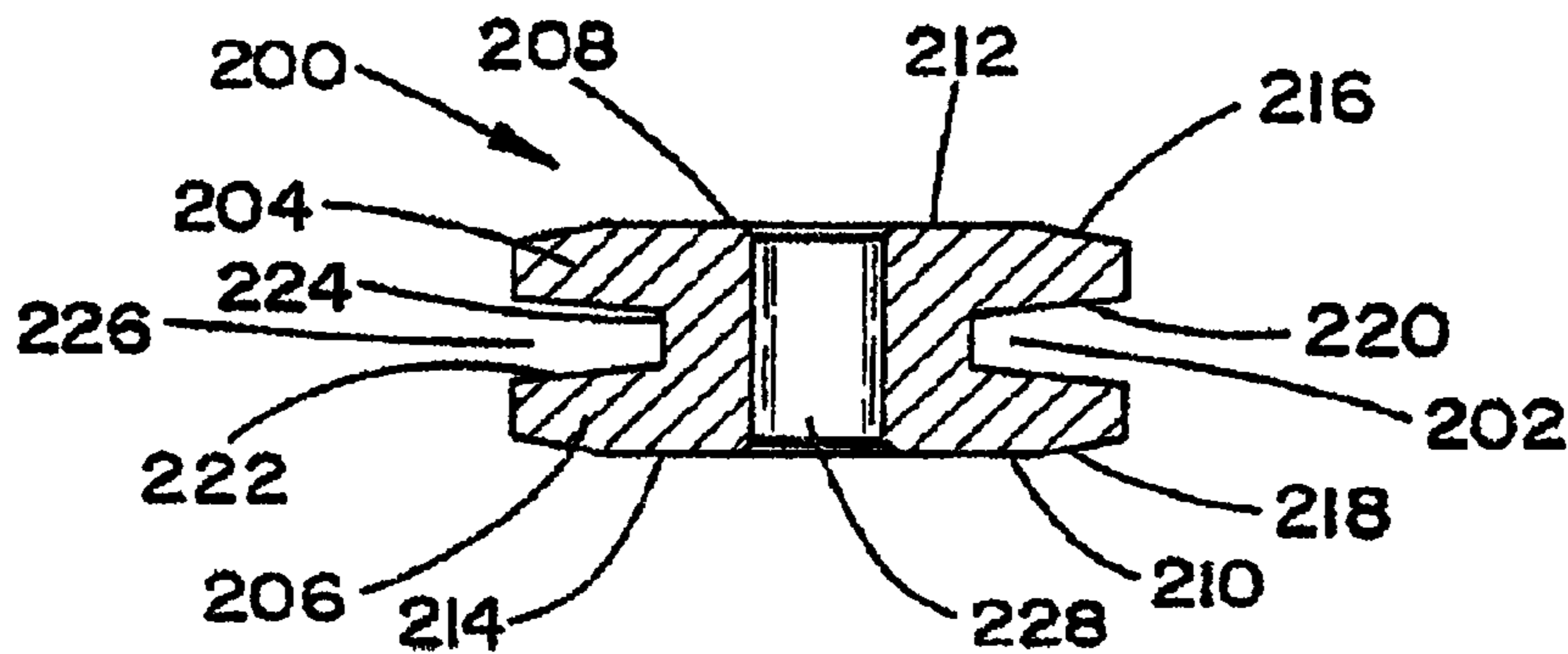
Section A-A
