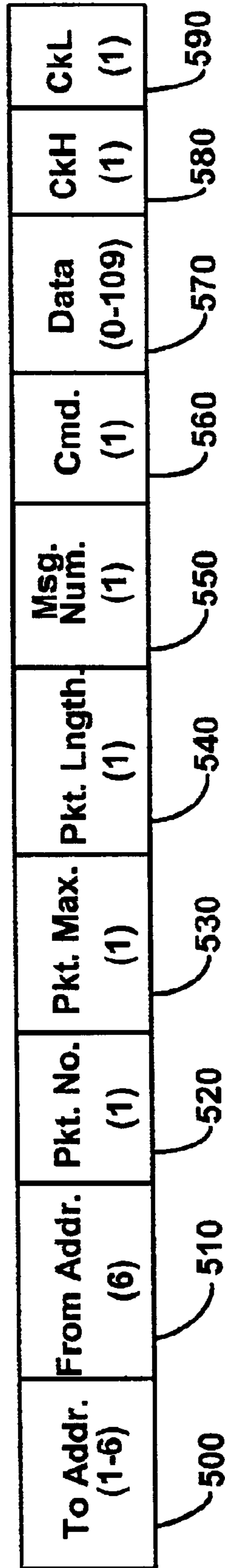
FIG. 5 Message Structure
