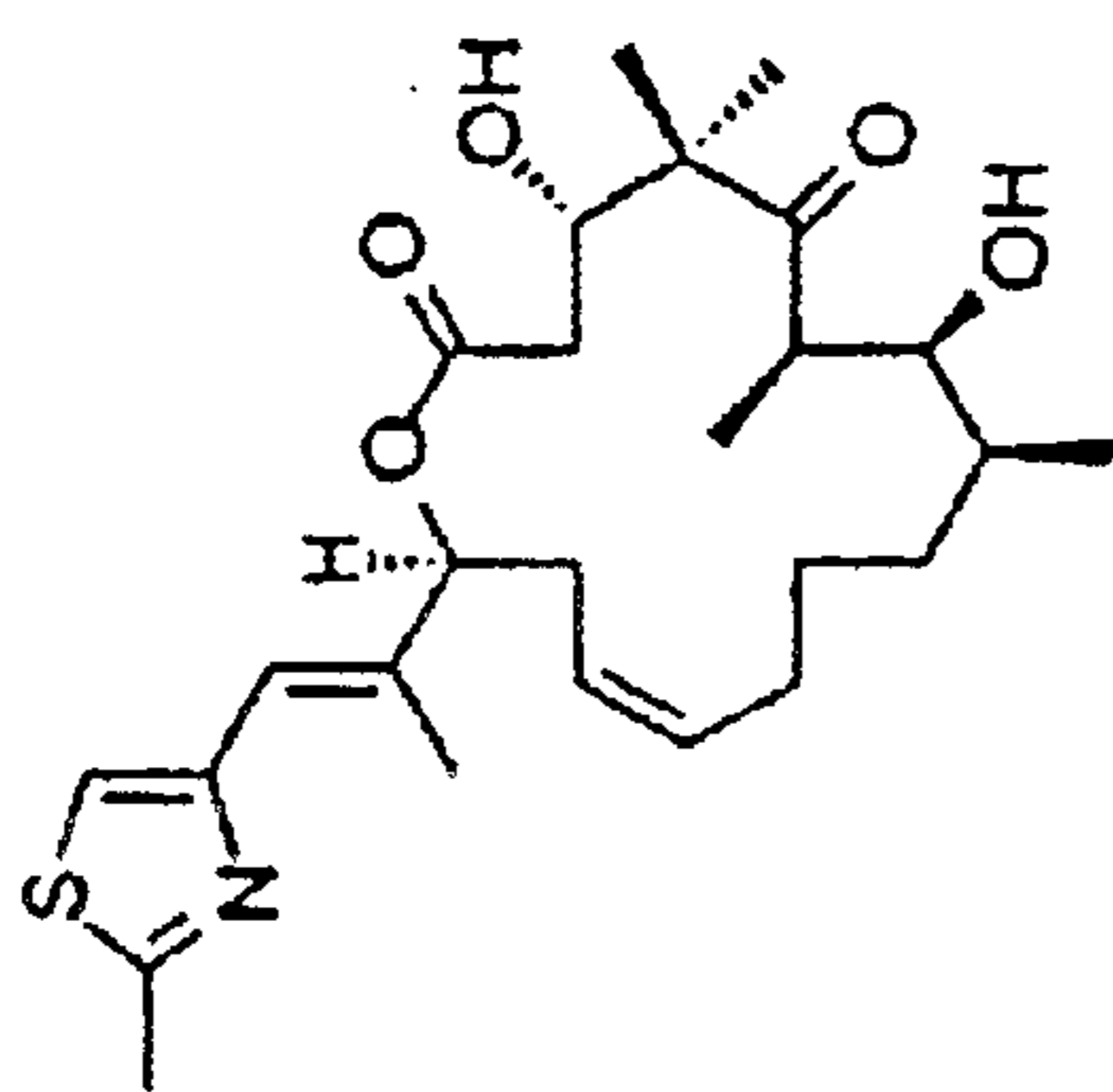
desoxyepothilone A
