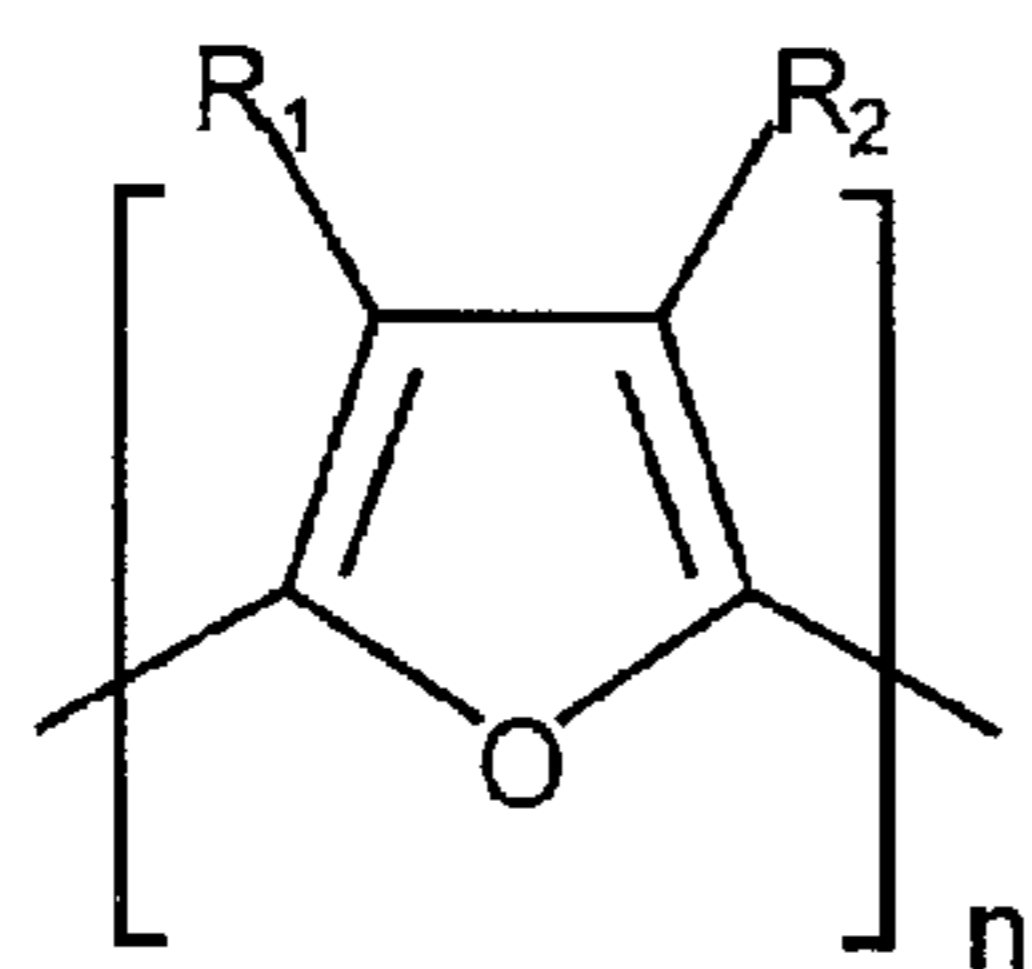
Polyfuran
