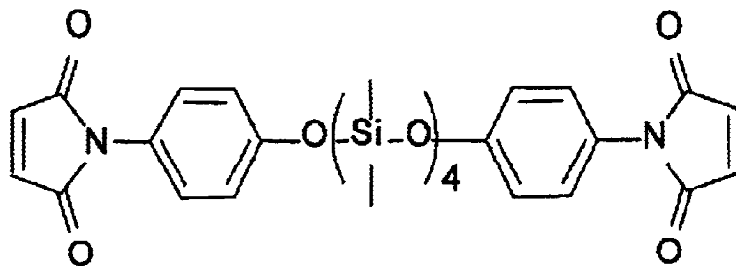
((C_4H_2O_2N)C_6H_4)_2(OSi(CH_3)_2)_4O
