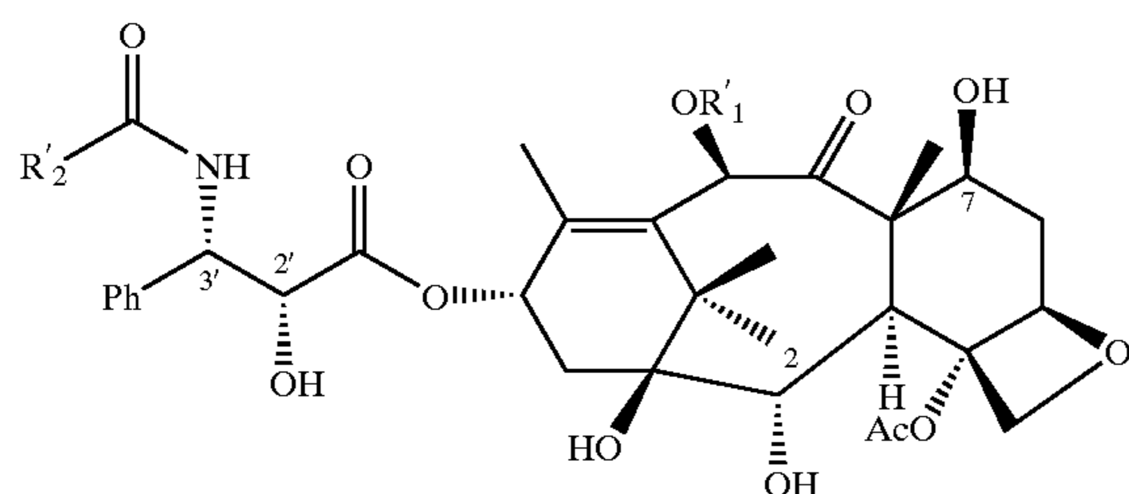
Paclitaxel: R_1 = C_6H_5 ; R_2 = CH_3C(=O) ; Taxotere: R_1 = (CH_3)_3C(=O) ; R_2 = H
