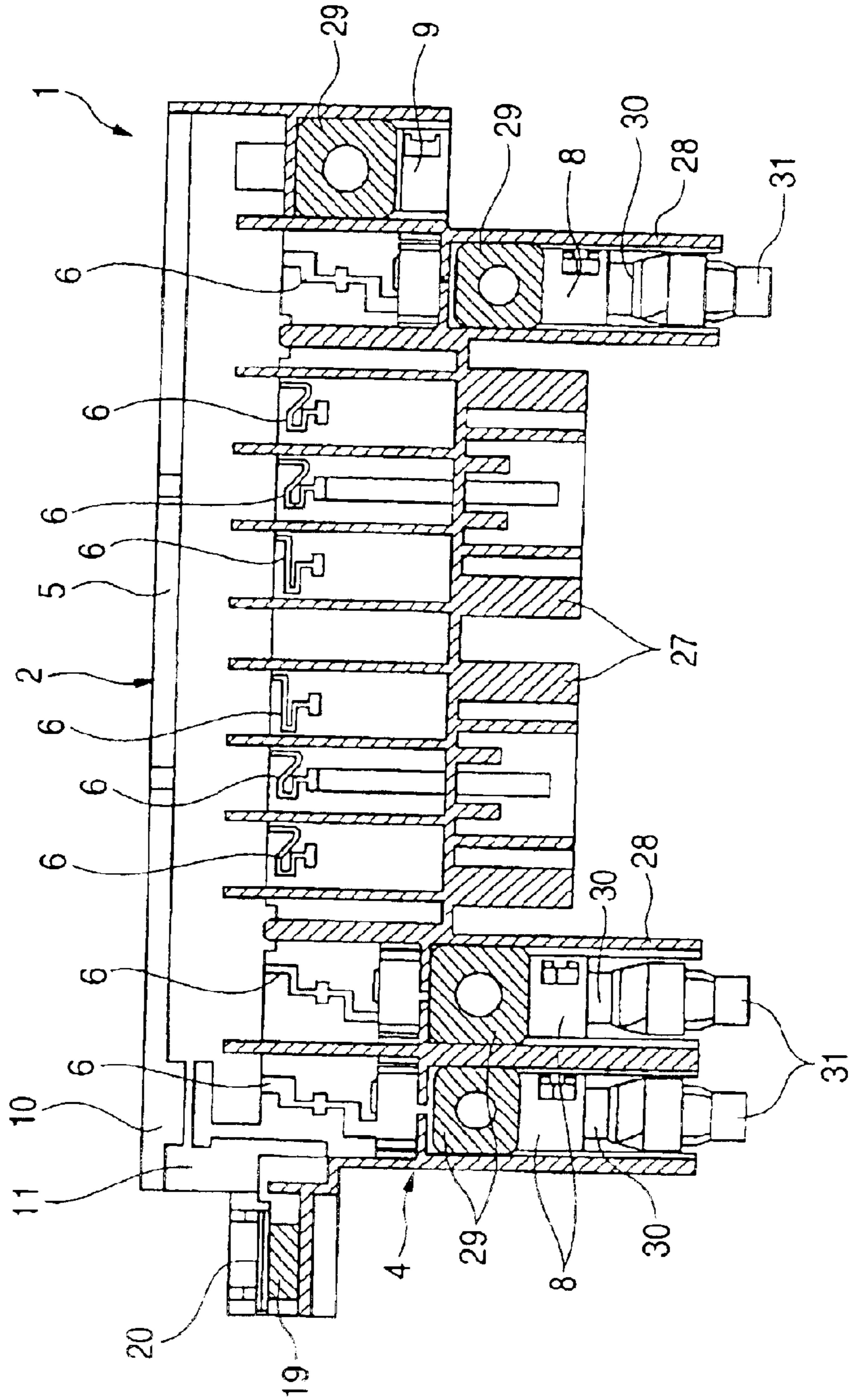
FIG. 6 B-B
