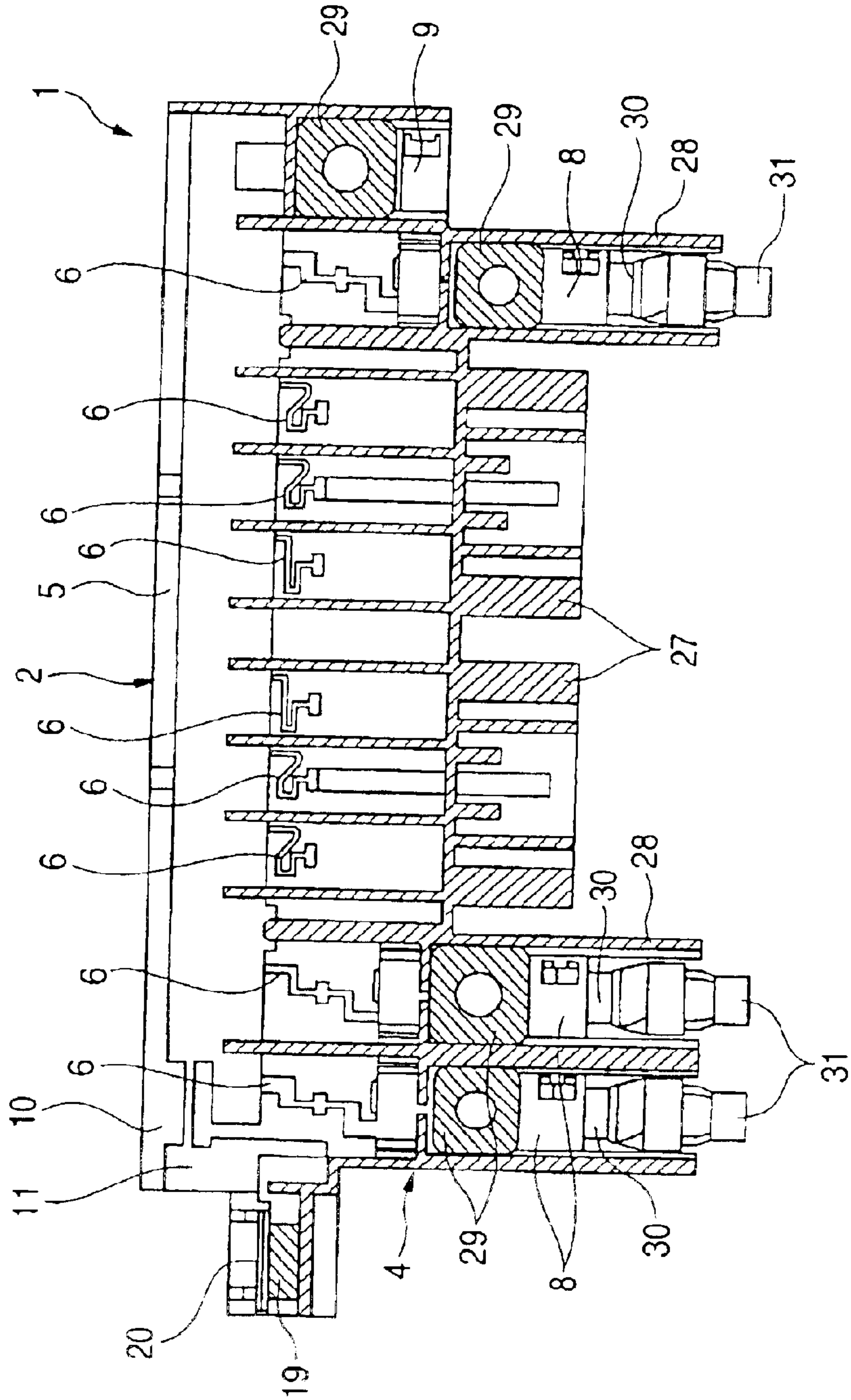
FIG. 6 B-B
