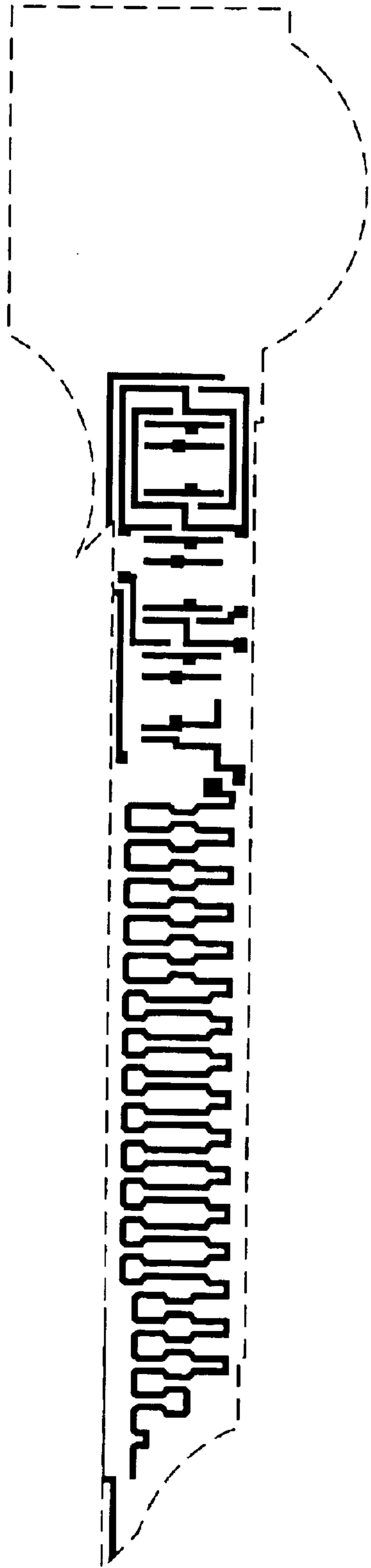
Poly mask
