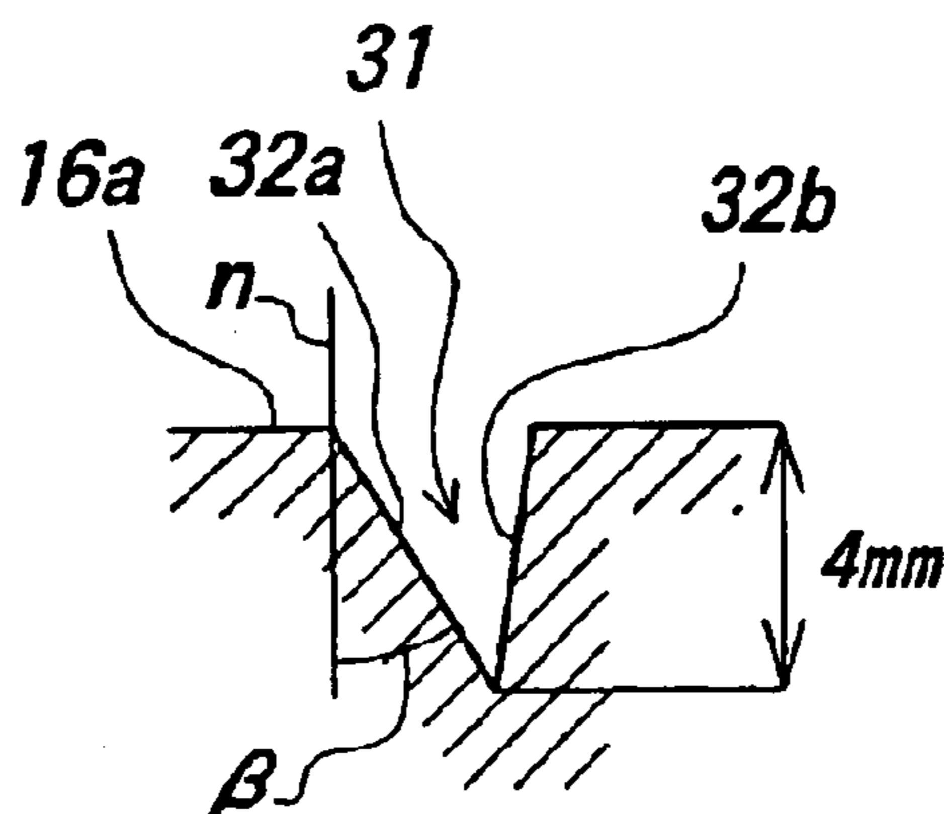
FIG. 10 IV-IV section
