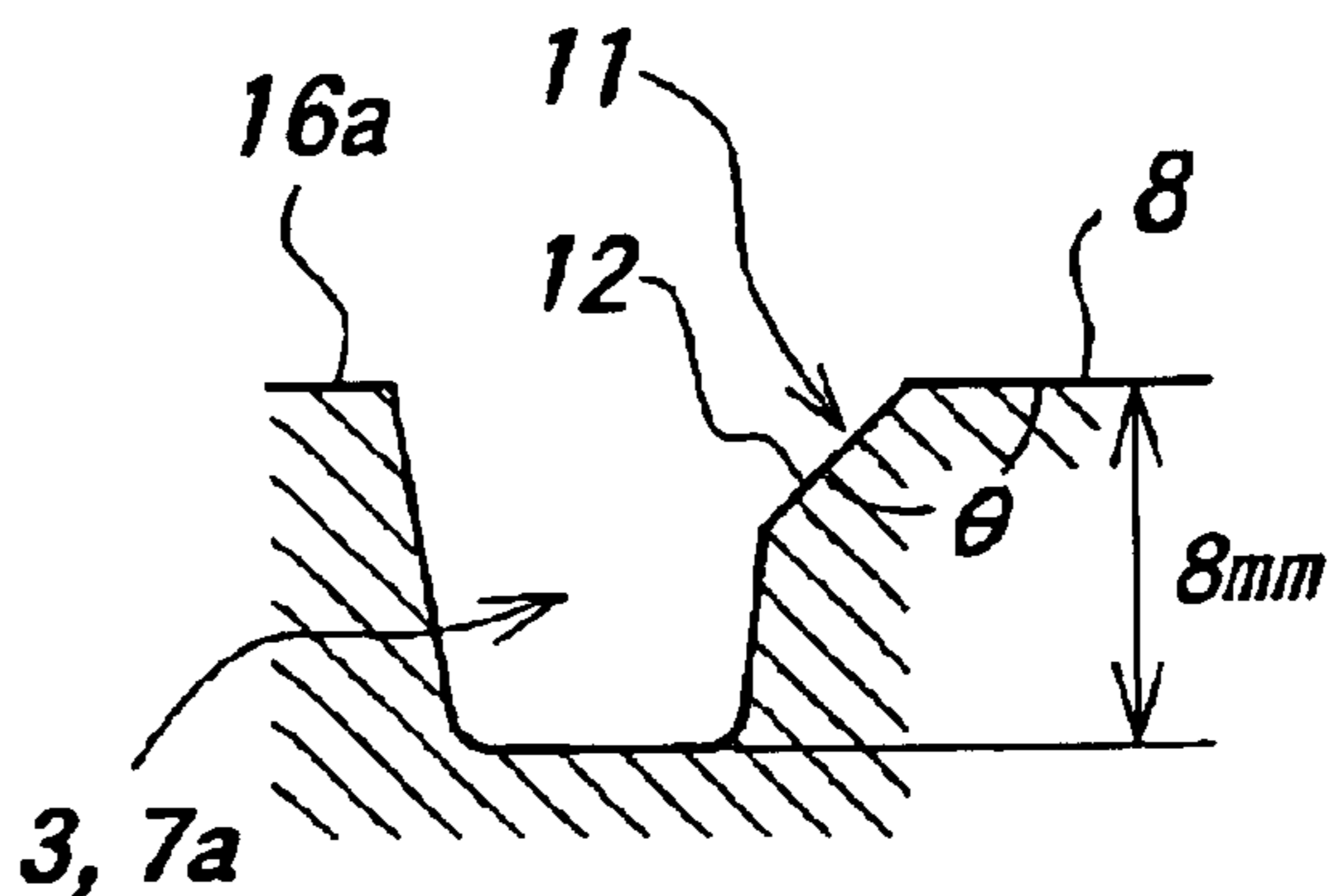
FIG. 9a I-I section
