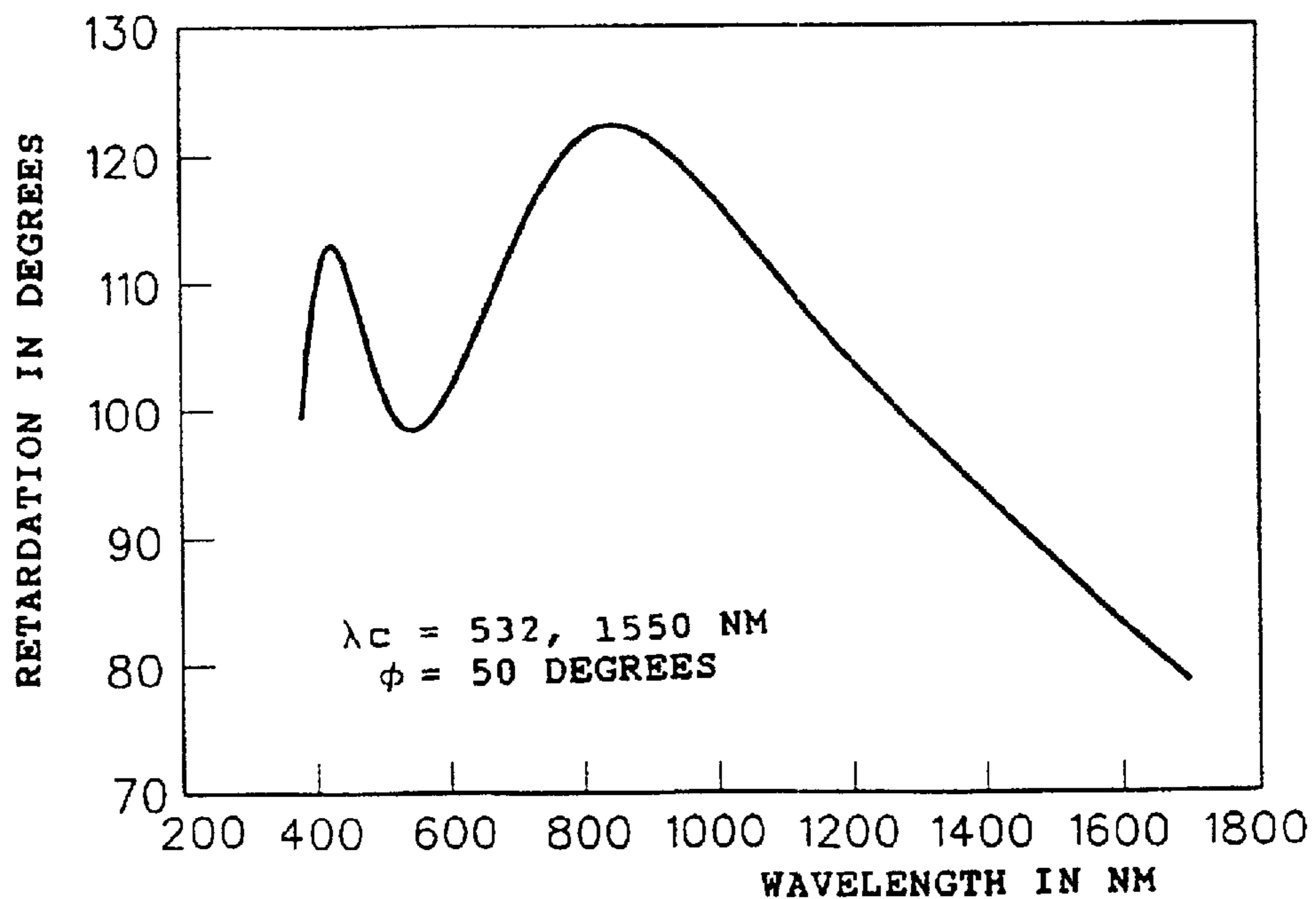
FIG. 10g1
