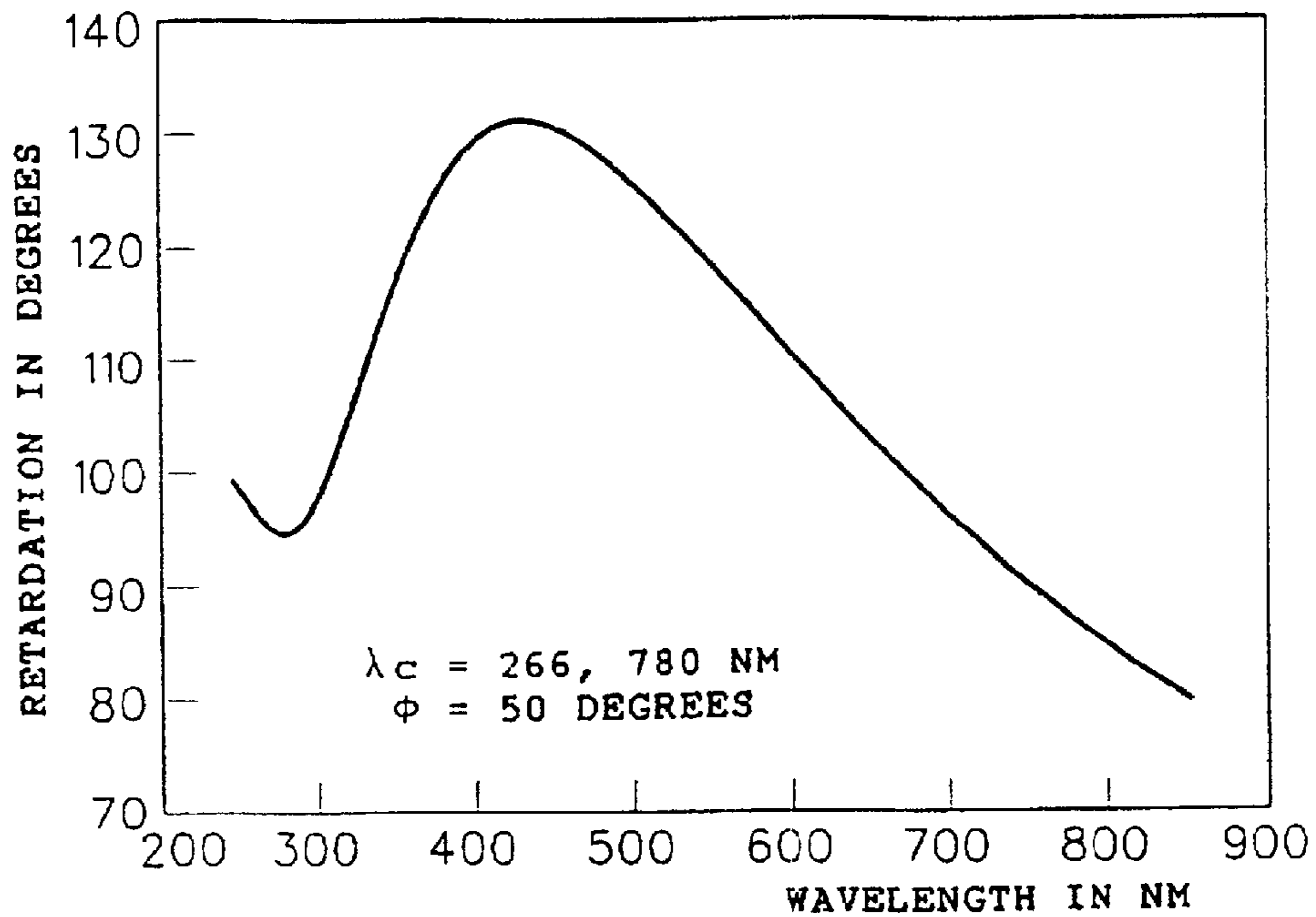
FIG. 10f
