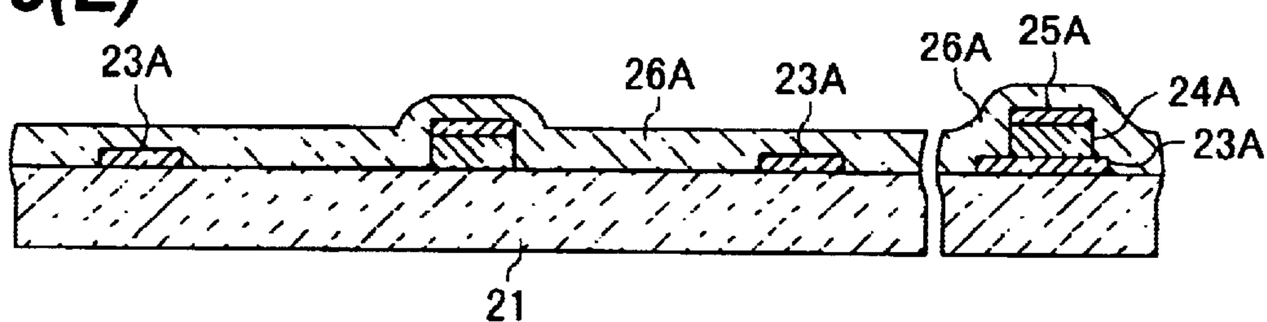
FIG.18(F)
