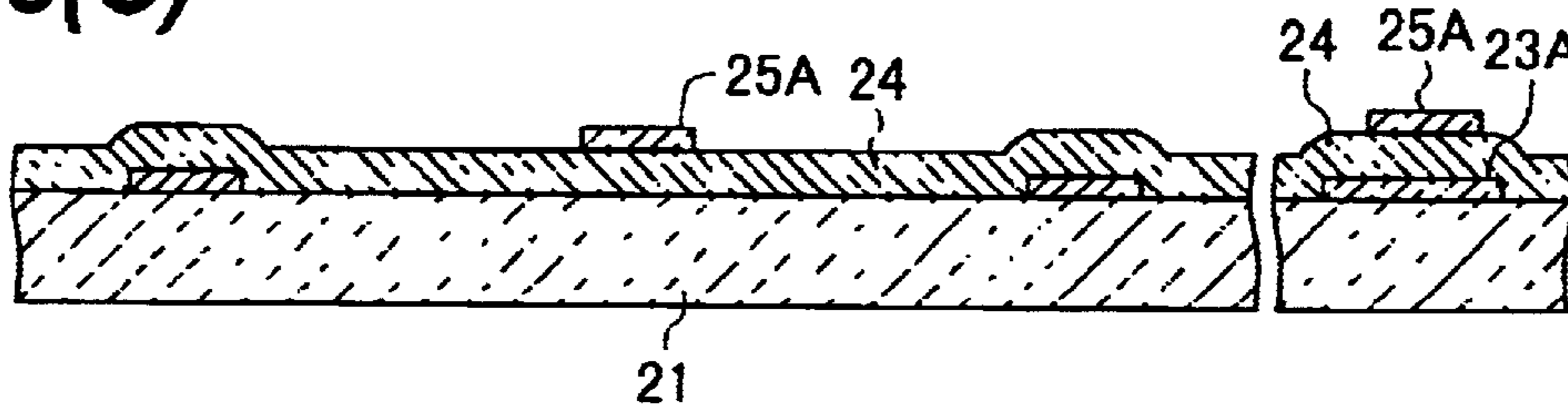
FIG.18(D)
