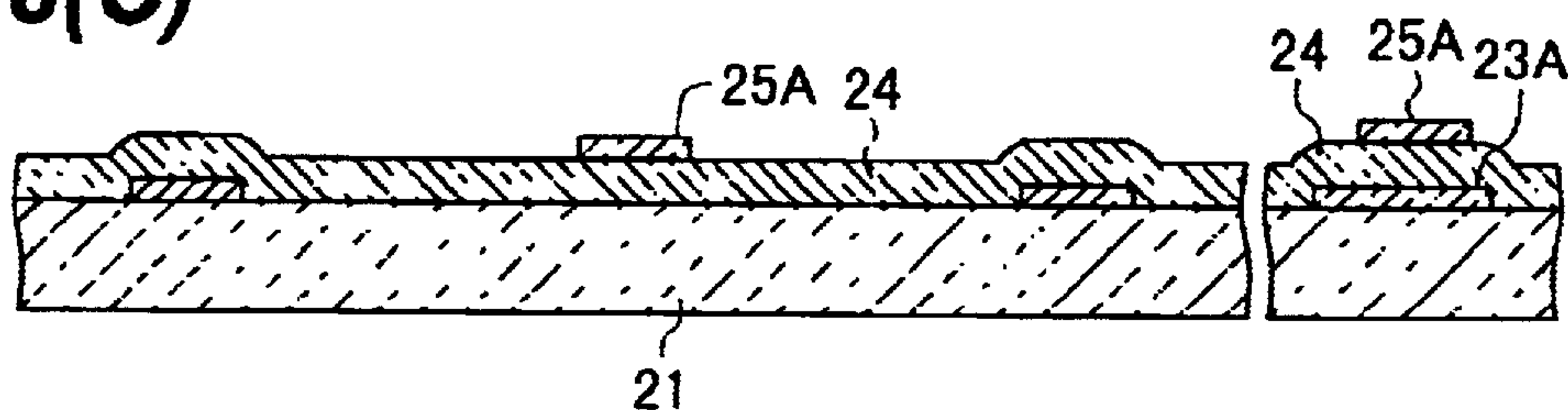
FIG.18(D)
