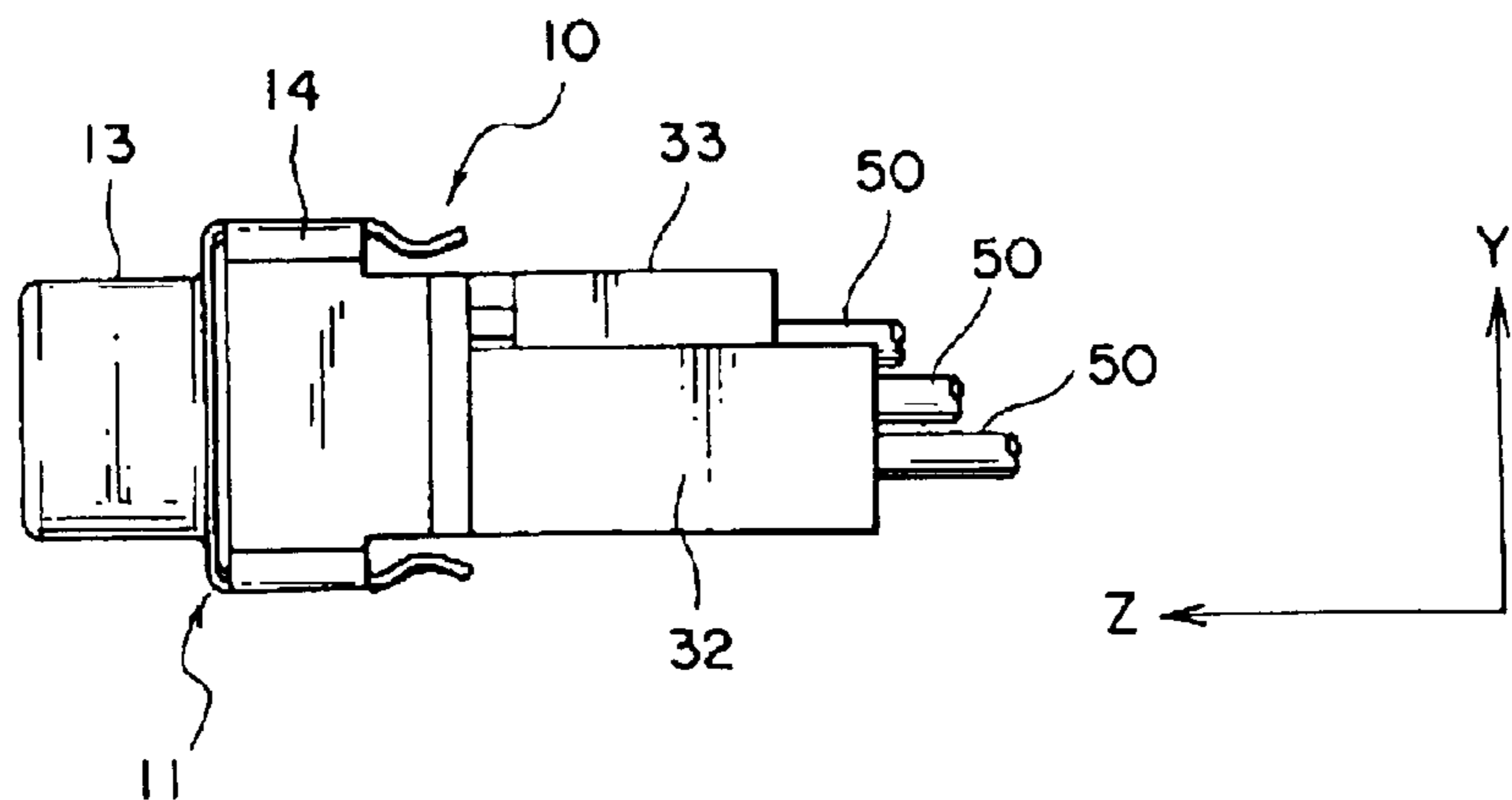
FIG. 15
