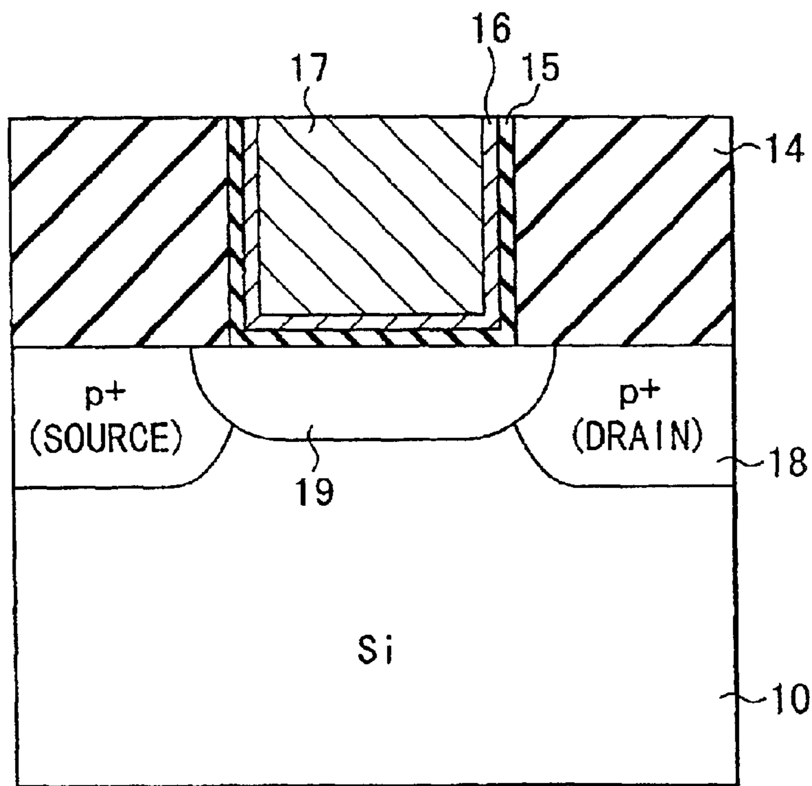
PMOS (CHANNEL: Si-Ge)
