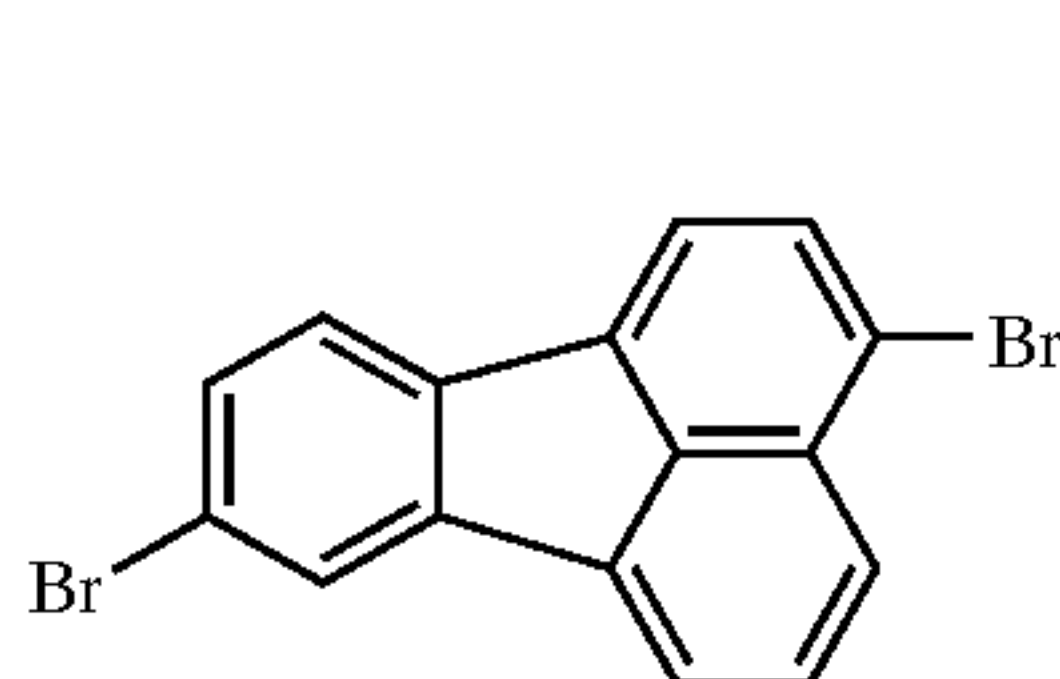
(17) 3,8-dibromo-fluoranthene
