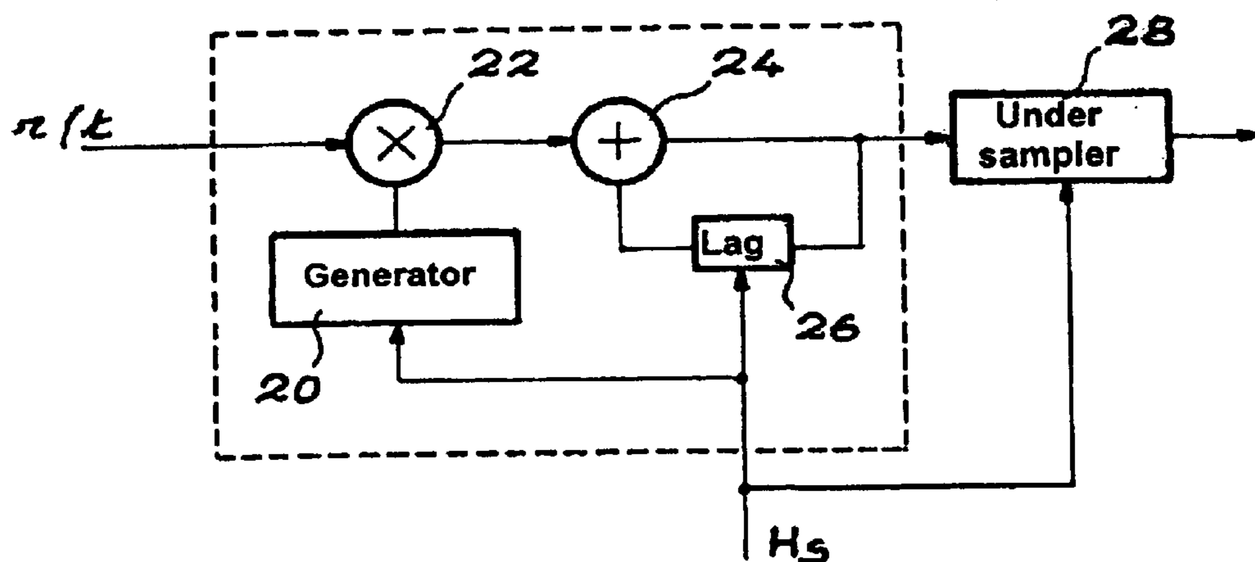
FIG. 2 -- PRIOR ART --
