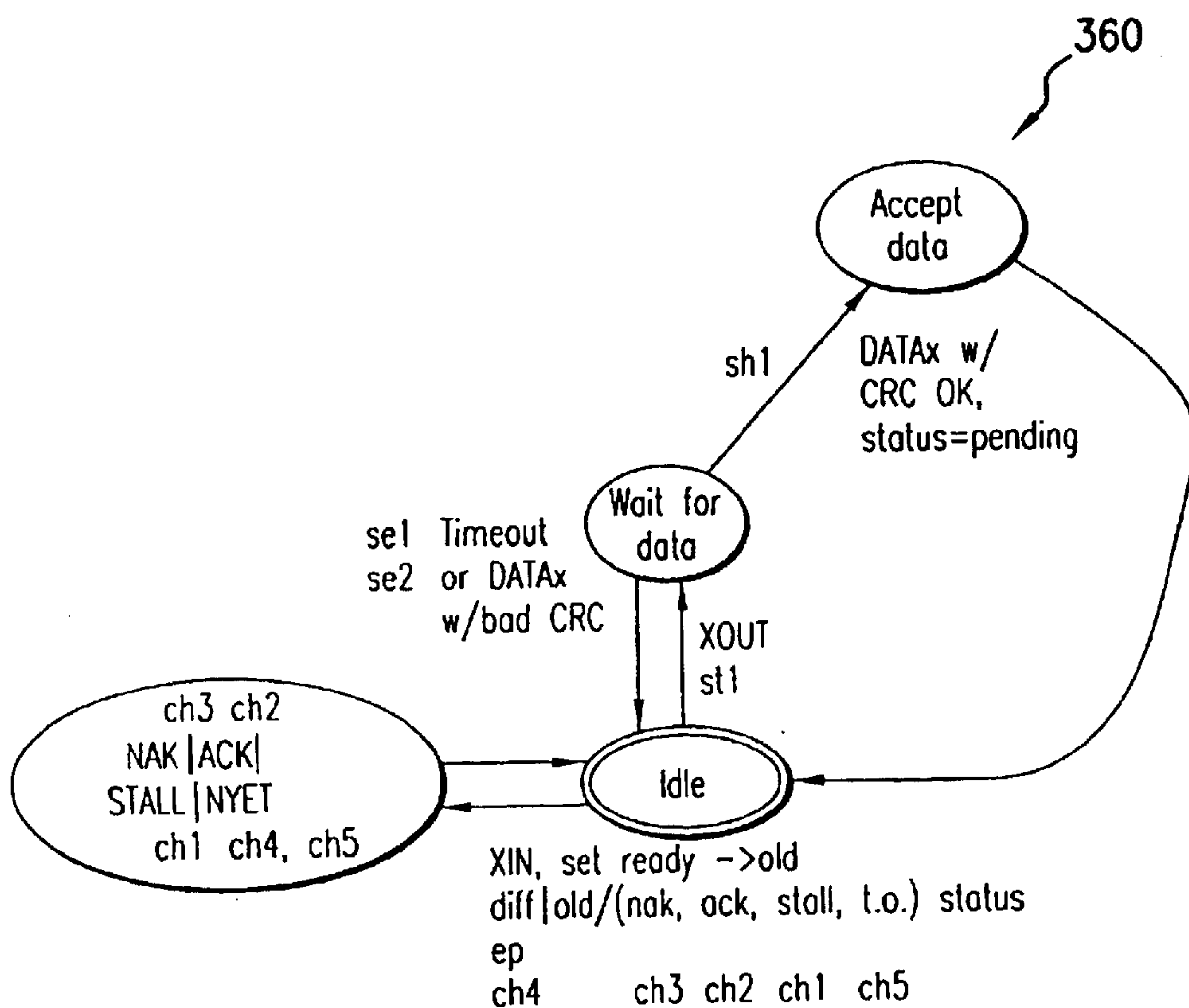
FIG. 3B
