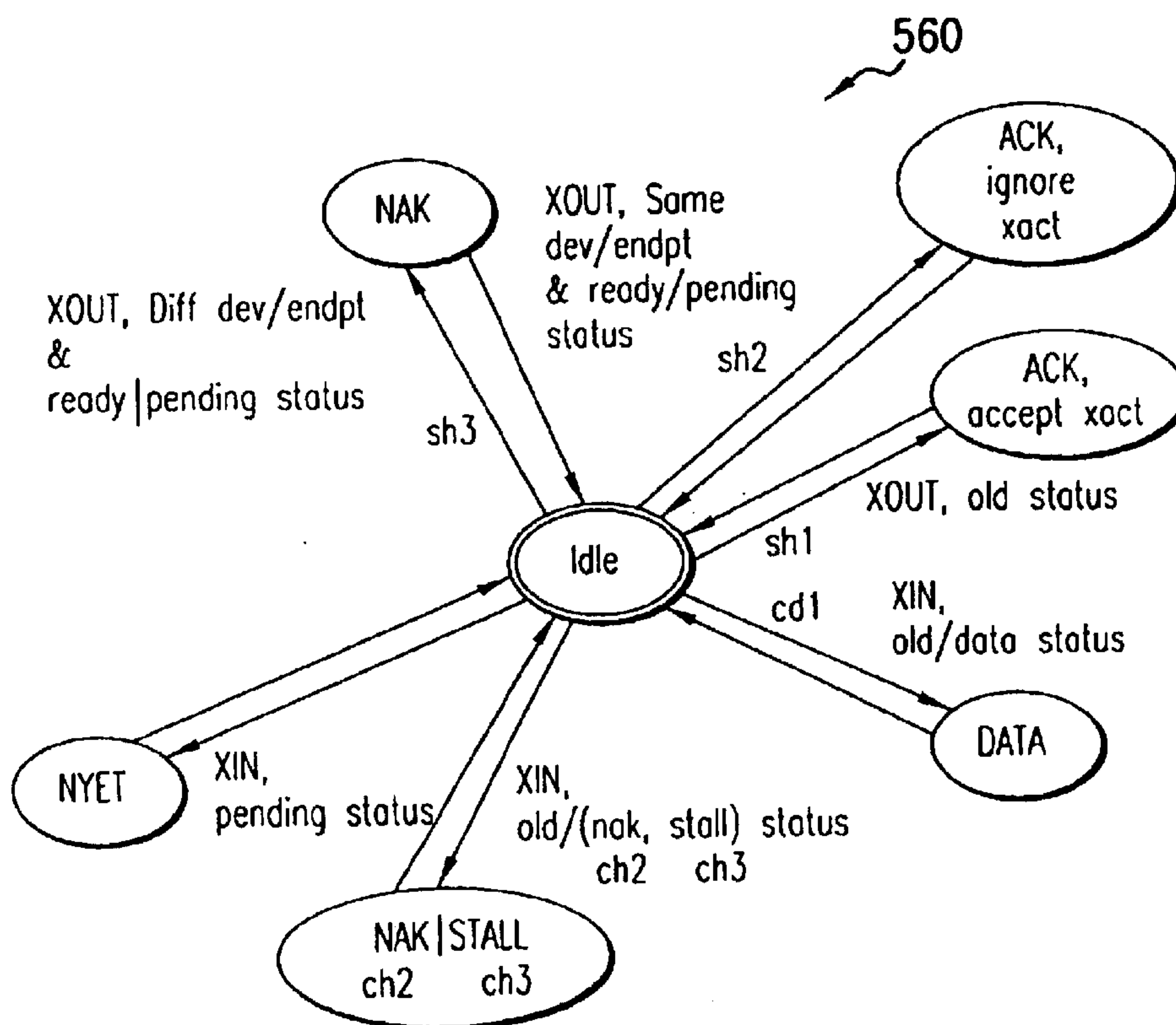
FIG.5B
