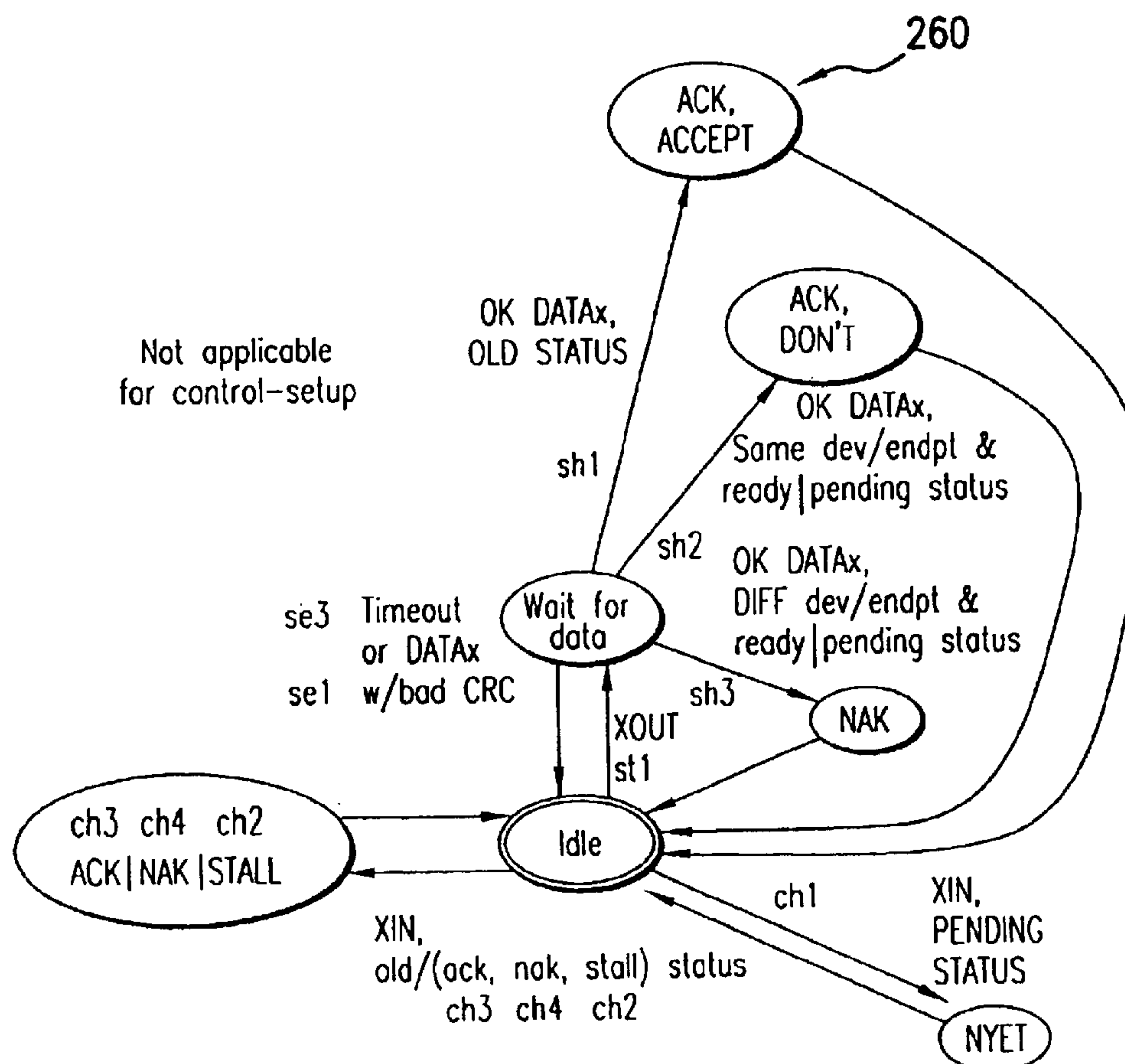
FIG. 2B
