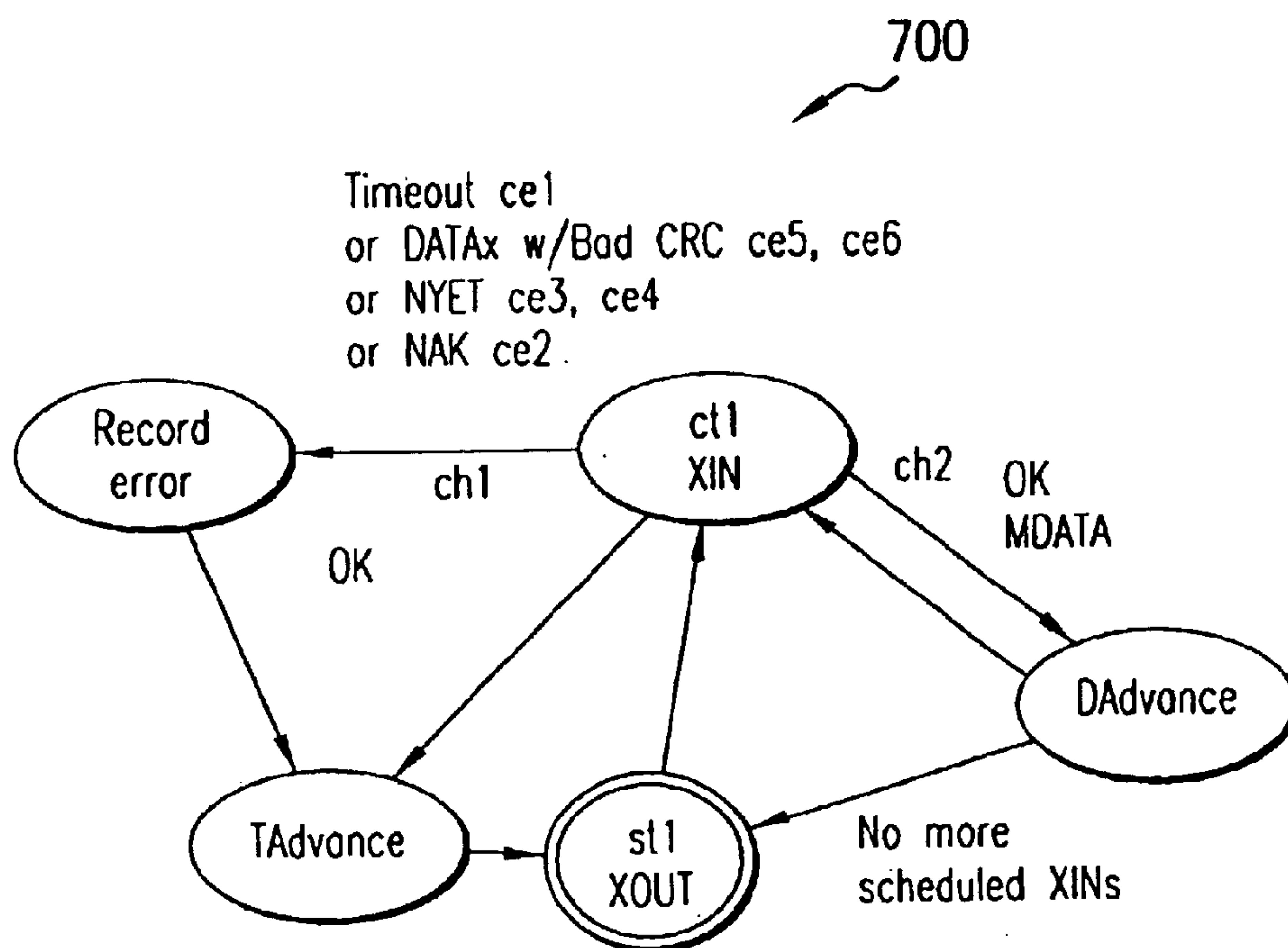
FIG.7A
