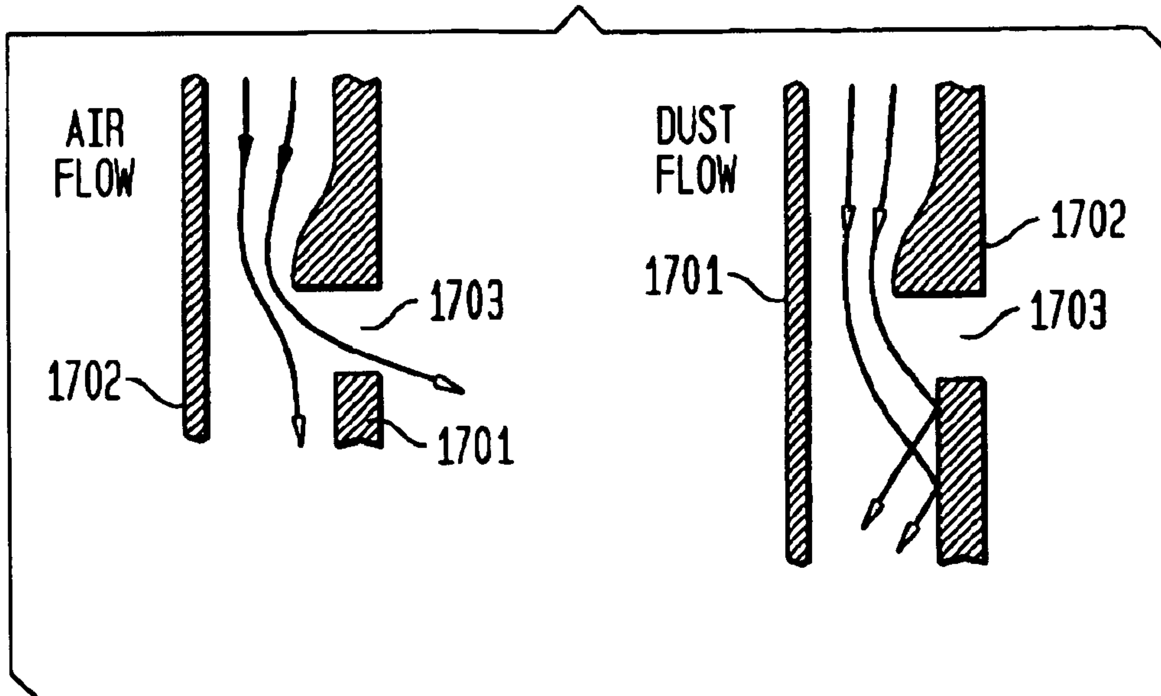
FIG. 17A
