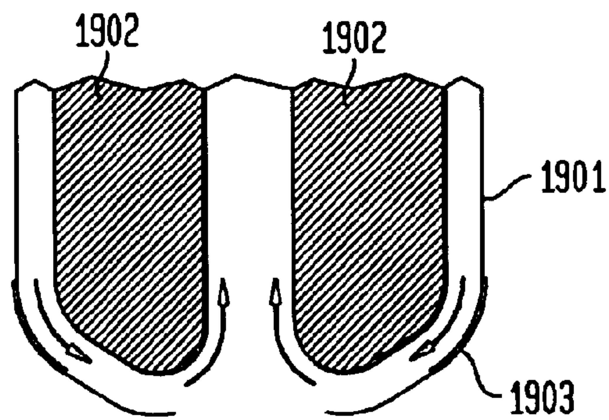
FIG. 19A
