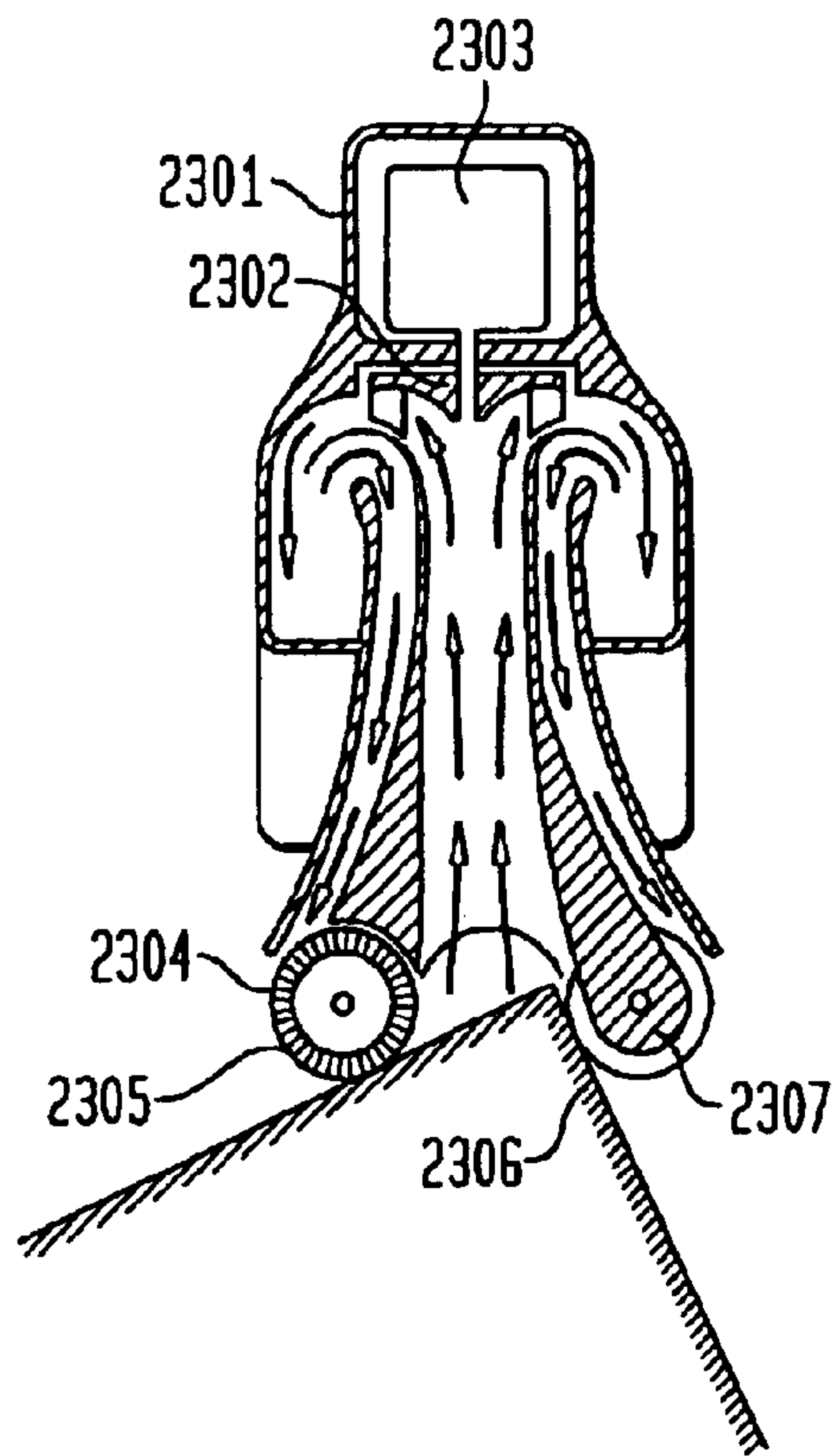
FIG. 23A
