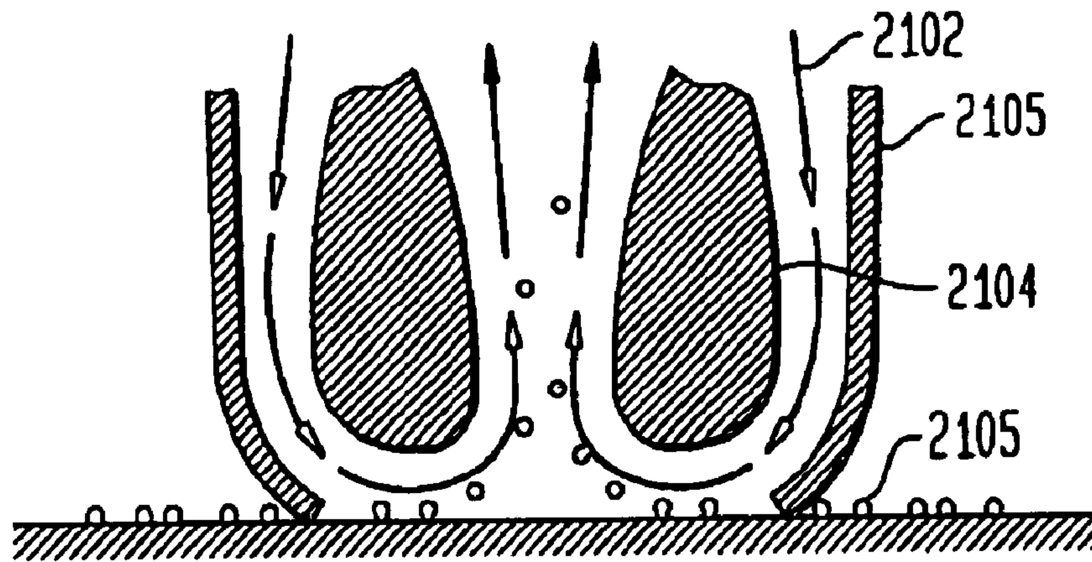
FIG. 21A
