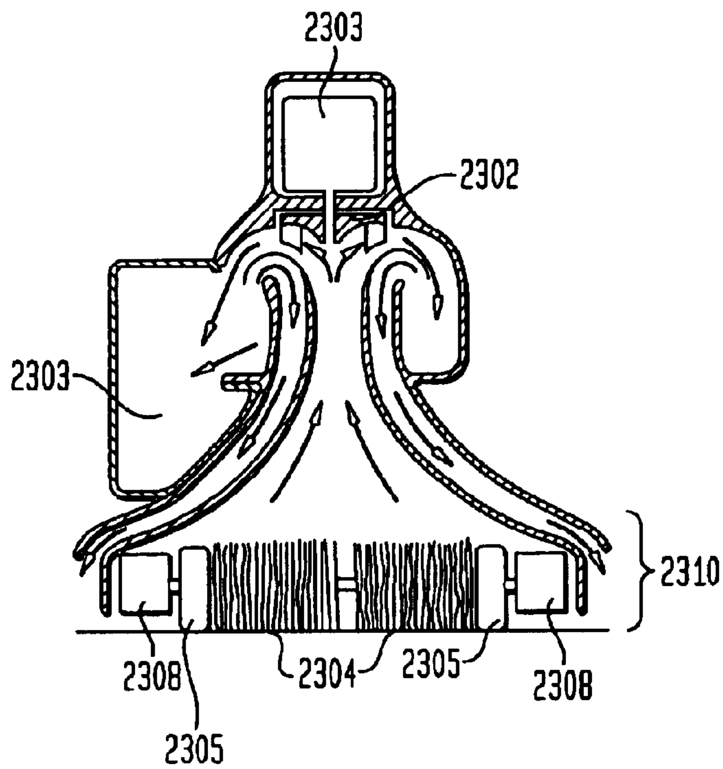
FIG. 23B
