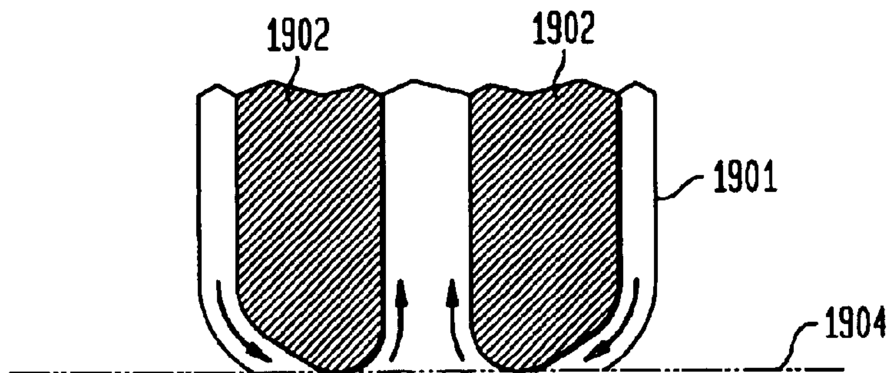
FIG. 19B
