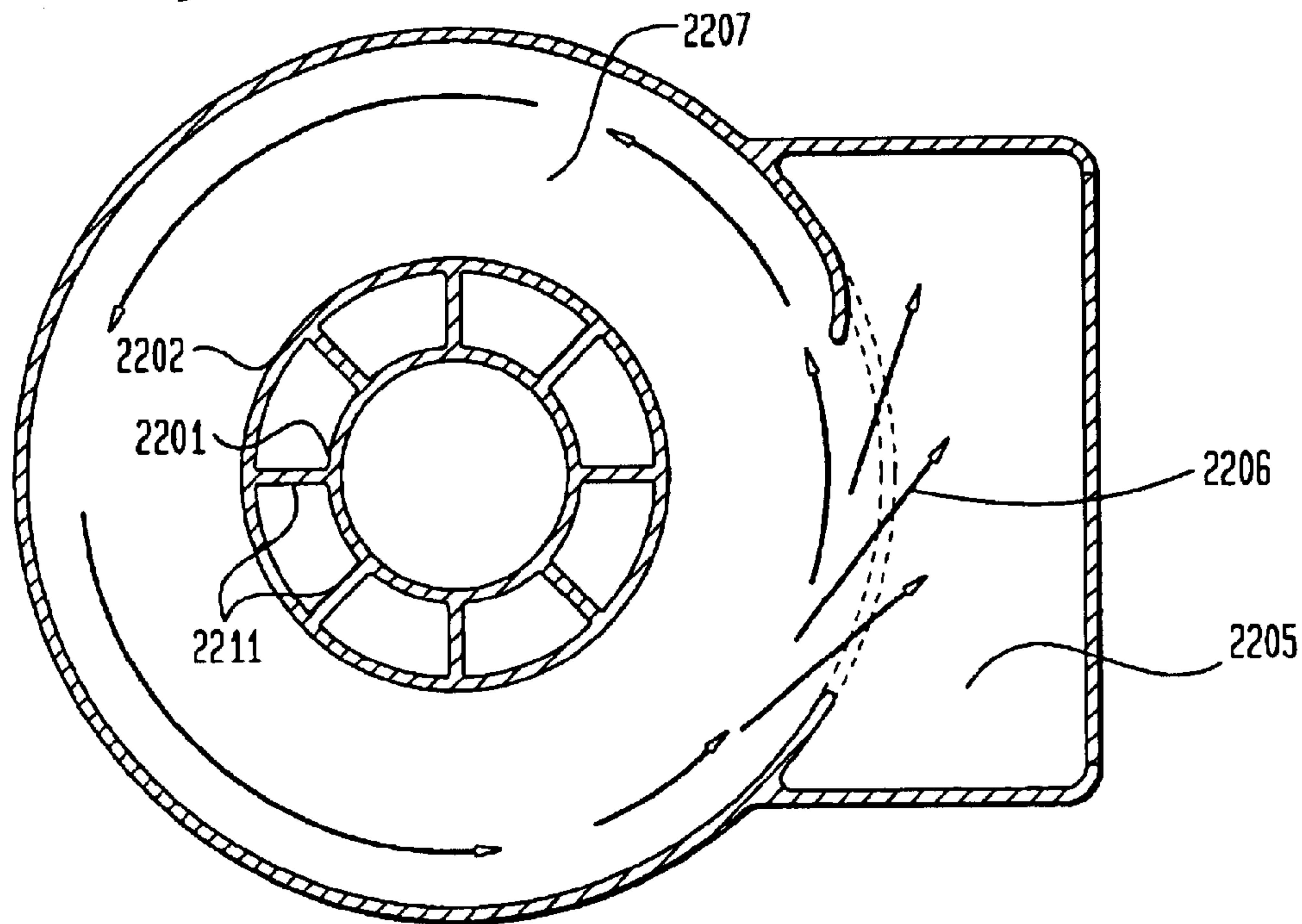
FIG. 22B
