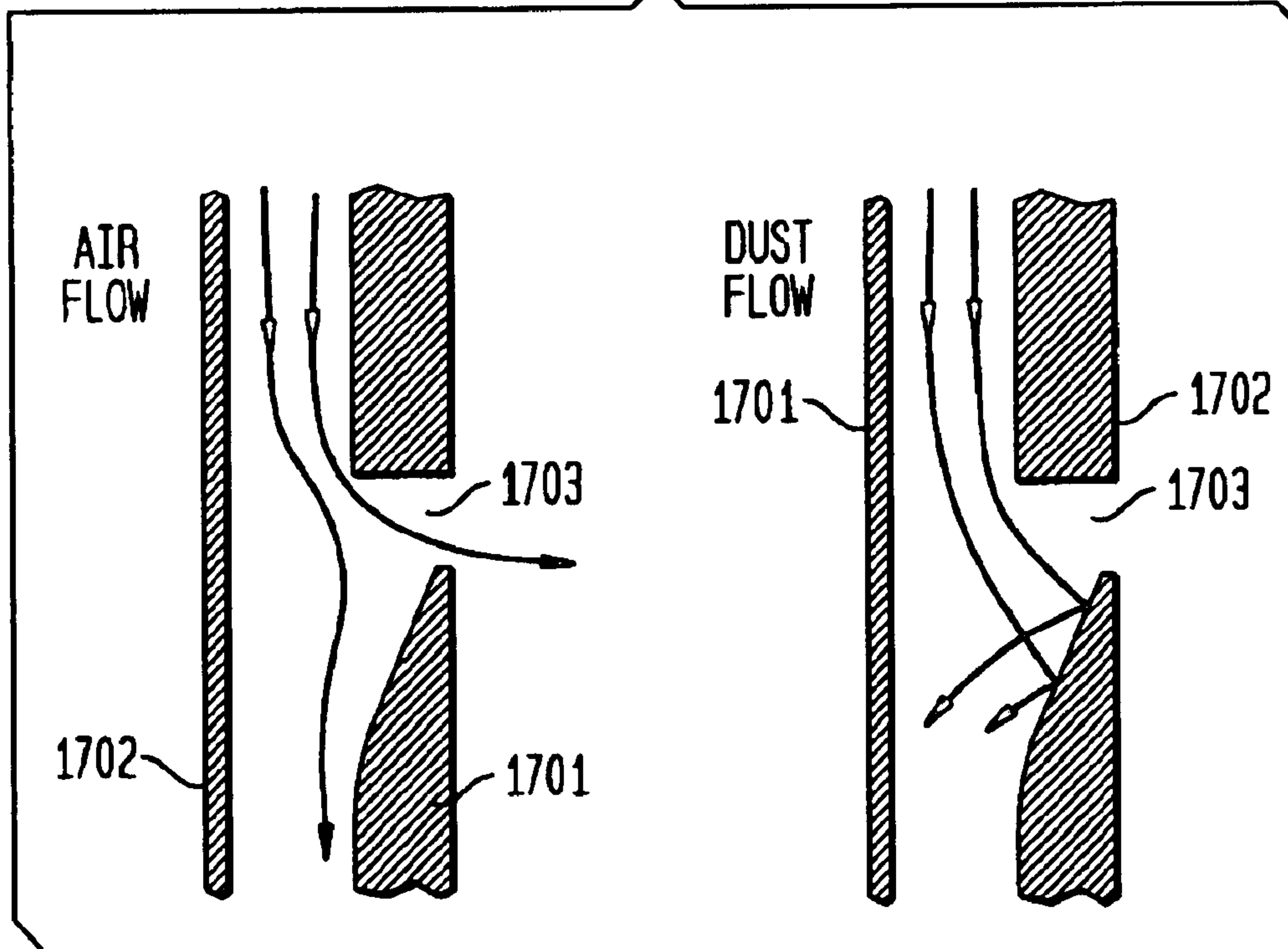
FIG. 17B
