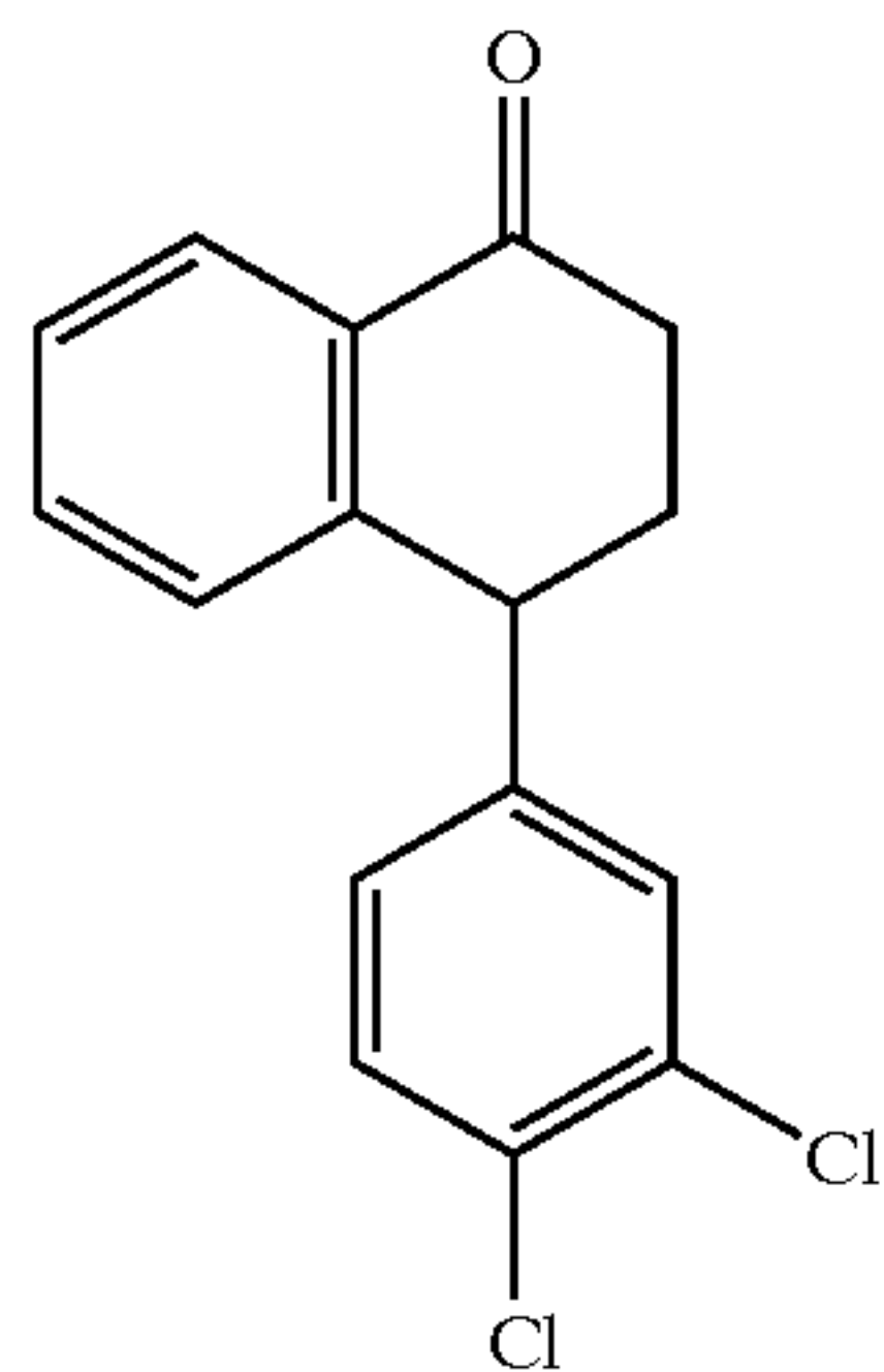
Sertralone
