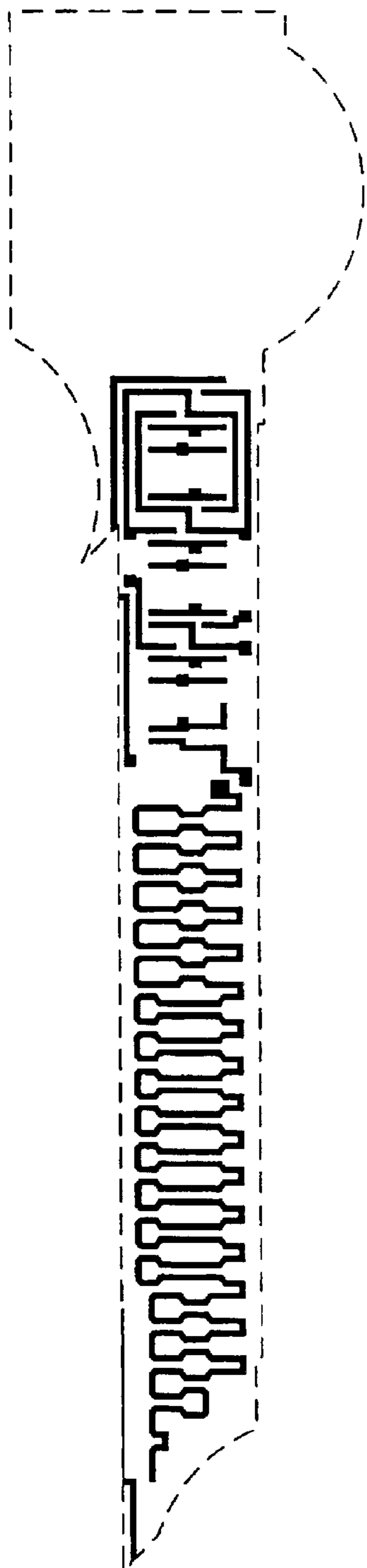
Poly mask
